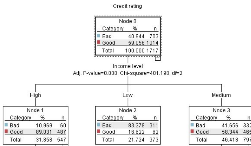
Abbildung 1. Ein einfaches Entscheidungsbaummodell
