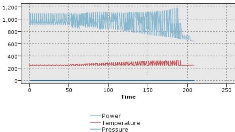
Рисунок 24. Стандартный график нескольких зависимостей, показывающий неравномерность работы силовой установки по времени (без нормализации; график для давления невиден)
