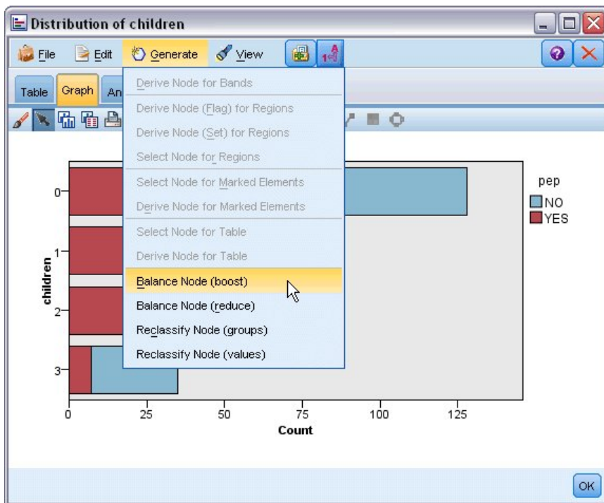
Рисунок 70. Диаграмма с выведенным меню генерирования
