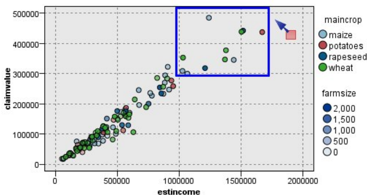
Рисунок 65. Определение региона высоких заявленных значений
