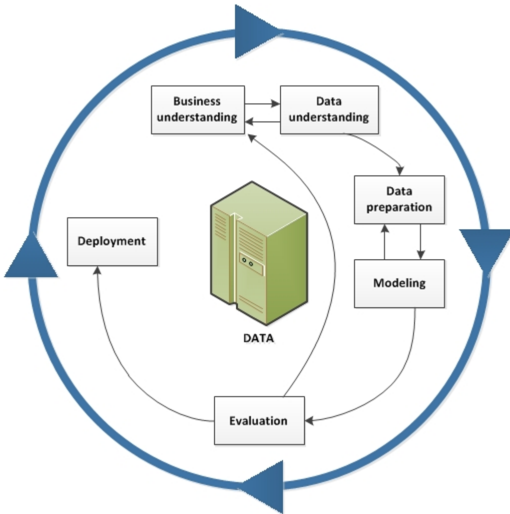
Рисунок 1. Жизненный цикл исследования данных
