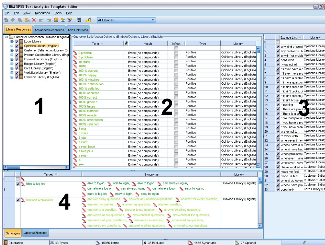
Rysunek 39. Edytor szablonów eksploracji tekstu
