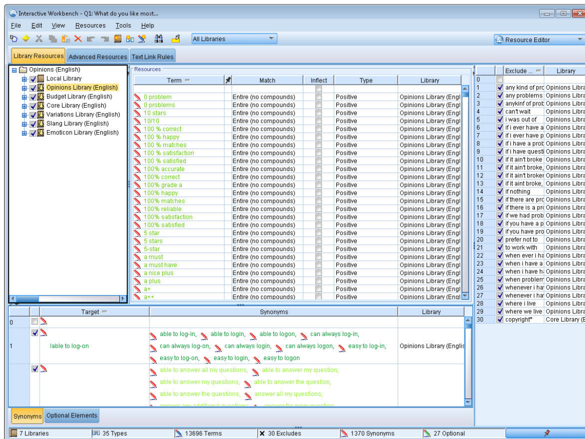
Rysunek 26. Widok Resource Editor
