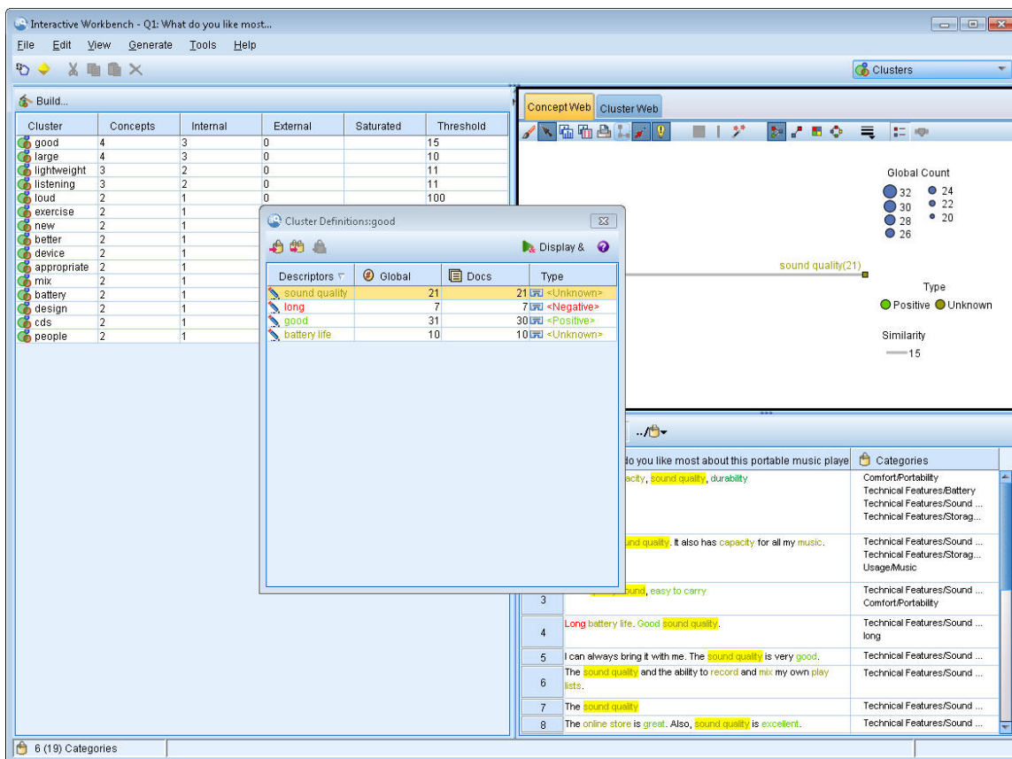
Rysunek 30. Widok Clusters
