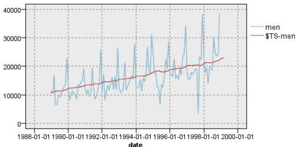
Rysunek 209. Model trendu liniowego Holta
