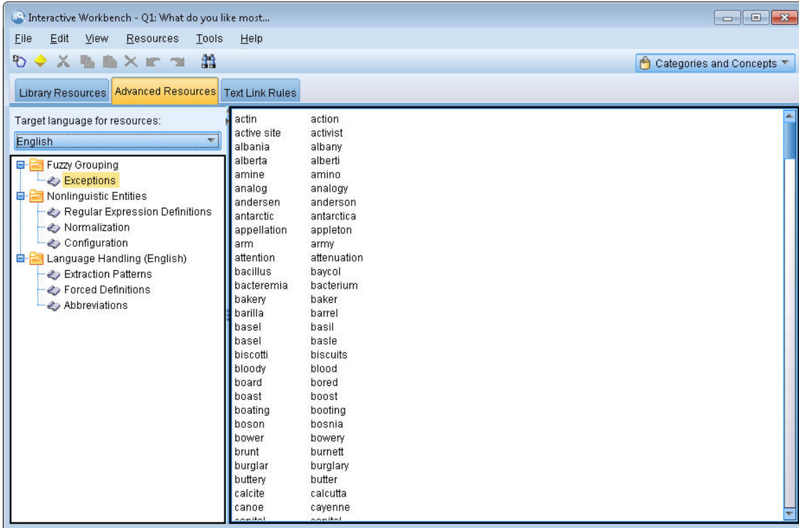
그림 40. 텍스트 마이닝 템플릿 편집기 - 고급 자원 탭
