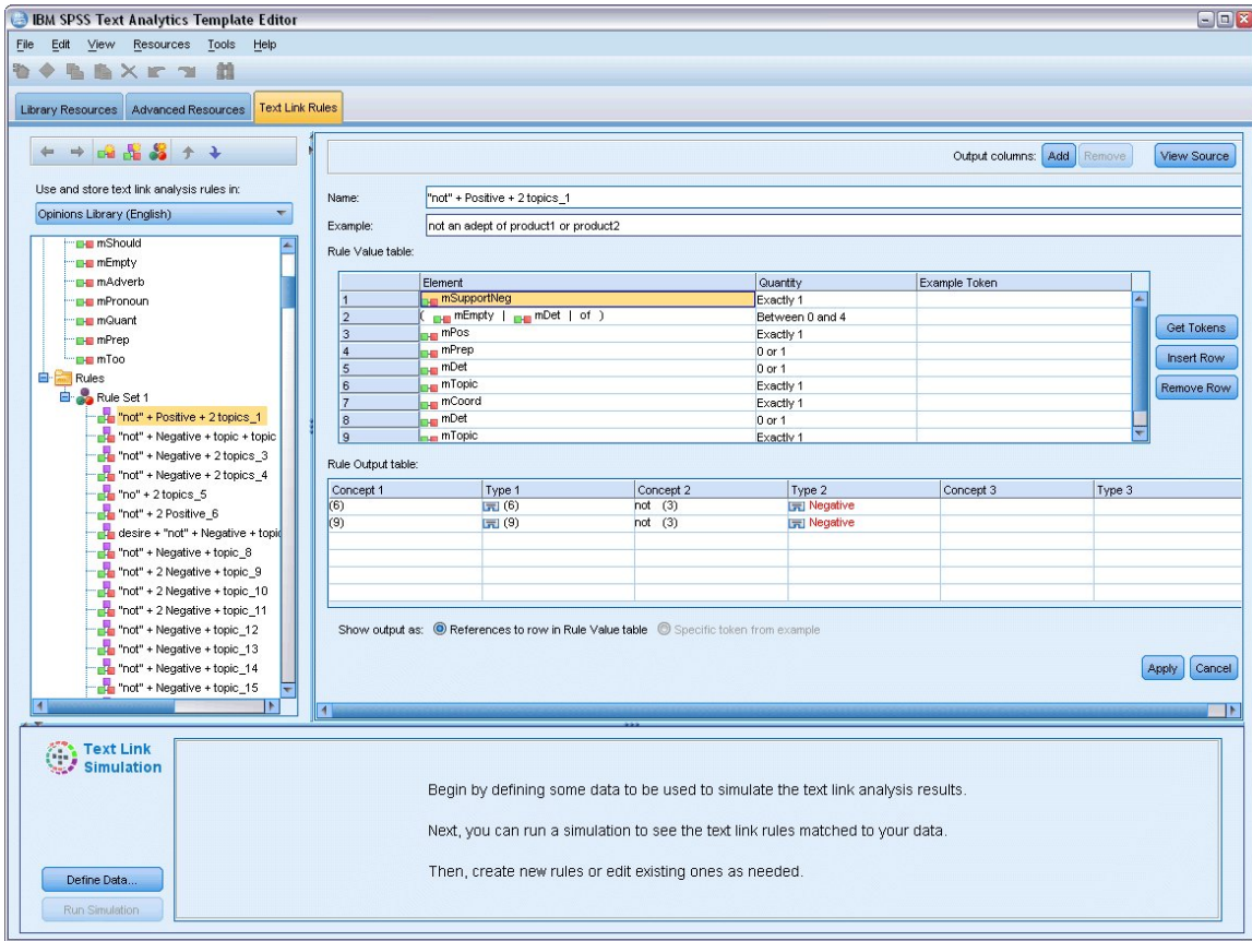
그림 44. 텍스트 링크 규칙 탭
