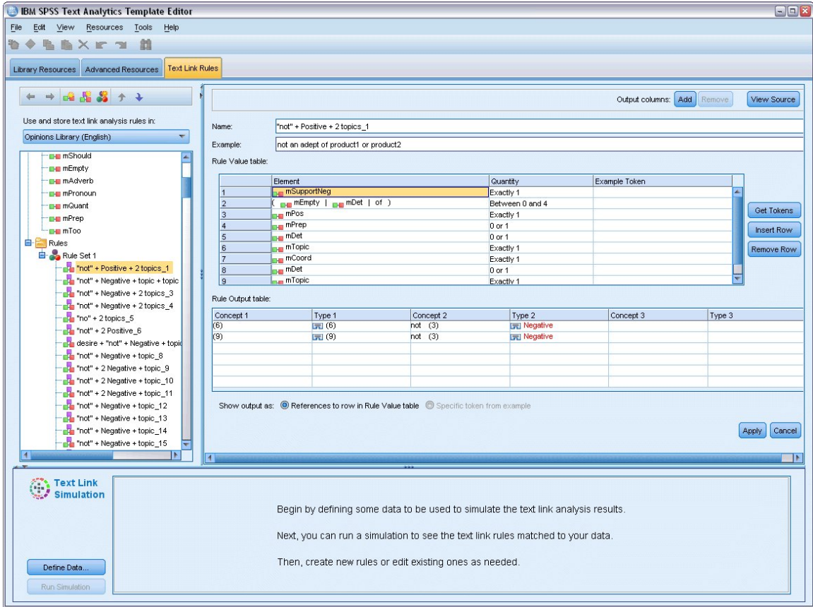
그림 41. 텍스트 마이닝 템플릿 편집기 - 텍스트 링크 규칙 탭
