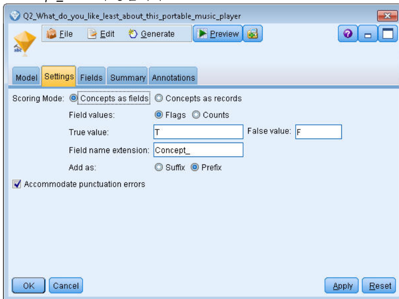
그림 6. 텍스트 마이닝 개념 모델 너깃 대화 상자: 설정 탭
