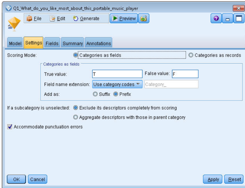
그림 12. 범주 모델 너깃 대화 상자: 설정 탭
