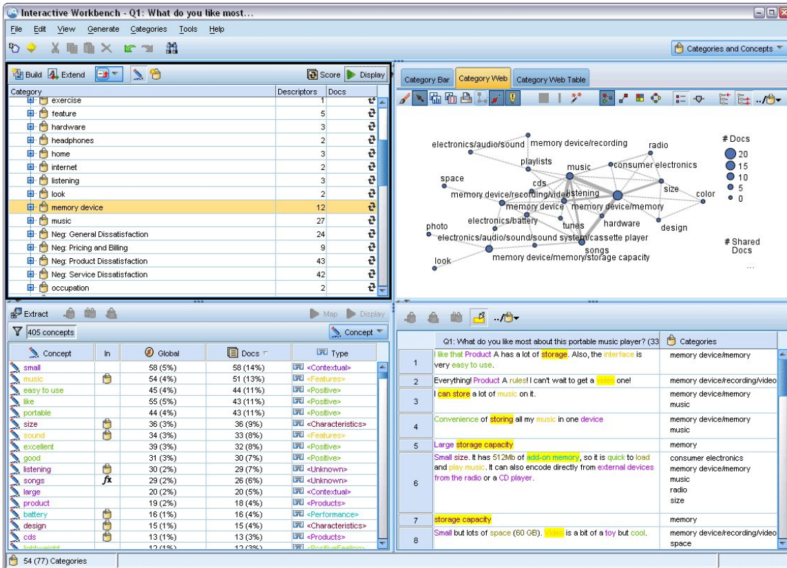
그림 23. 범주 및 개념 보기
