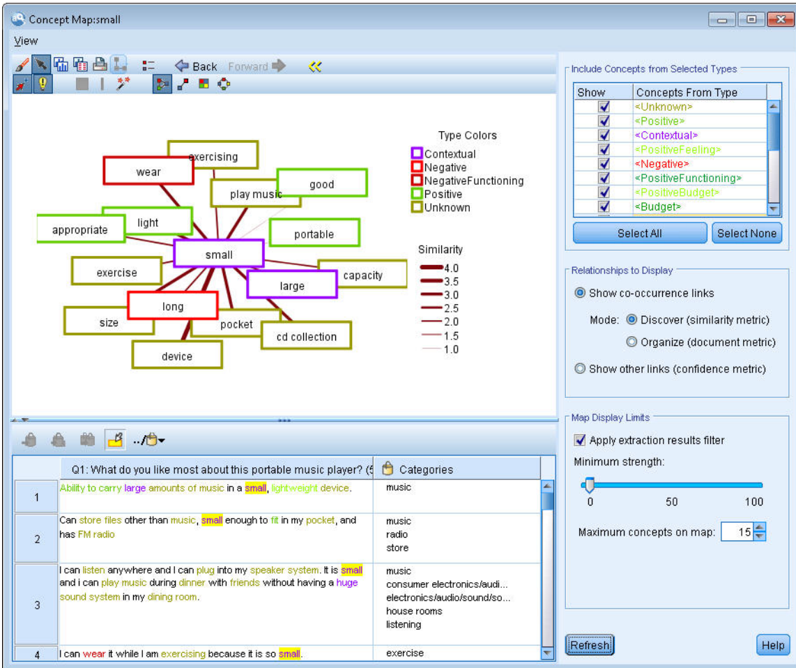
그림 27. 선택된 개념에 대한 개념 맵
