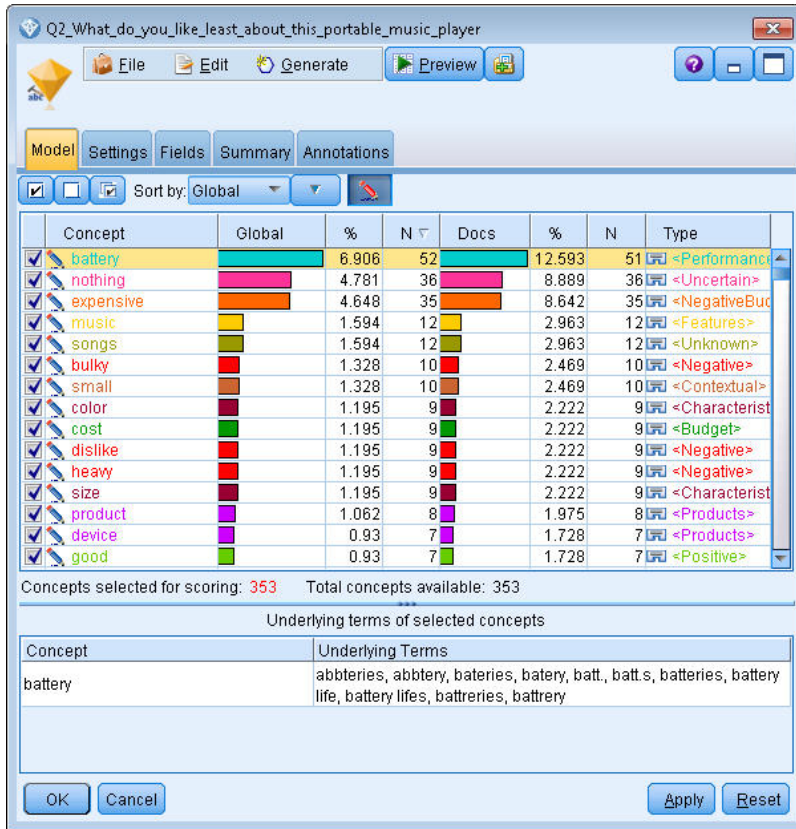
그림 5. 텍스트 마이닝 모델 너깃 대화 상자: 모델 탭
