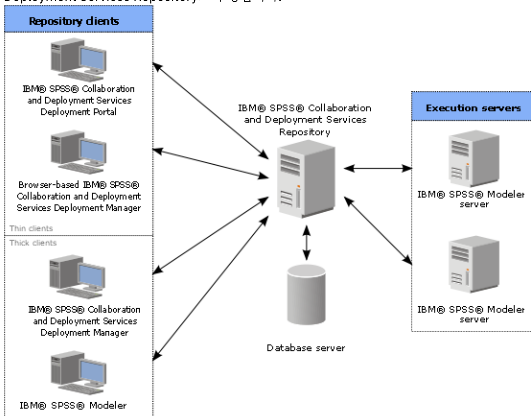
그림 1. IBM SPSS Collaboration and Deployment Services 아키텍처
