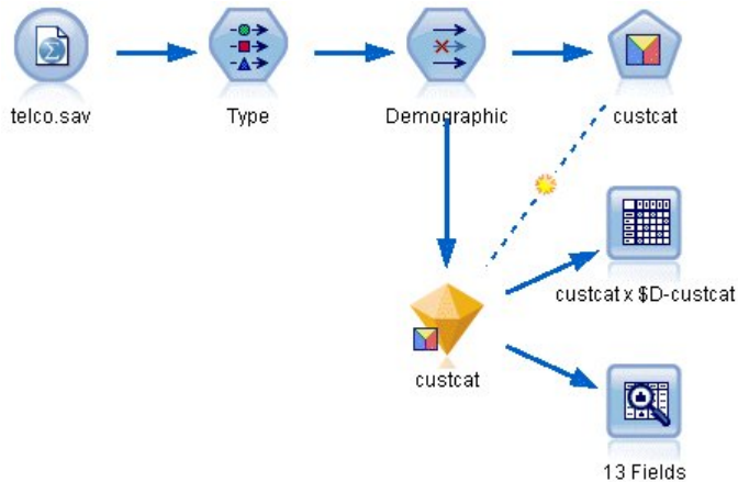
図 266. 判別分析を使用して顧客を分類するためのサンプル・ストリーム
