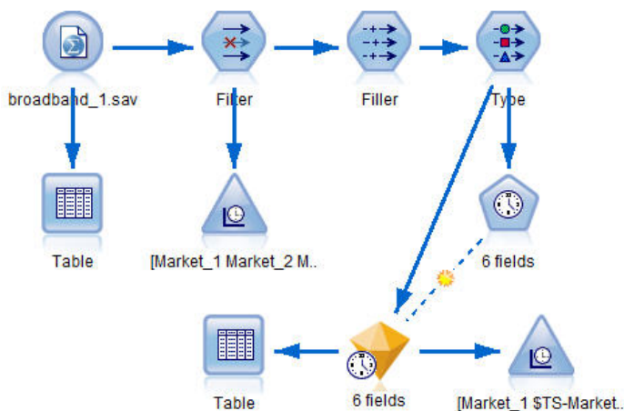
図 170. 時系列モデル作成を示すサンプル・ストリーム
