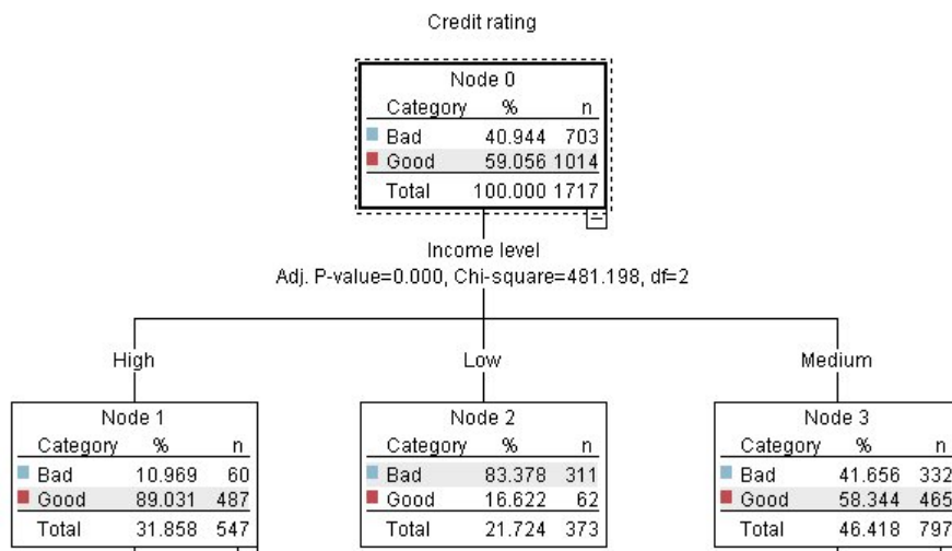
図 11. 簡単なディジジョン ツリー モデル
