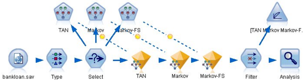
図 230. ベイズ・ネットワークのサンプル・ストリーム
