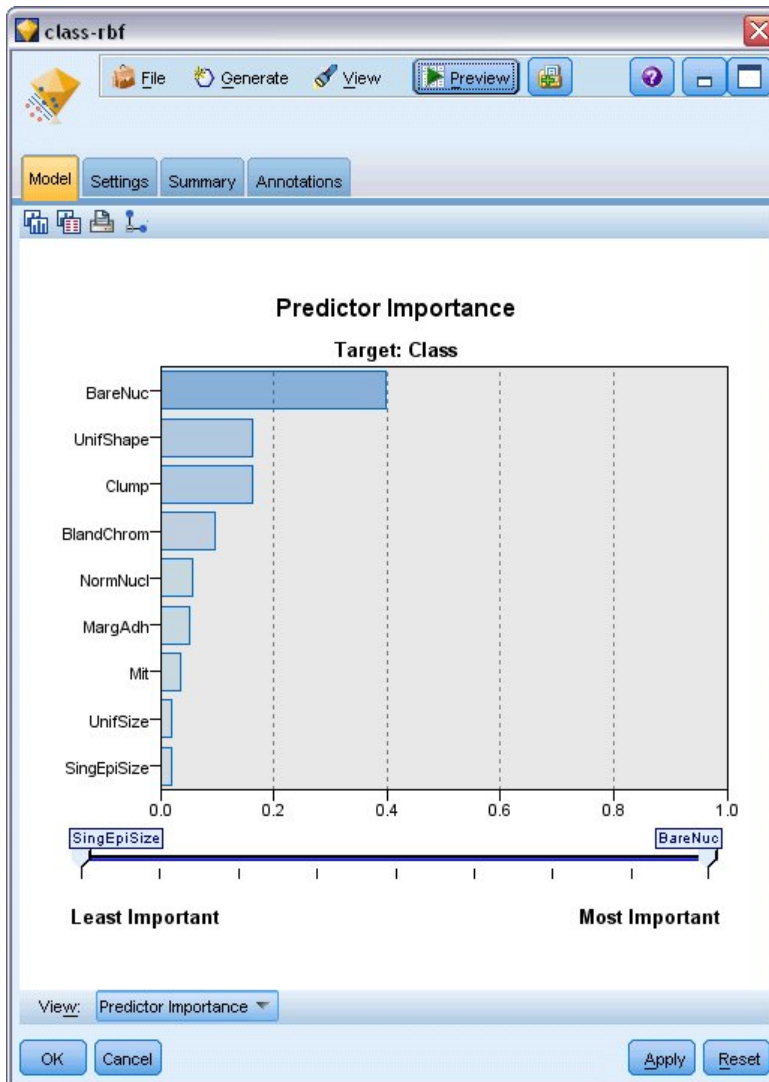
図 333. 予測重要度グラフ
