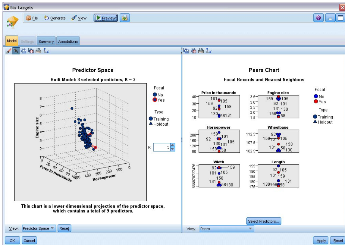
図 391. モデル・ビューアー・ウィンドウ
