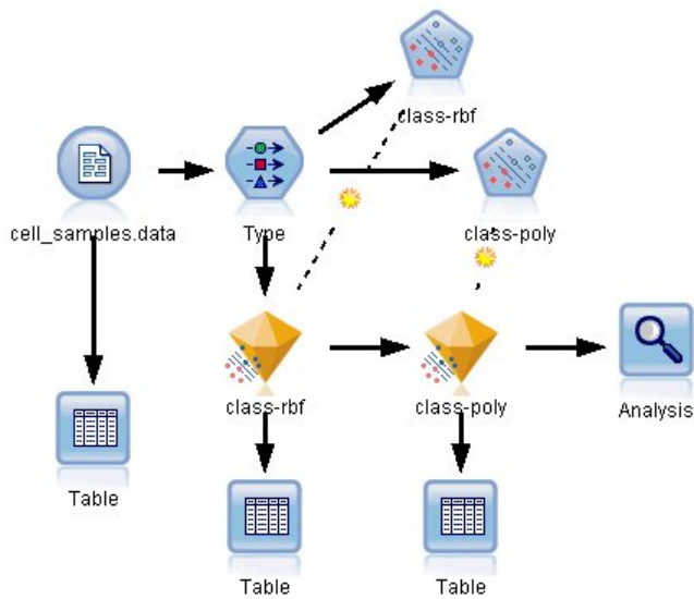
図 327. SVM モデル作成を表示するサンプル・ストリーム
