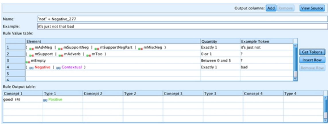
图 35. TLA 规则
