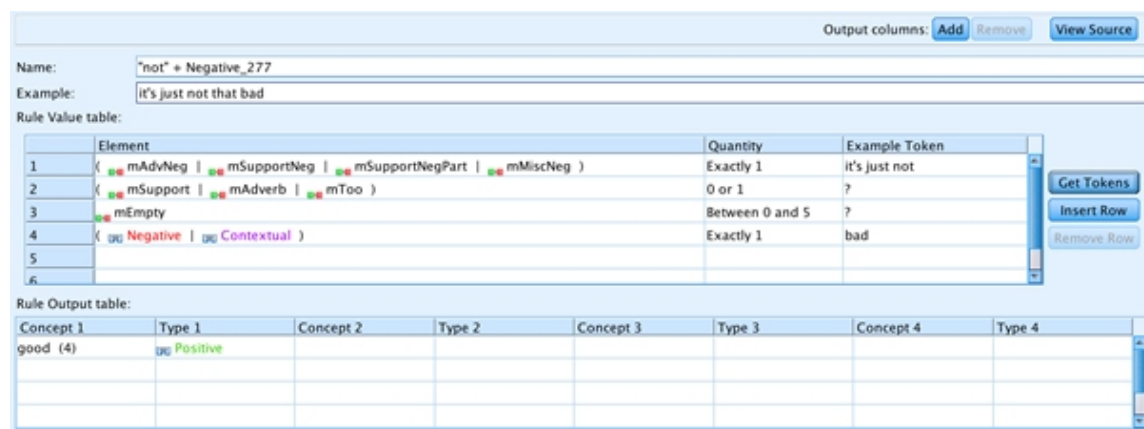
Рисунок 35. Правила TLA
