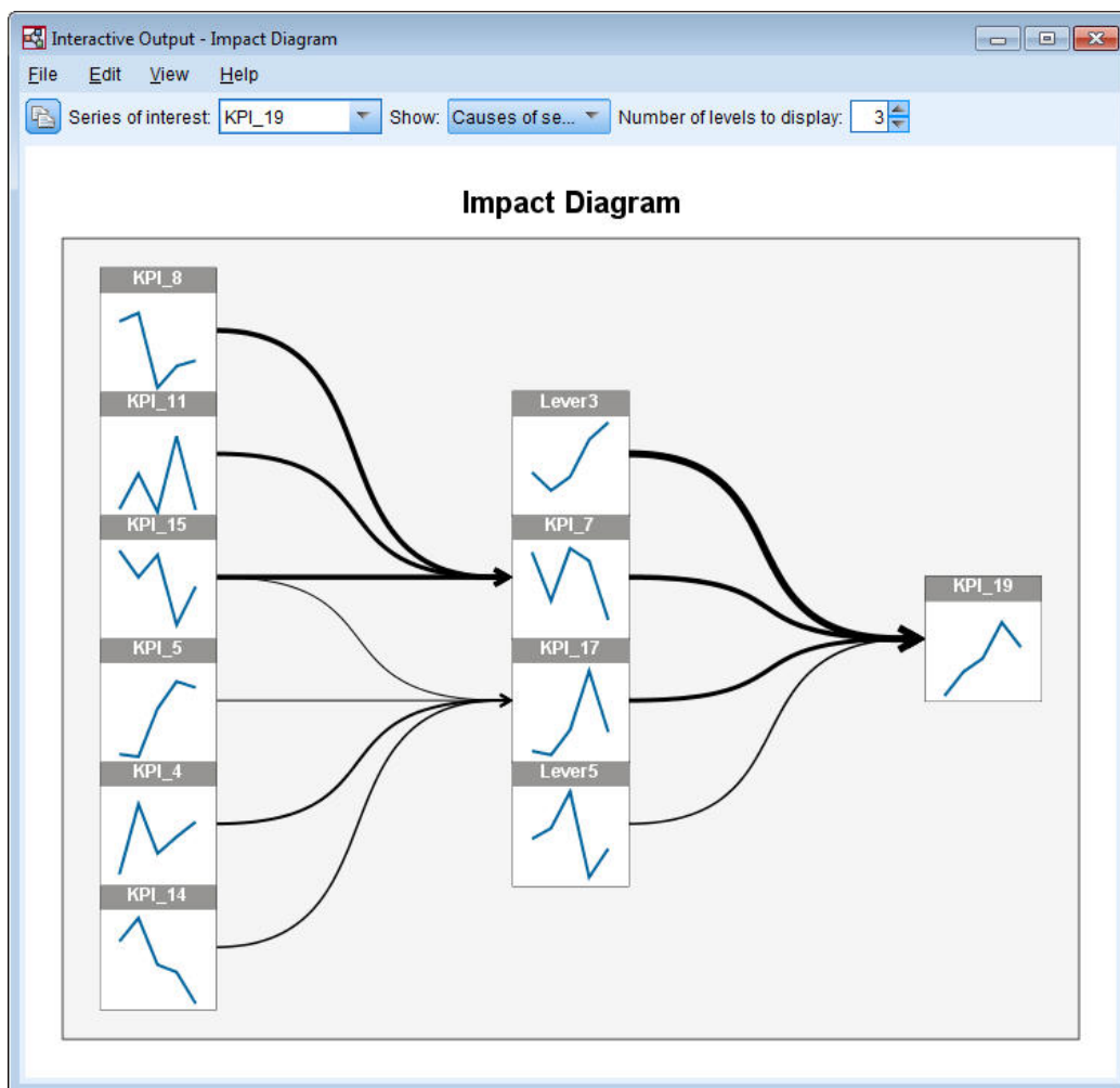
Rysunek 405. Diagram wpływu przyczyn
