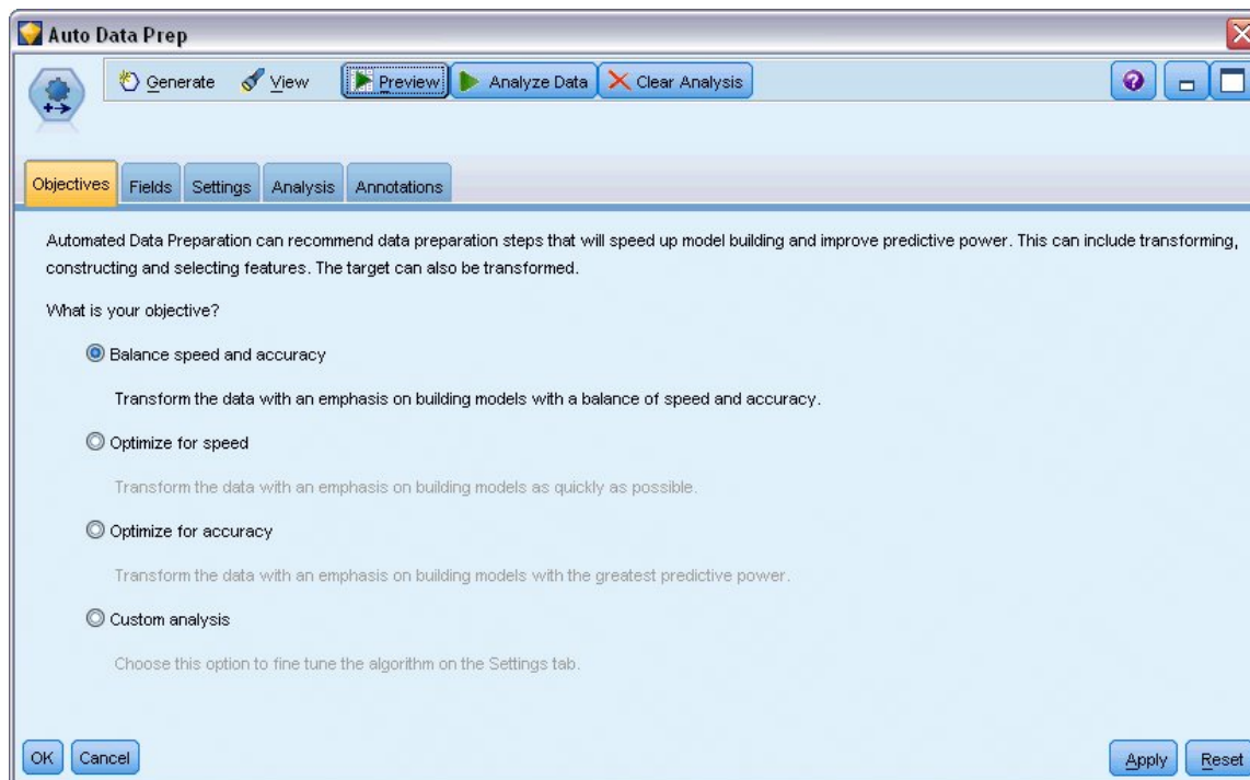
Rysunek 53. Domyślne cele ADP
