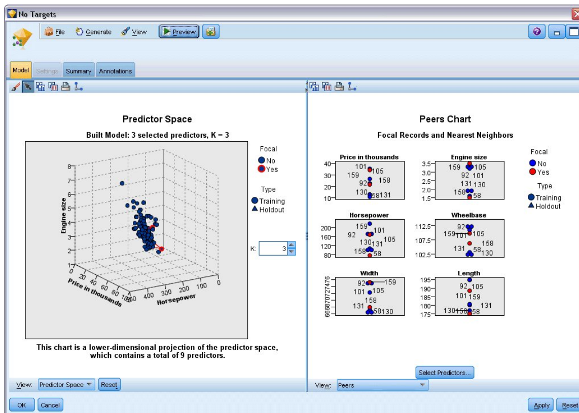
Rysunek 391. Okno Przegląd modelu
