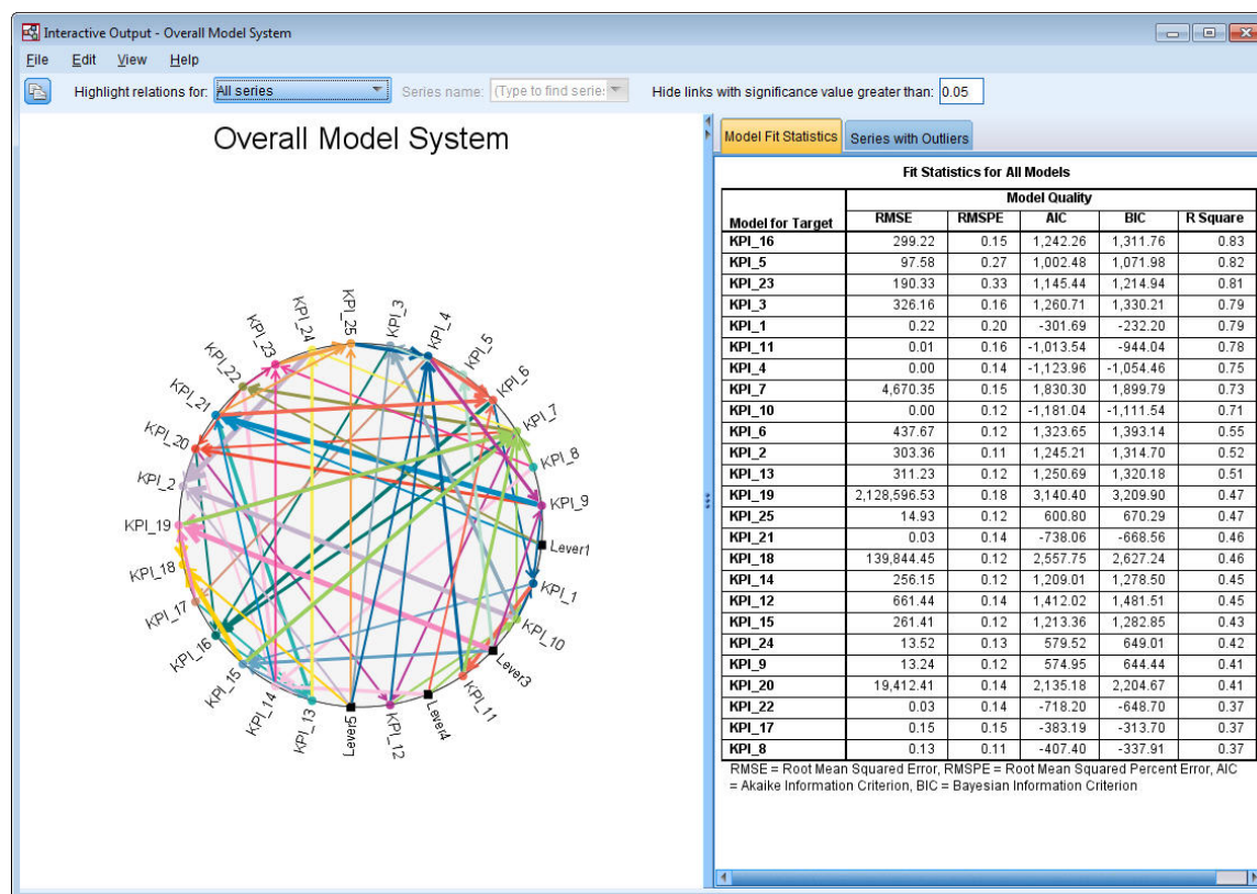
Rysunek 401. Ogólny system modelu, widok dla wszystkich szeregów
