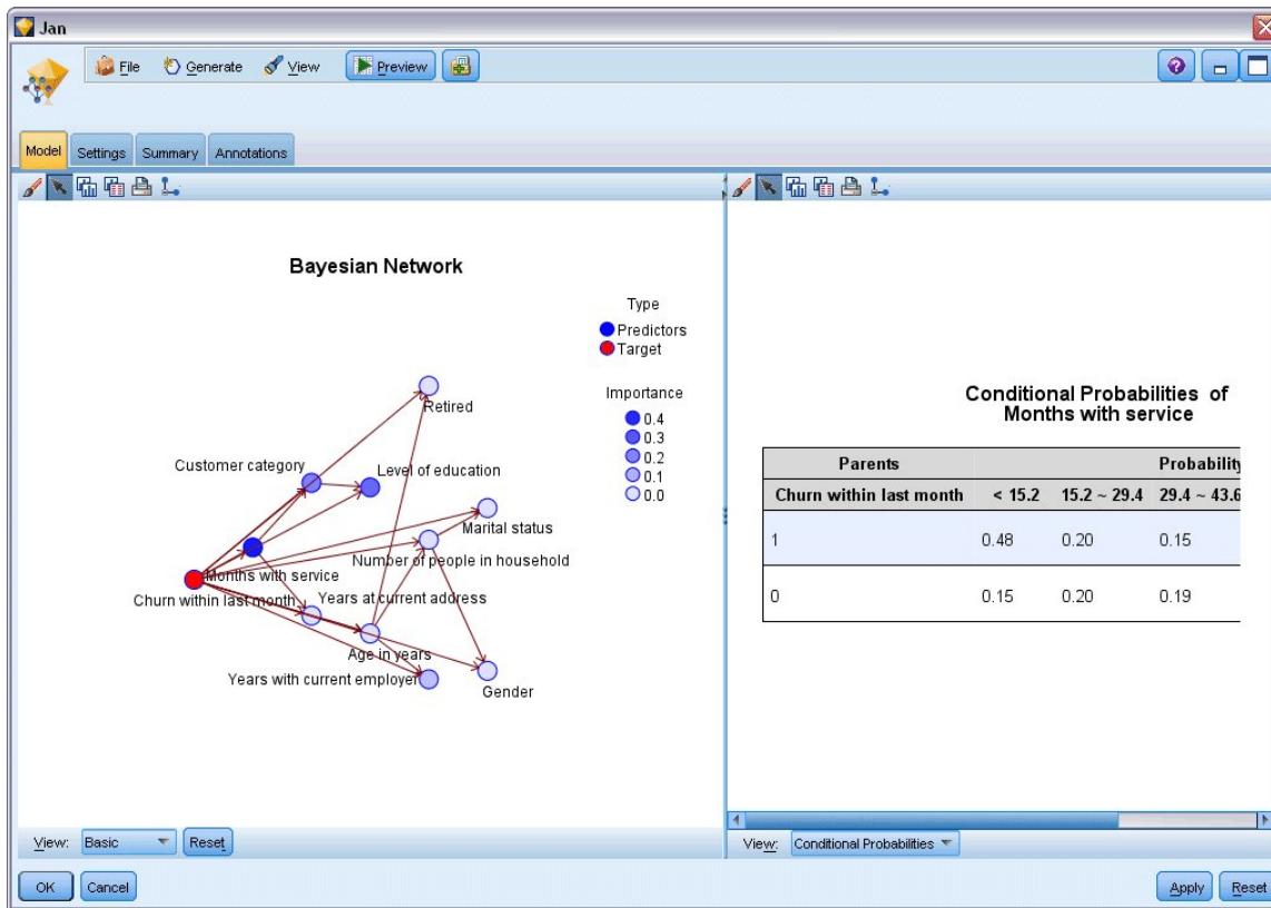
Rysunek 251. Model Sieć Bayesa przedstawiający prawdopodobieństwa warunkowe
