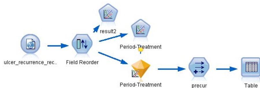
Rysunek 295. Przykładowy strumień pozwalający przewidzieć nawroty wrzodów
