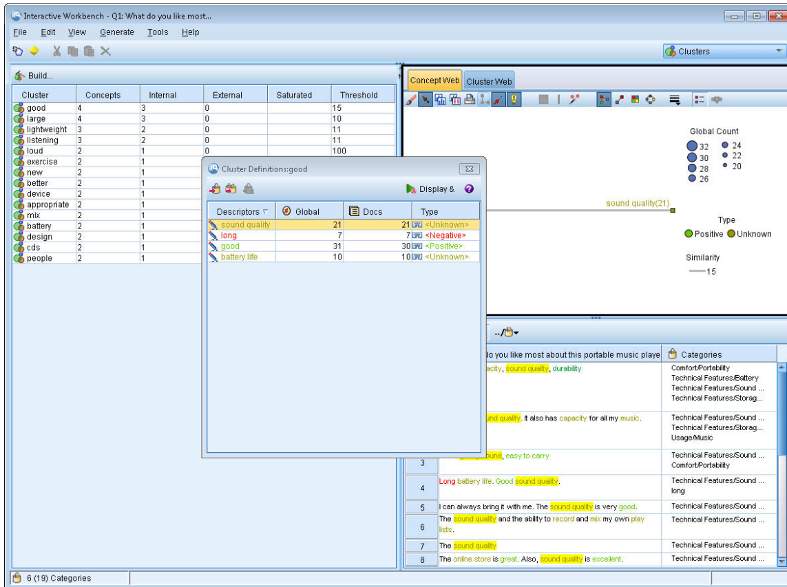
그림 24. 군집 보기
