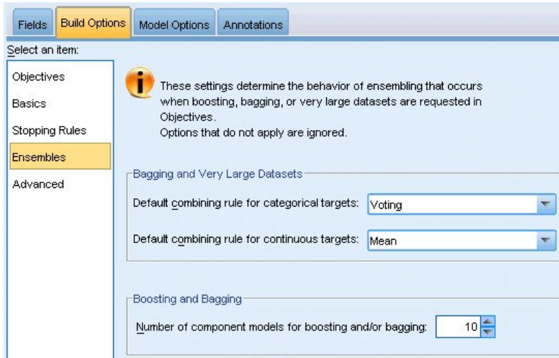
그림 35. 앙상블 설정
