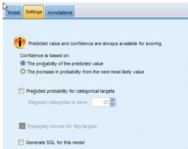
그림 43. 설정 탭
