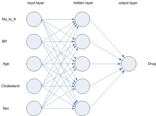
그림 31. 신경망의 구조
