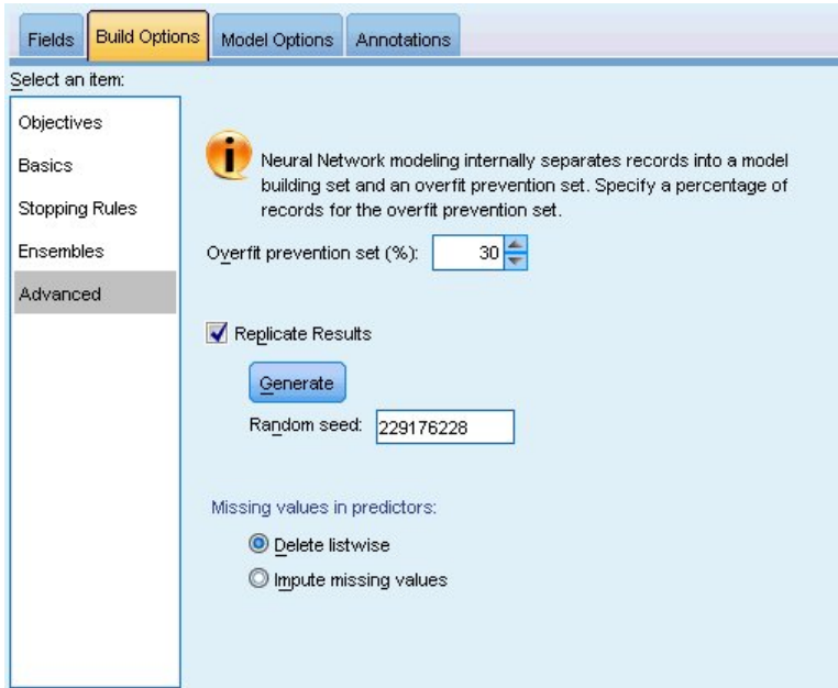
그림 36. 고급 설정
