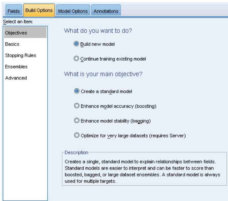
그림 32. 목적 설정
