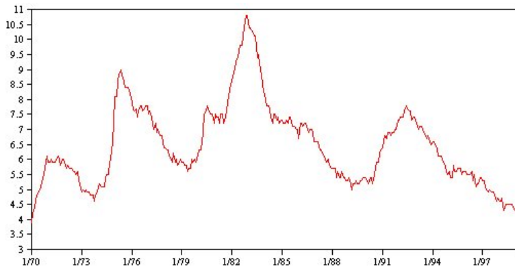
그림 55. 비계절 순환
