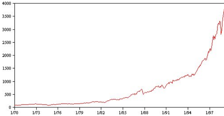
그림 53. 추세
