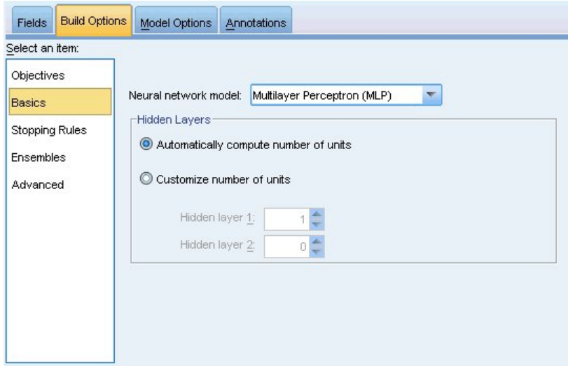
그림 33. 기본 설정
