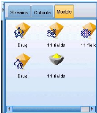
그림 26. 모델 팔레트
