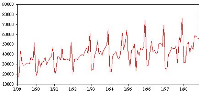
그림 54. 계절 순환
