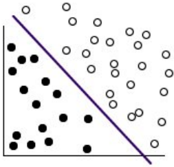
그림 61. 변환 데이터
