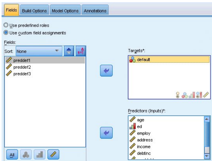
그림 30. 필드 탭
