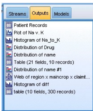
Abbildung 6. Registerkarte "Ausgaben"
