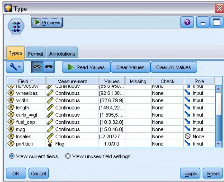
Abbildung 389. Typknoteneinstellungen
