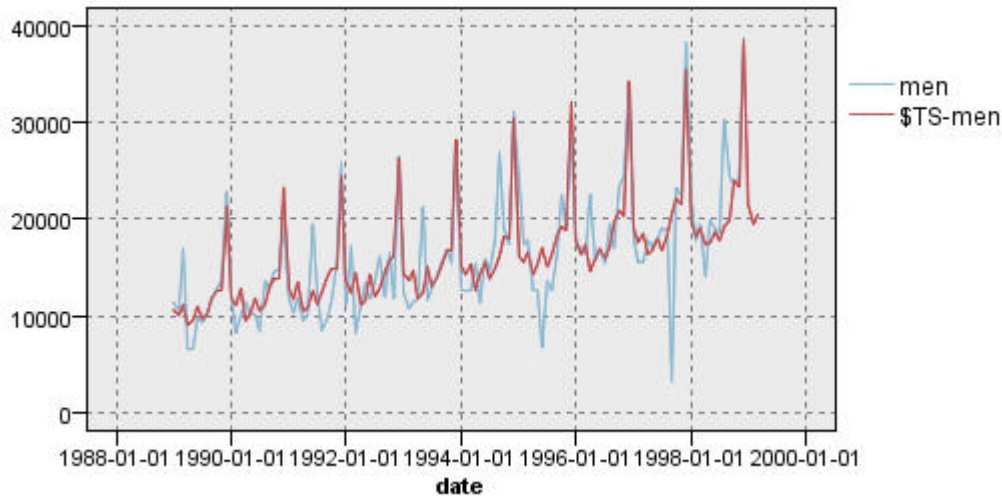
Abbildung 211. Multiplikatives Winters-Modell.
