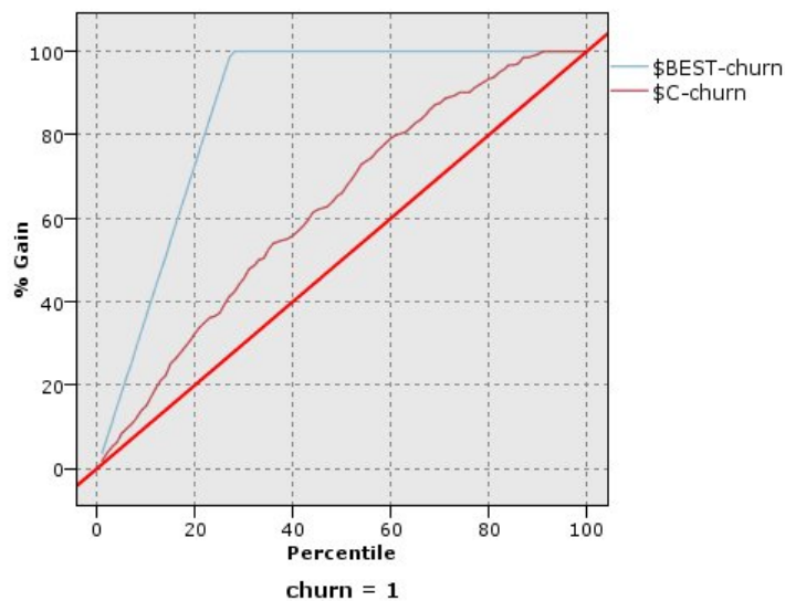
Abbildung 357. Gewinnndiagramm
