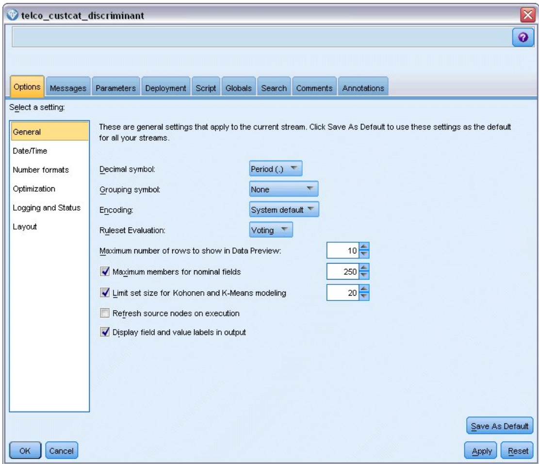
Abbildung 265. Streameigenschaften
