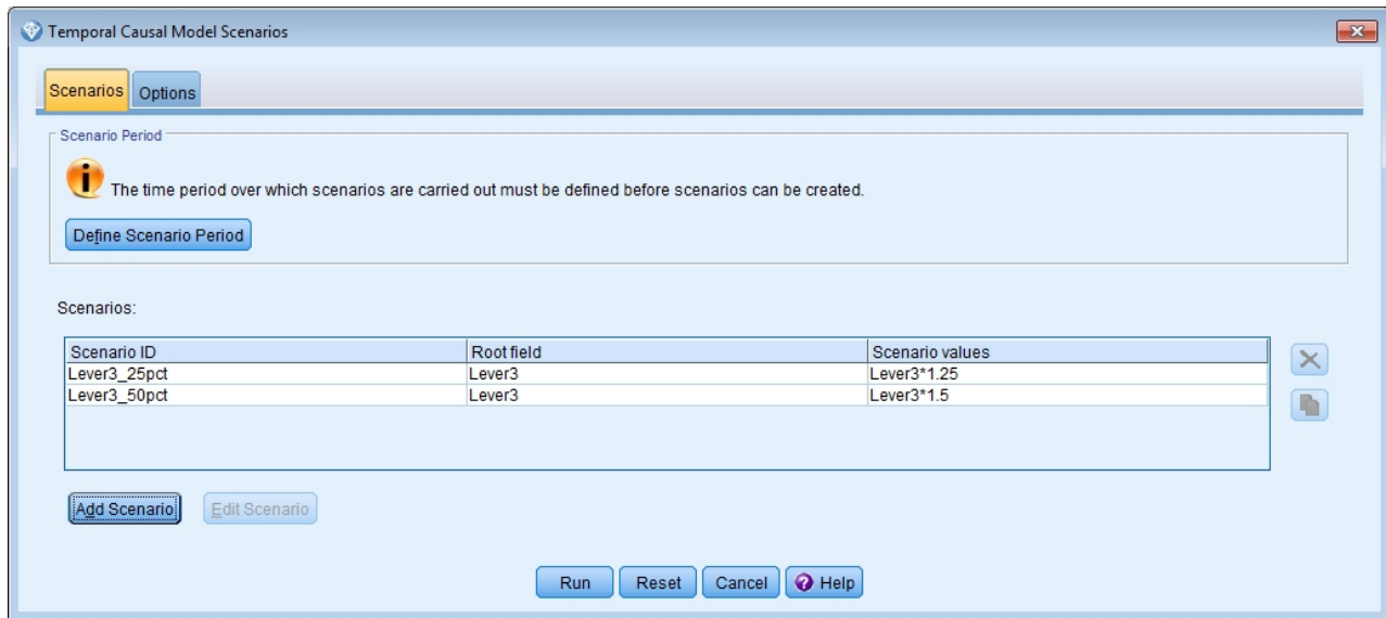
Abbildung 412. Szenarios
