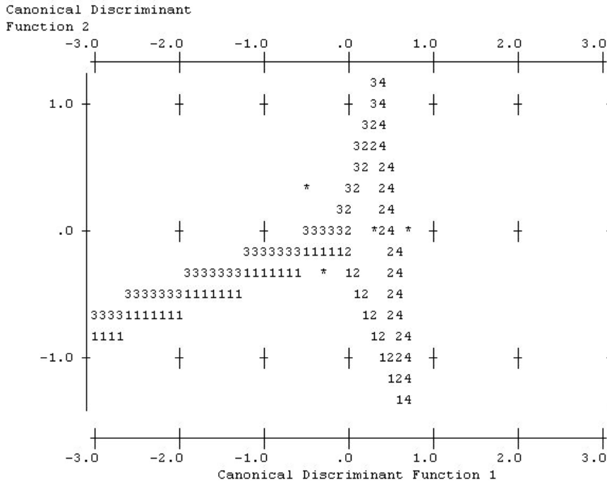
Abbildung 279. Territorien
