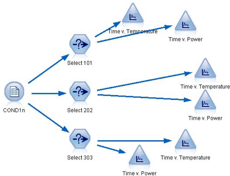
Abbildung 260. Condplot-Stream
