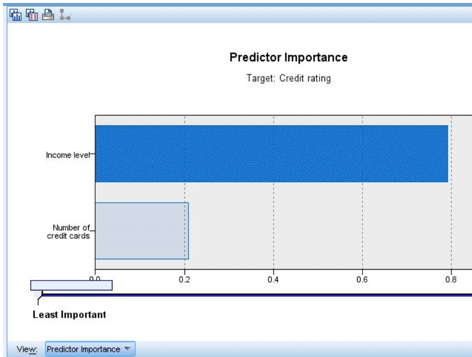
Abbildung 20. Prädiktoreinfluss - Diagramm
