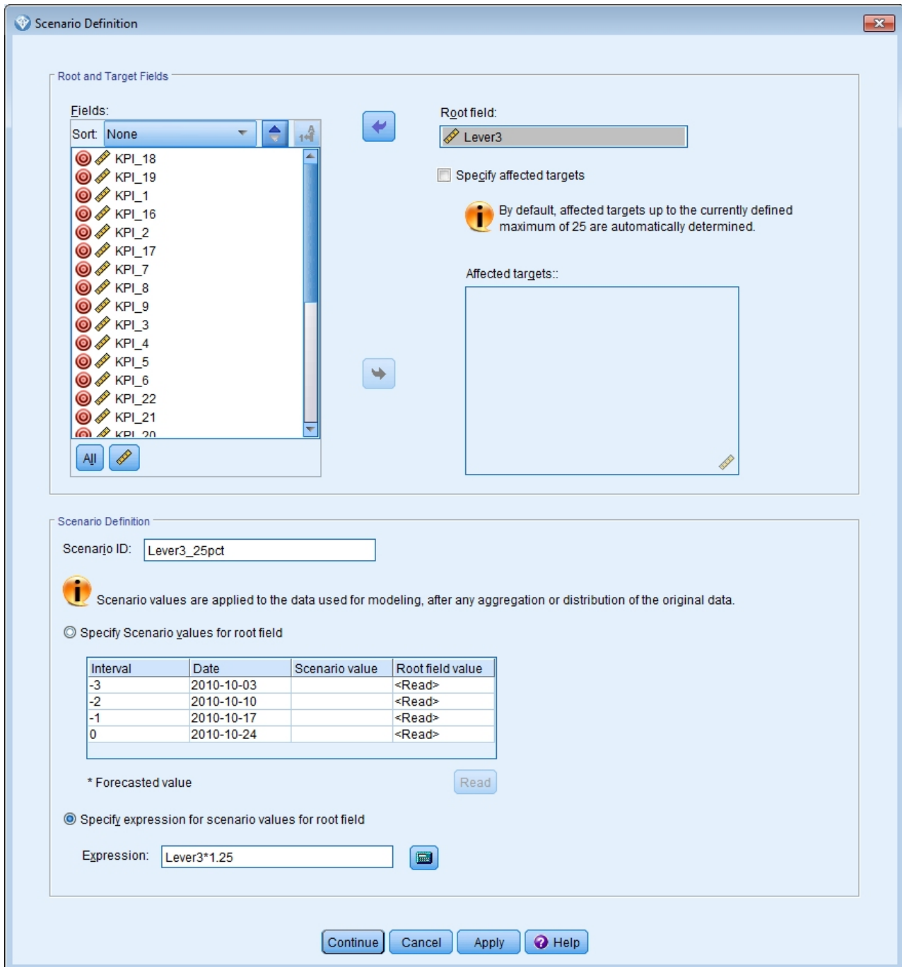
Abbildung 411. Szenariodefinition
