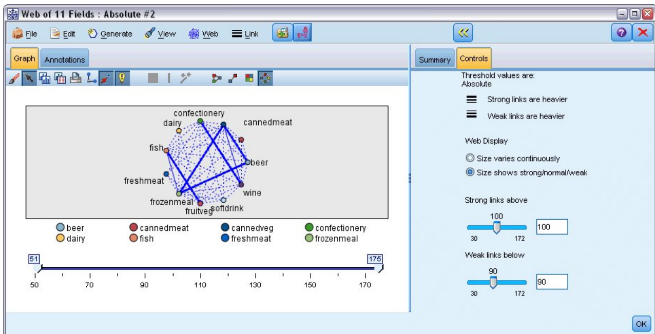
Abbildung 385. Beschränkte Netzdiagrammanzeige
