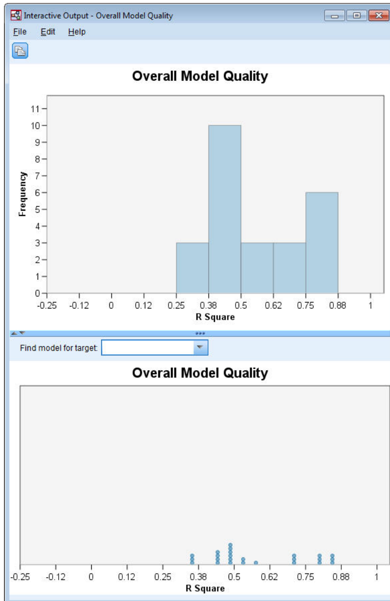
Abbildung 401. Gesamtmodellqualität
