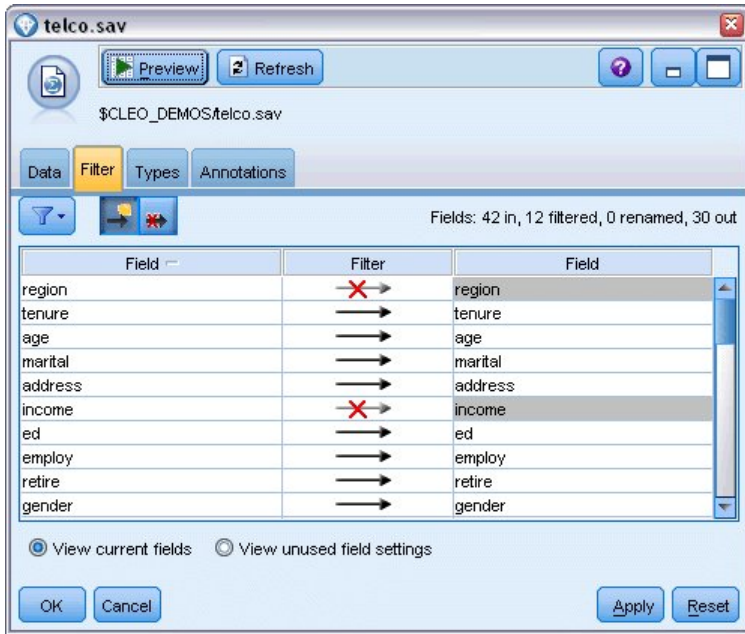
图 341. 过滤不需要的字段
