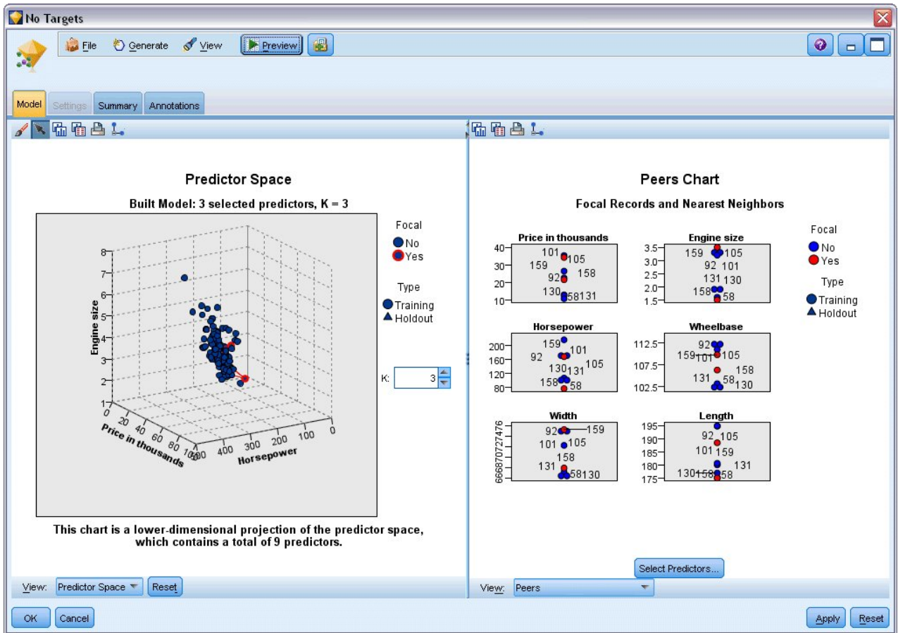
图 392. “模型查看器”窗口
