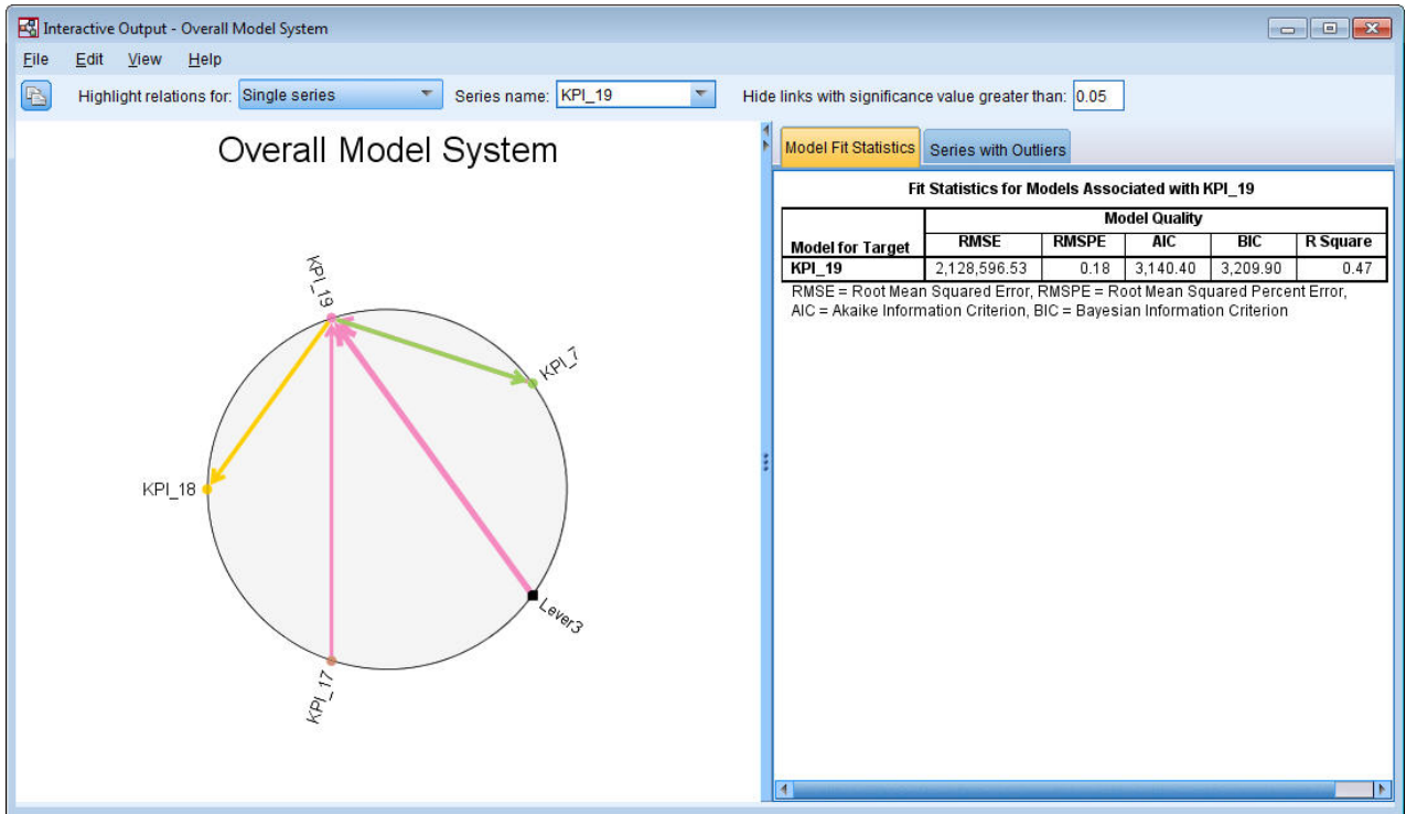
图 403. 单个序列的“总体模型系统”视图
