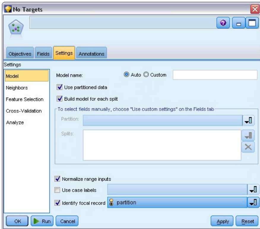
图 391. 使用分区字段识别焦点记录
