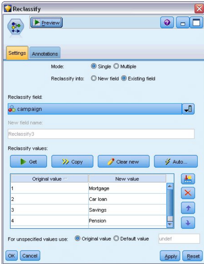
图 221. 对营销活动名称进行重新分类
