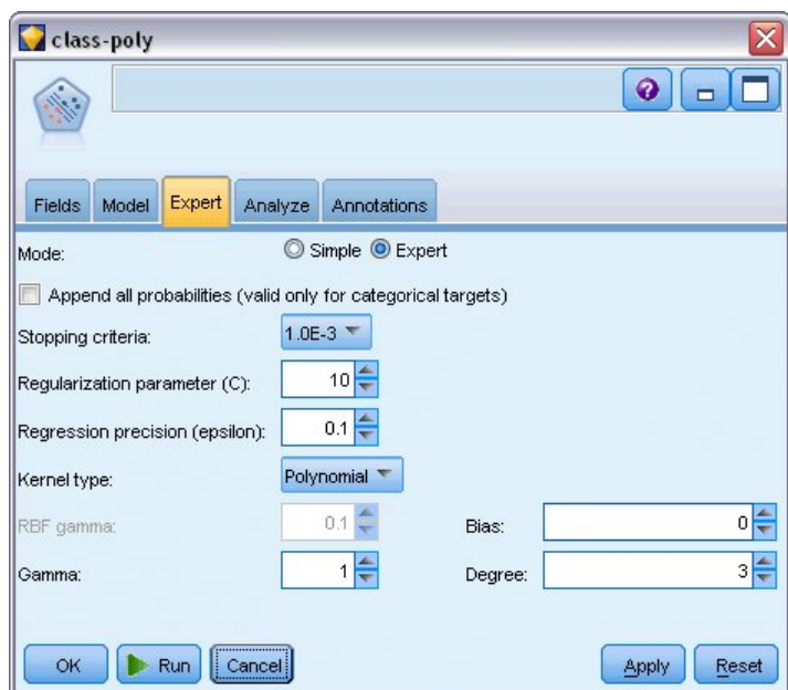
图 337. 多项式的“专家”选项卡设置
