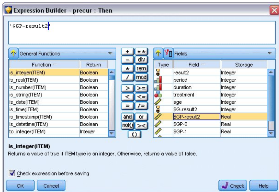
图 307. “派生”节点: Then 表达式的表达式构建器
