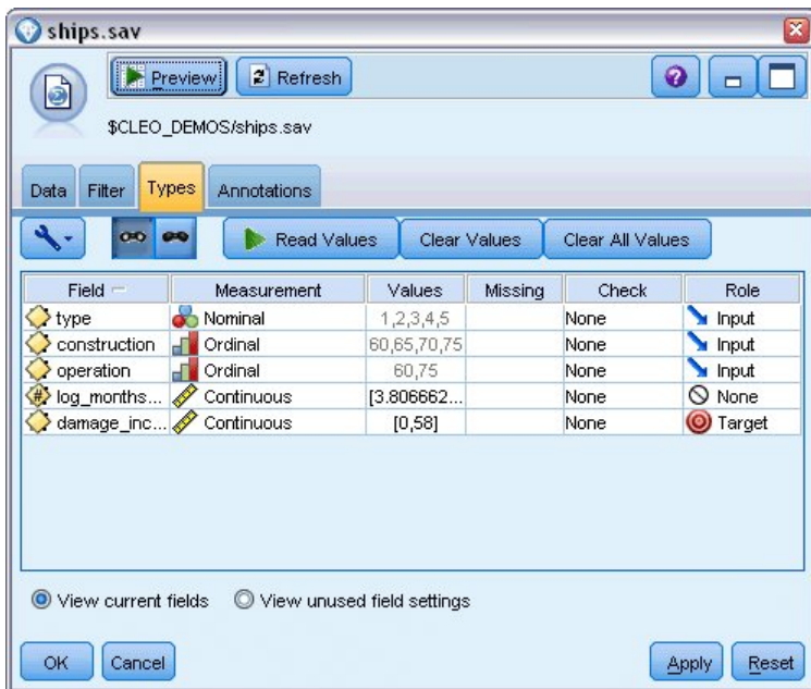
图 313. 设置字段角色
