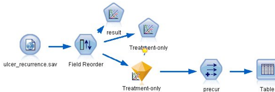
图 281. 用于预测溃疡复发的样本流
