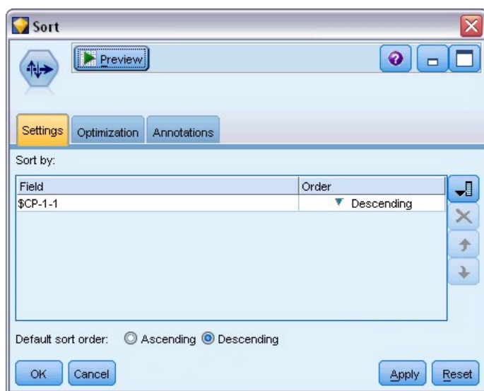
图 358. “排序”节点：“设置”选项卡
