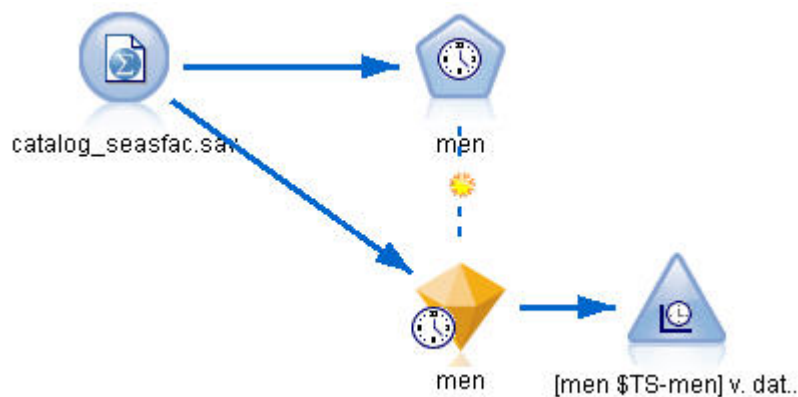
图 199. 预测产品分类销售情况
