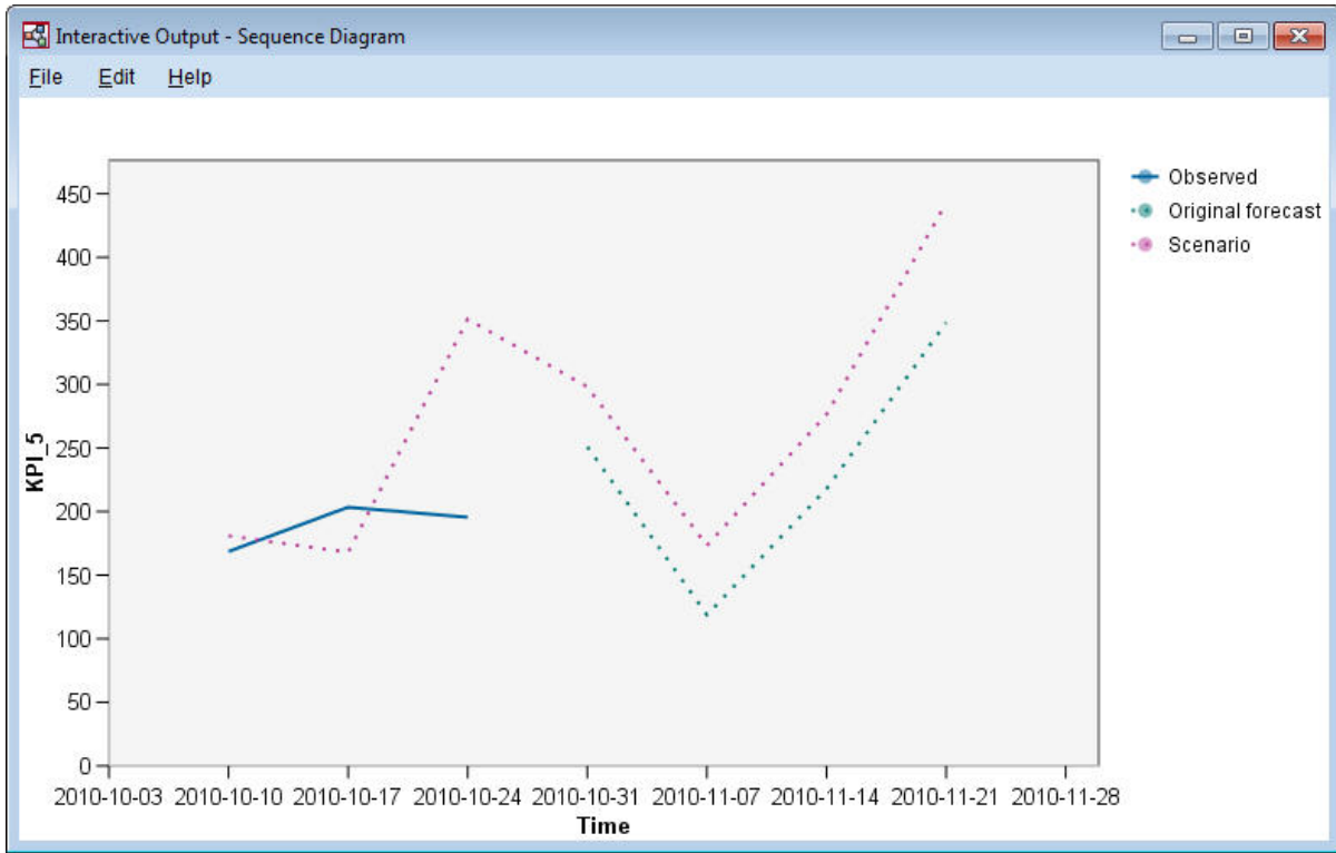
图 414. KPI_5 的时序图
