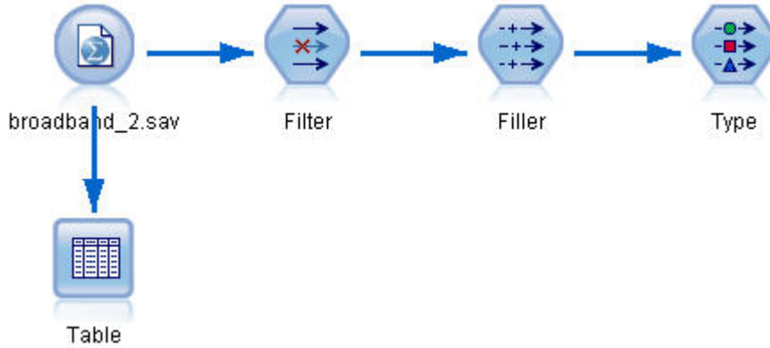
图 190. 打开流
