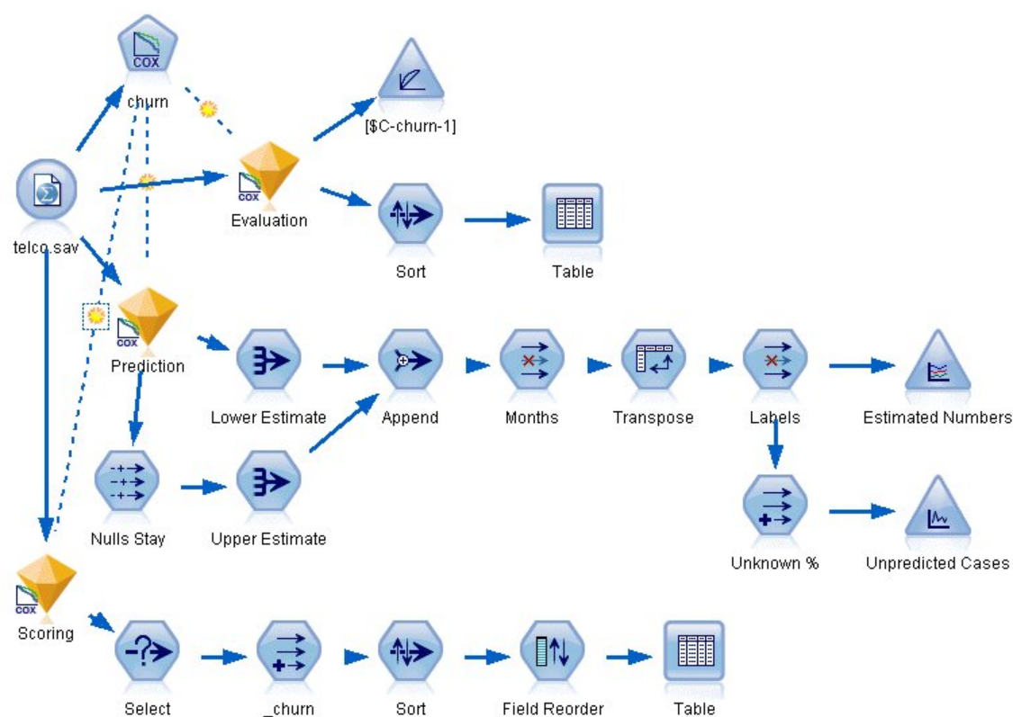
图 340. 用于分析流失时间的样本流
