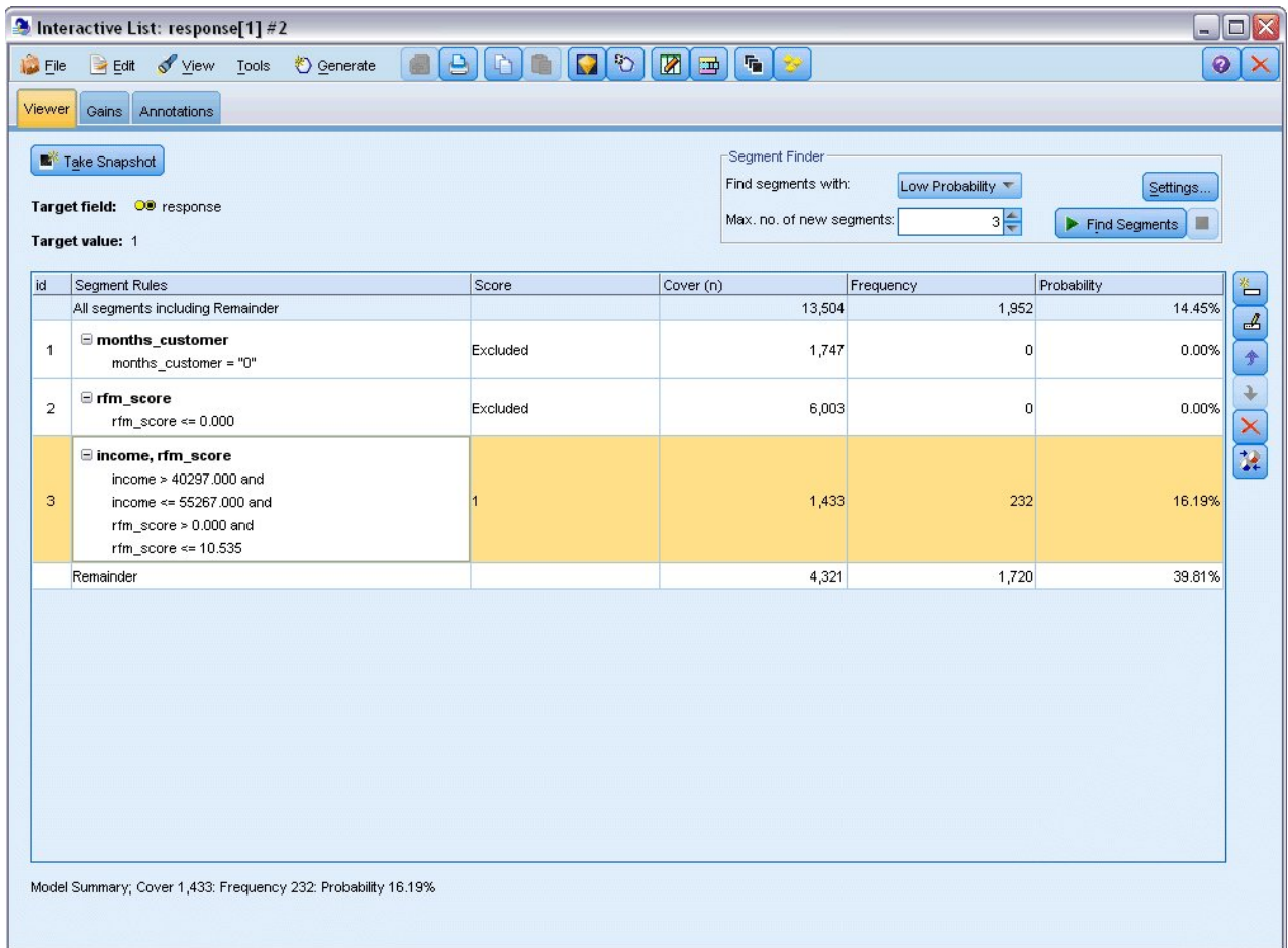
图 130. 排除段
