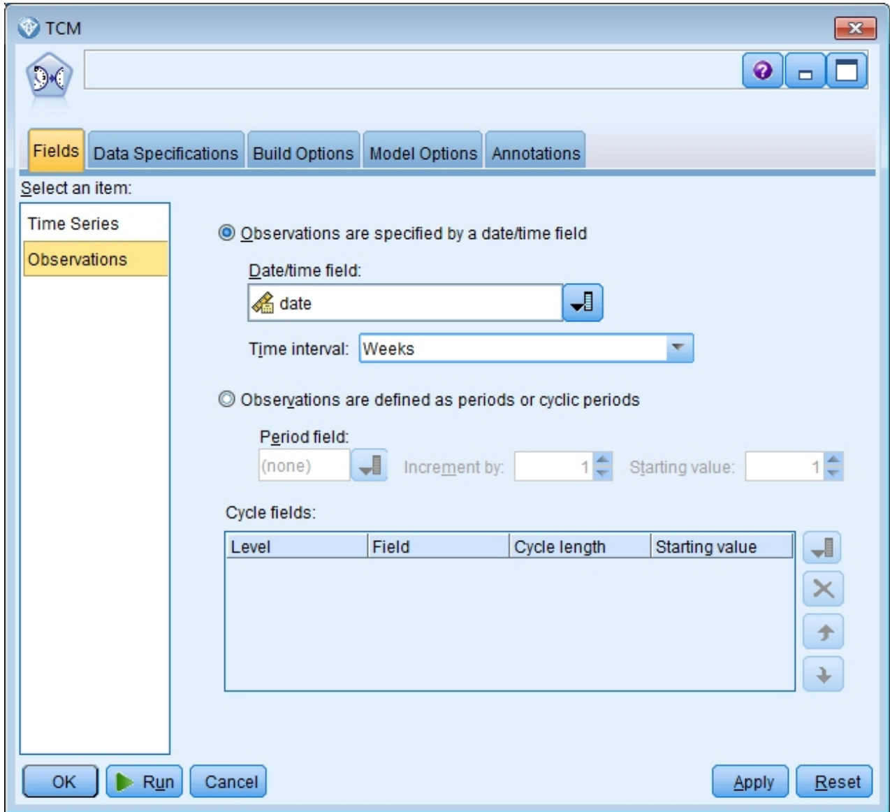
图 400. “时间因果关系建模”观测
