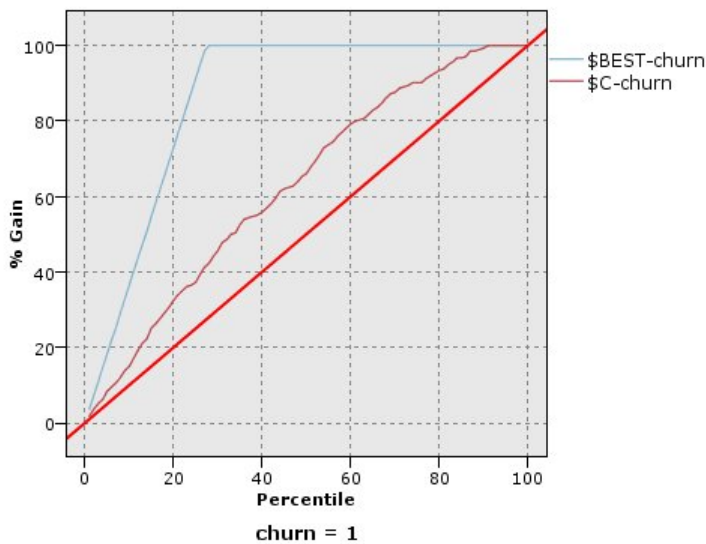
图 357. 增益图
