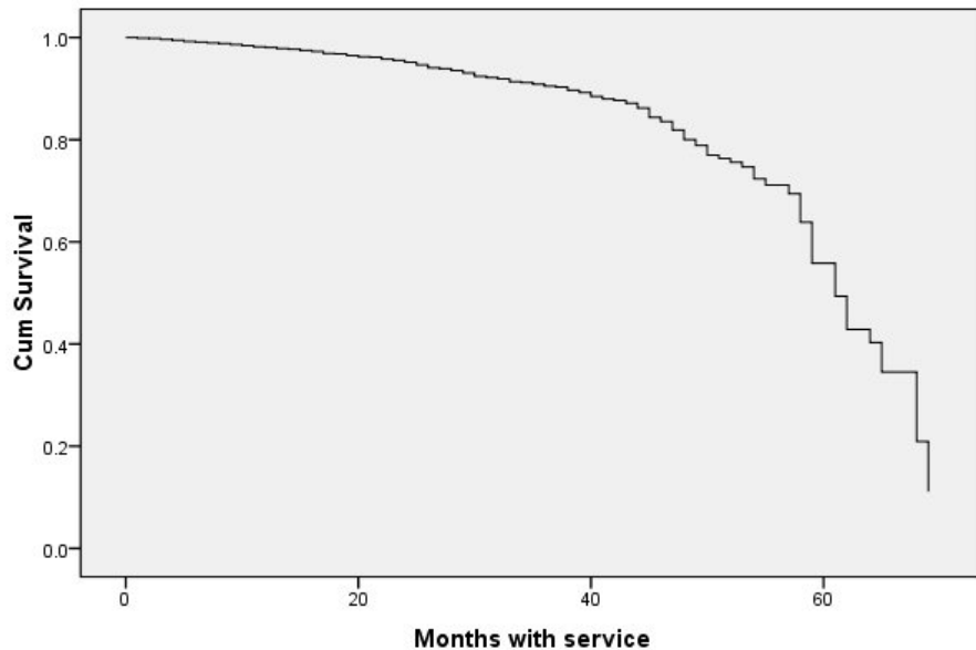
图 352. “平均”客户的存活曲线
