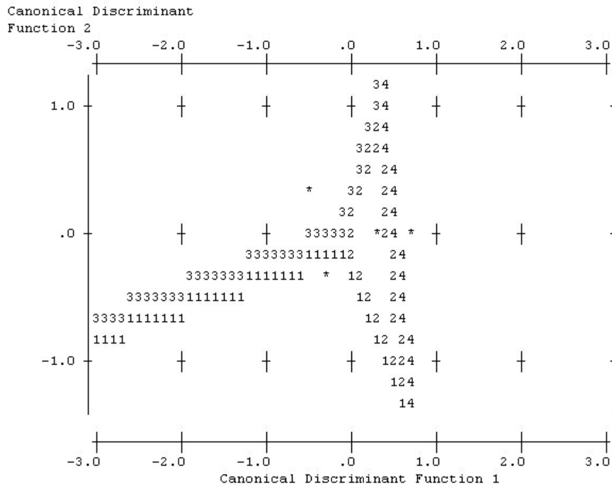
图 279. 区域图
