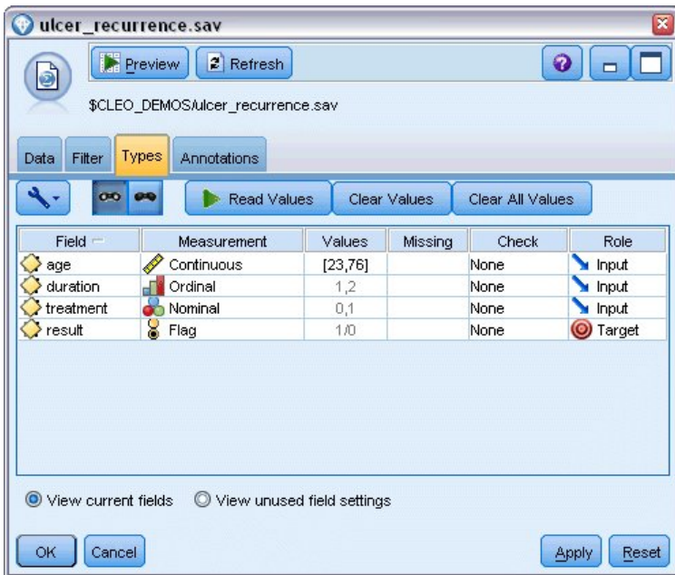
图 283. 设置字段角色
