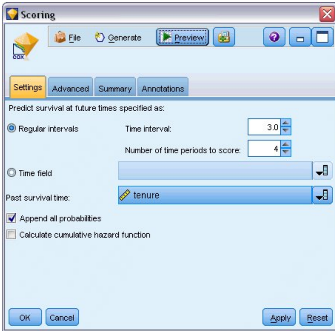
图 374. Coxreg 块：“设置”选项卡
