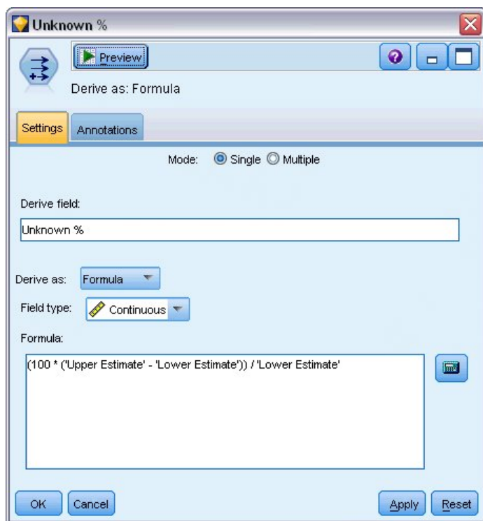
图 370. “派生”节点：“设置”选项卡
