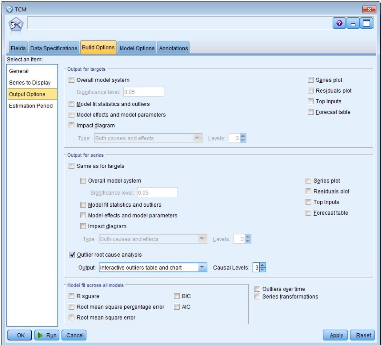
图 408. 时间因果关系模型输出选项
