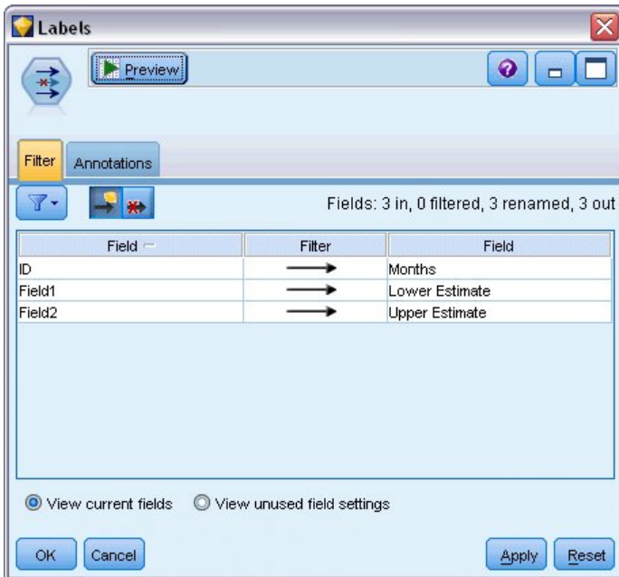
图 366. “过滤”节点：“过滤”选项卡
