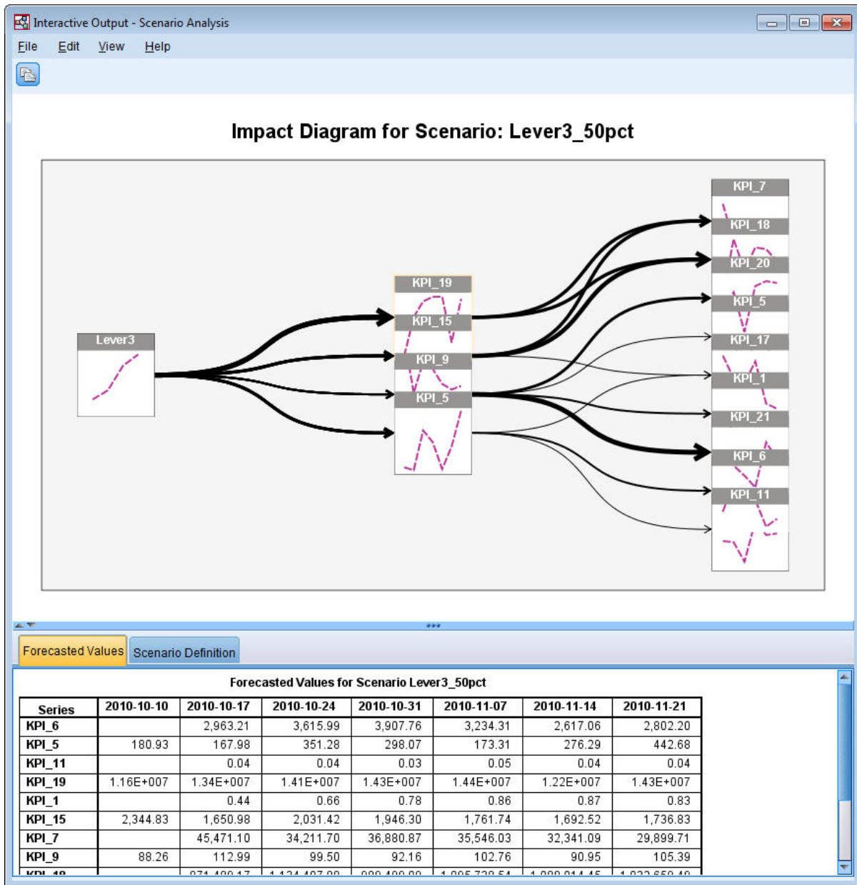
图 413. 方案影响图: Lever3_50pct
