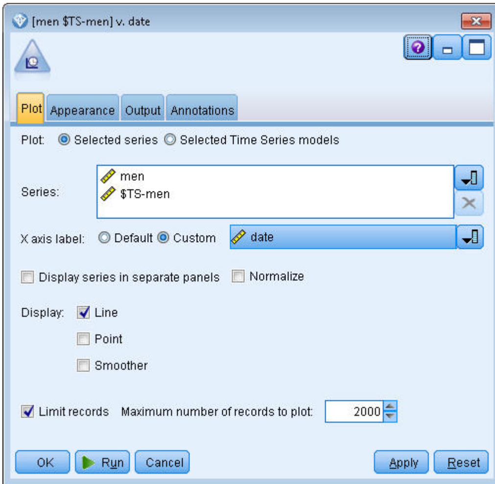
图 206. 绘制时间序列模型
