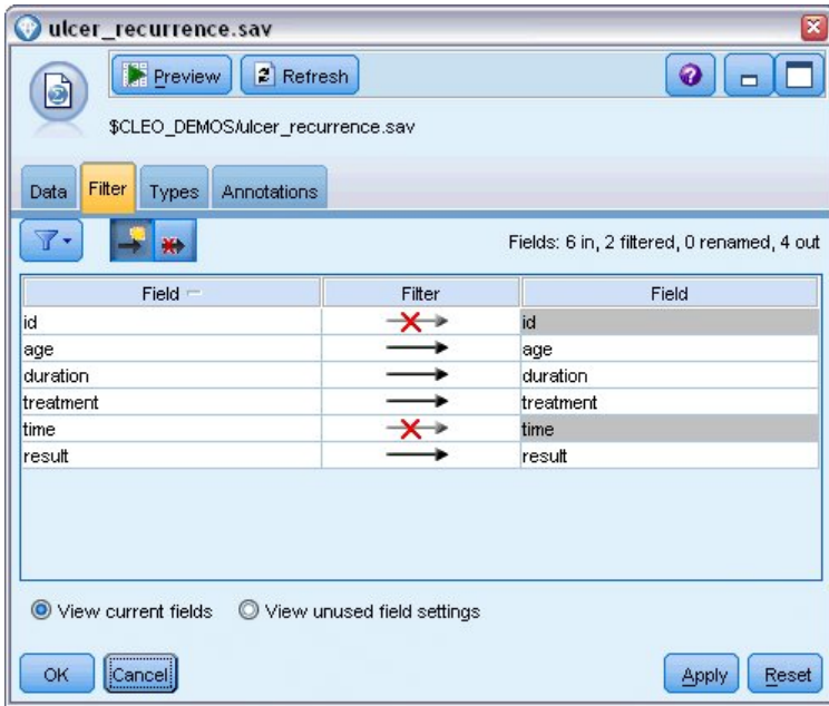
图 282. 过滤不需要的字段
