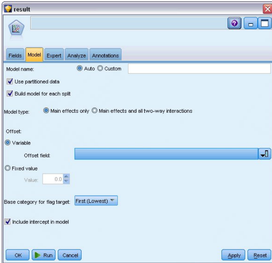
图 285. 选择模型选项
