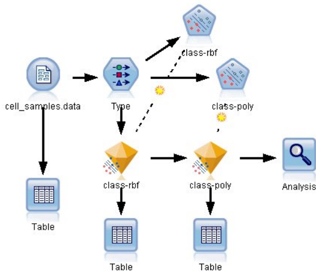
图 328. 用于显示 SVM 建模的样本流
