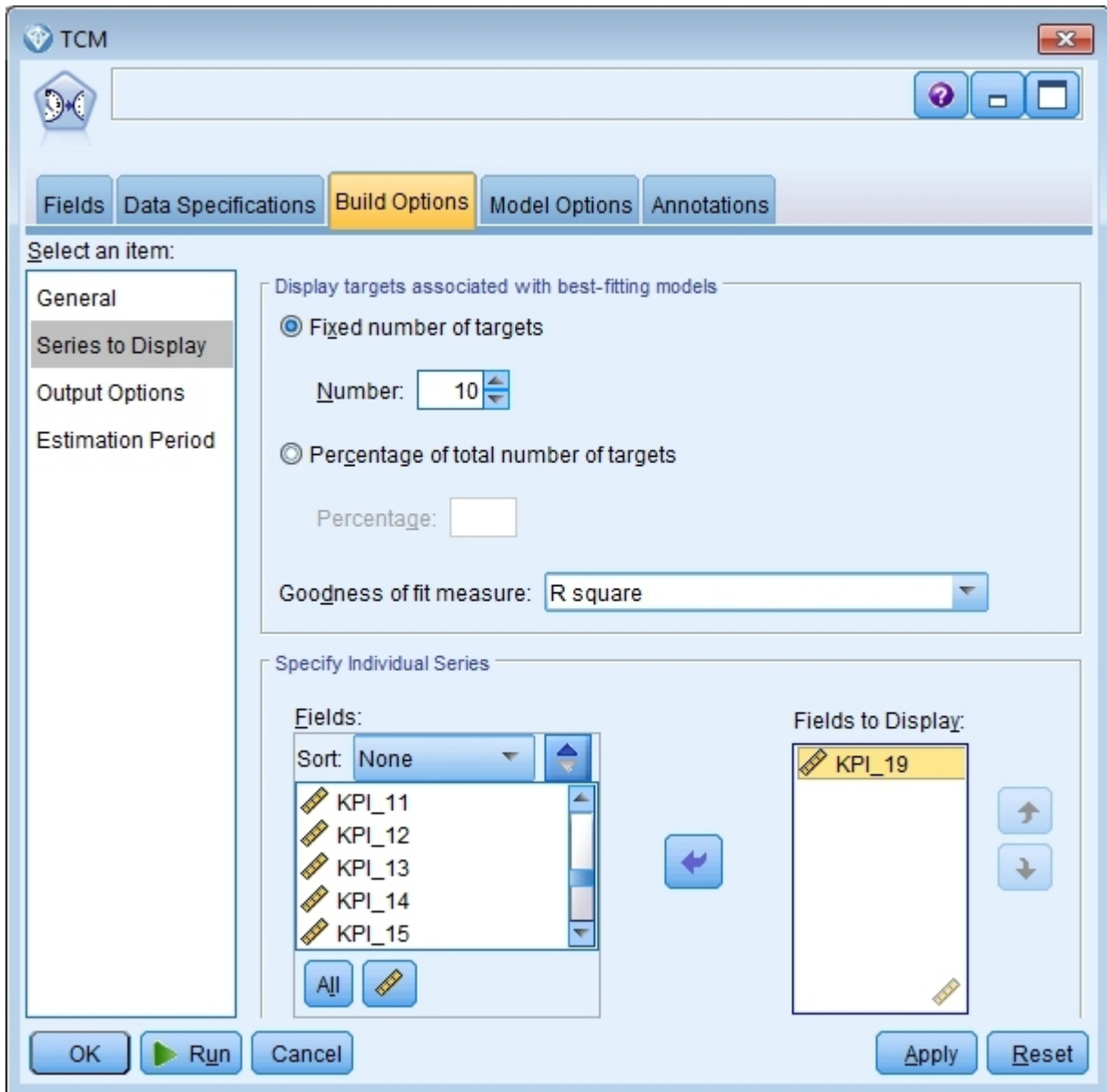
图 407. 要显示的时间因果关系模型序列
