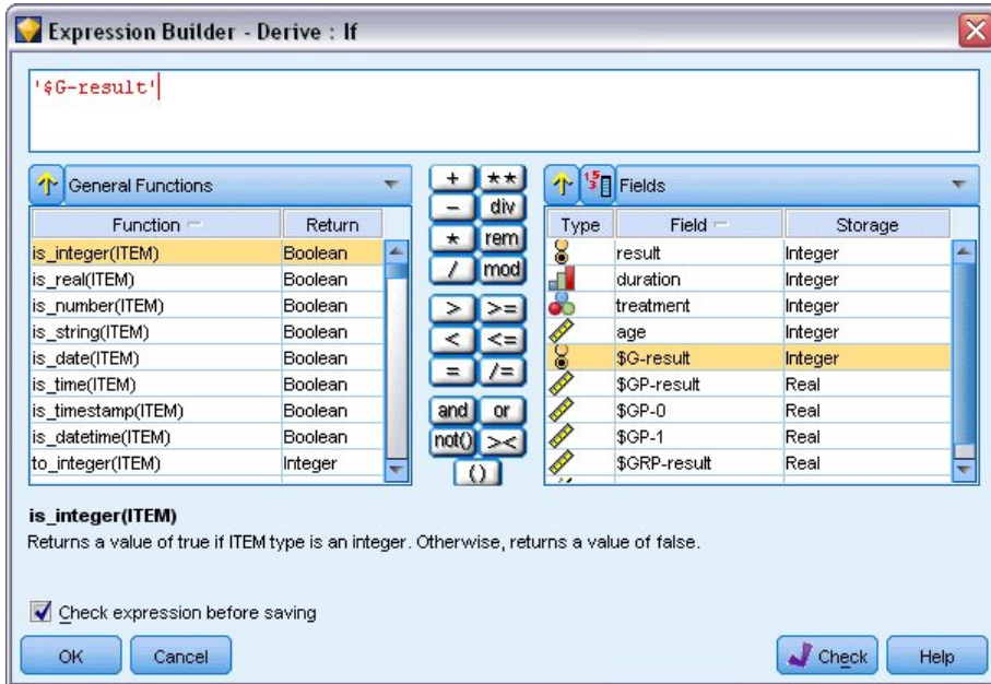
图 291. “派生”节点: If 条件的表达式构建器
