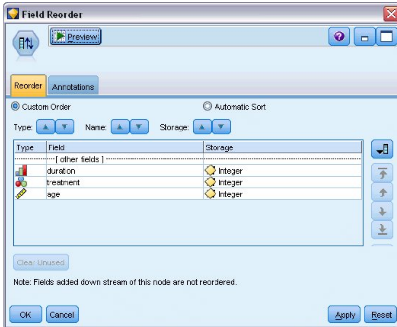
图 284. 对字段进行重新排序以使其按预期输入到模型中
