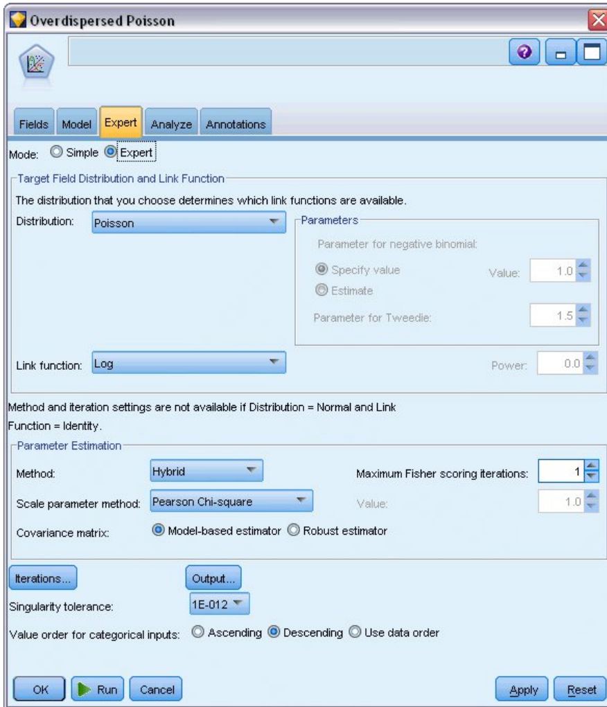
图 315. 选择专家选项
