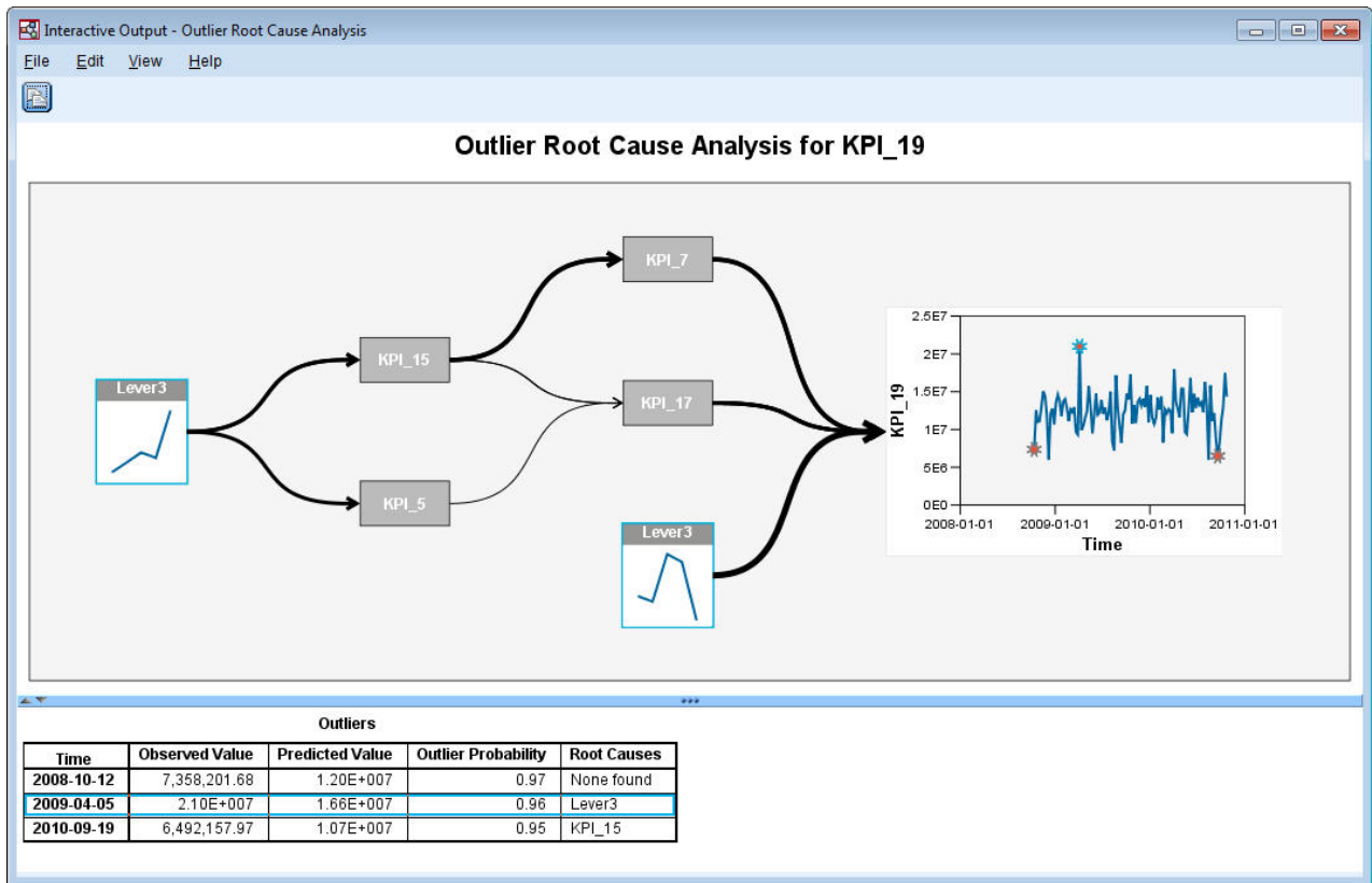
图 409. KPI_19 的离群值根本原因分析
