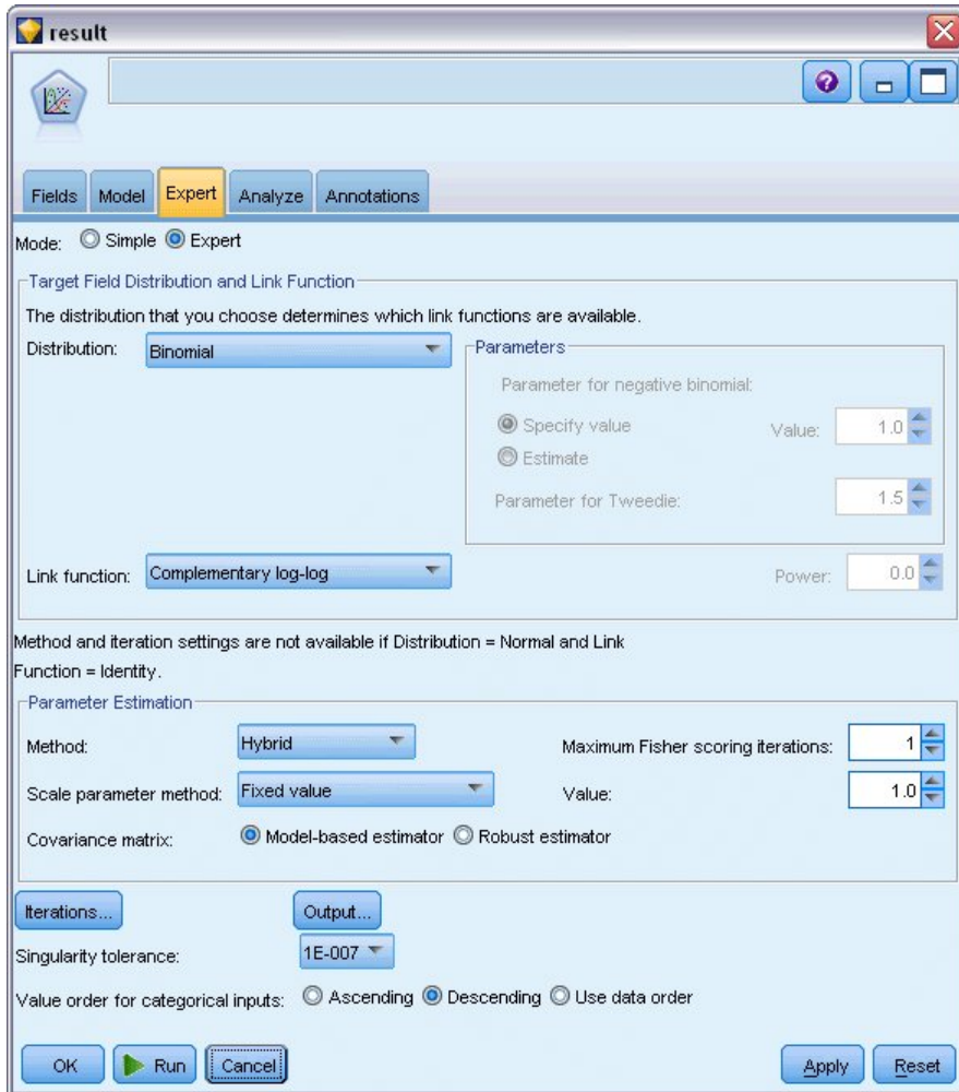
图 301. 选择专家选项
