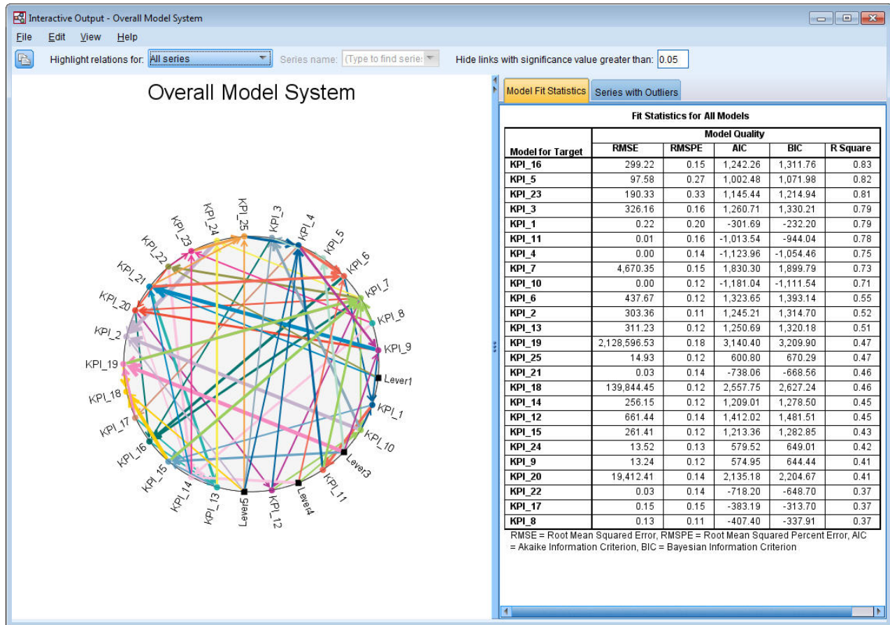
图 402. 所有序列的"总体模型系统"视图
