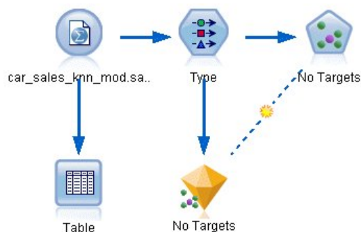
图 387. KNN 建模的样本流
