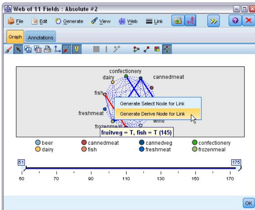
图 386. 派生每个客户组的标志
