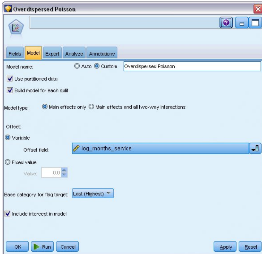
图 314. 选择模型选项
