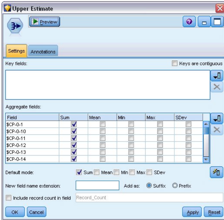
图 363. “汇总”节点：“设置”选项卡
