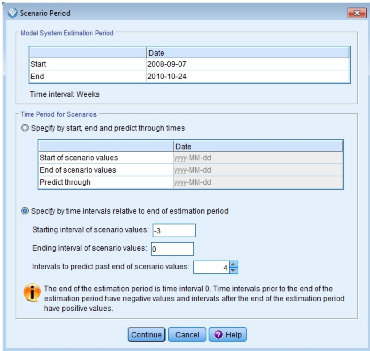
图 410. 方案期
