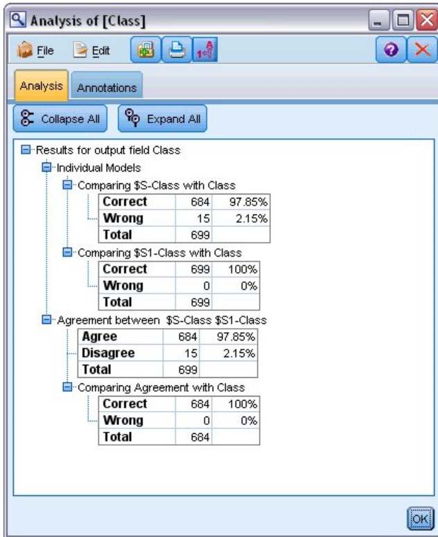
图 339. “分析”节点
