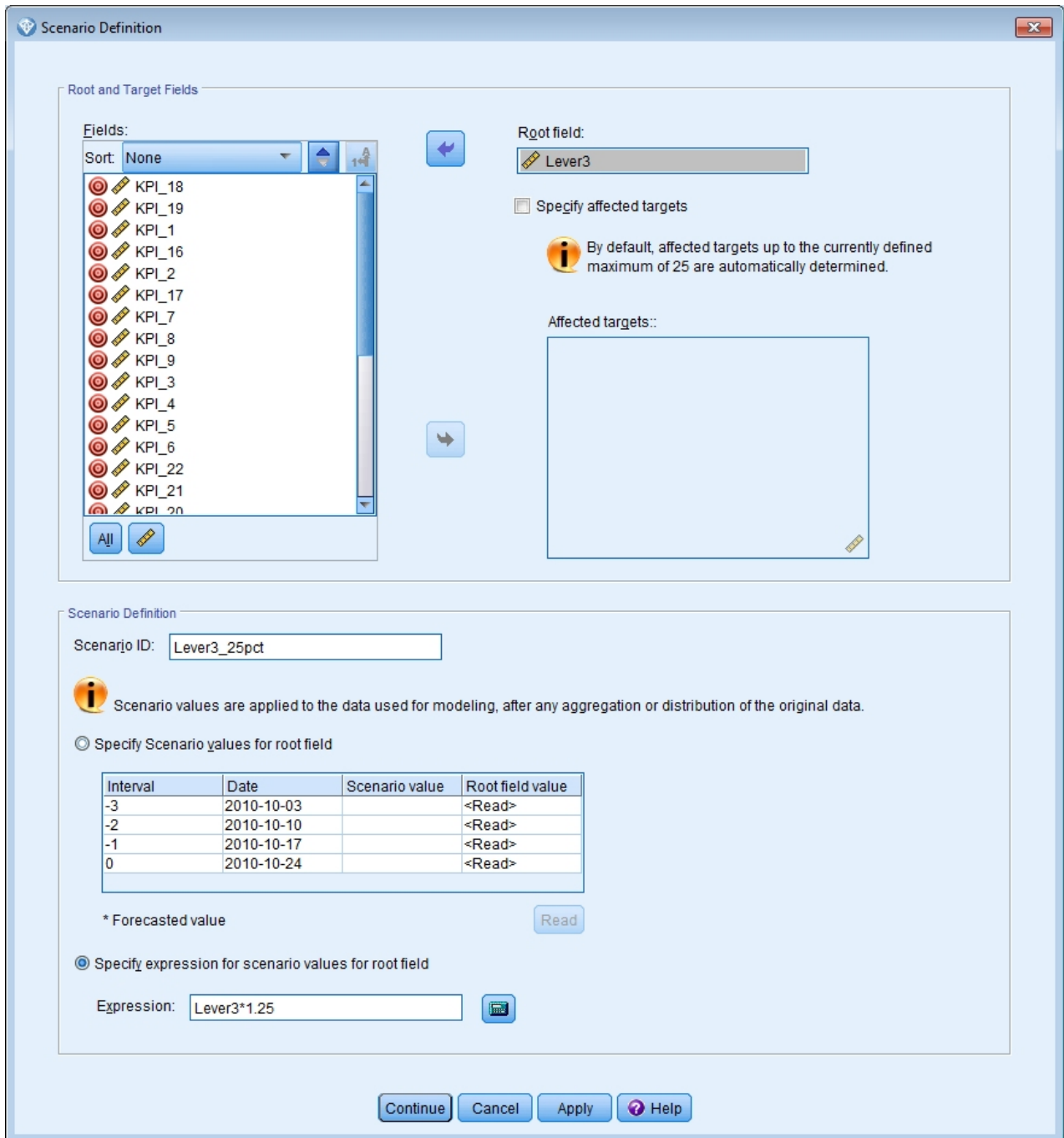
图 411. 方案定义
