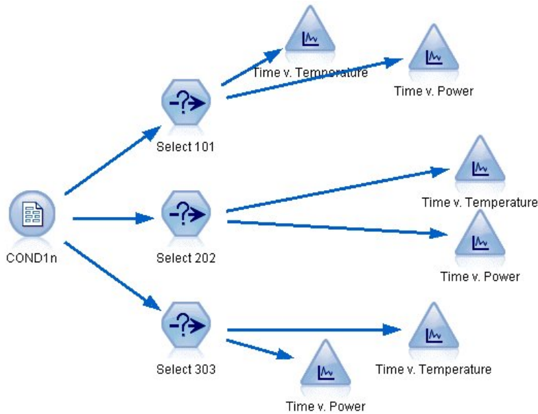
图 260. Condplot 流
