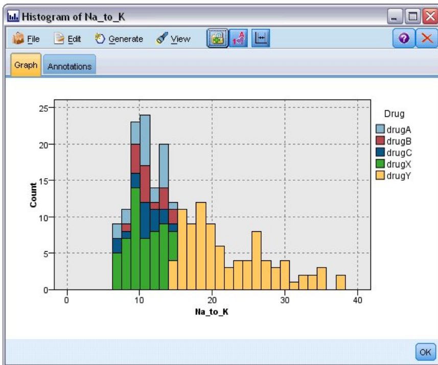
图 92. 直方图显示
