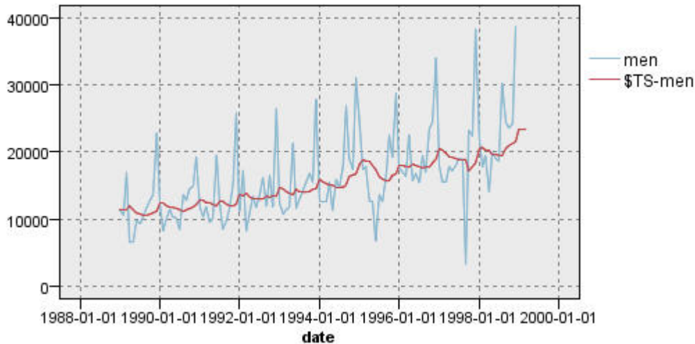
图 207. 简单指数平滑法模型
