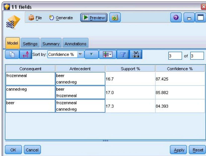
图 383. 关联规则
