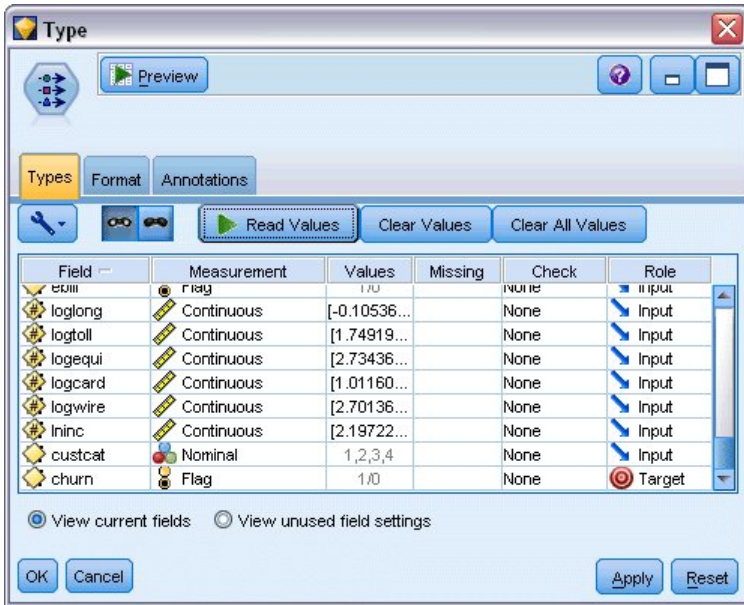
图 61. 设置目标
