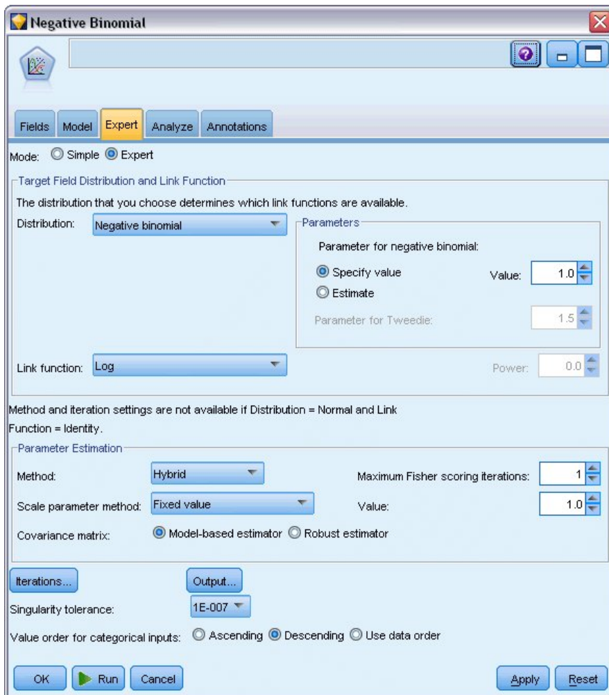
图 320. “专家”选项卡
