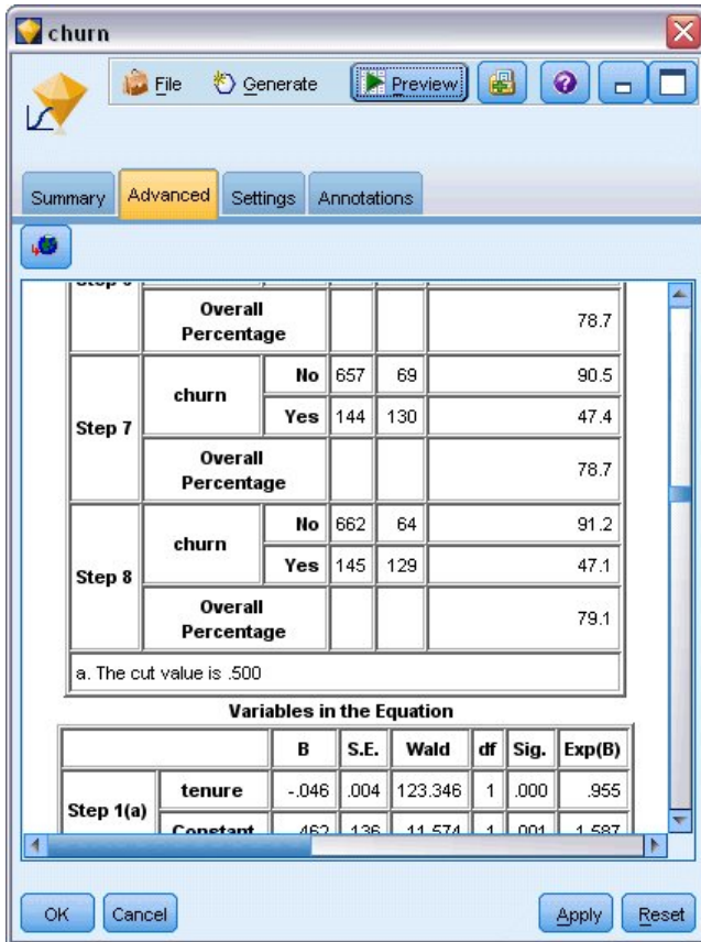
图 169. 分类表 - 块 1
