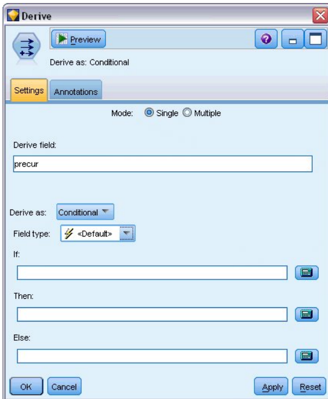
图 305. “派生”节点设置选项
