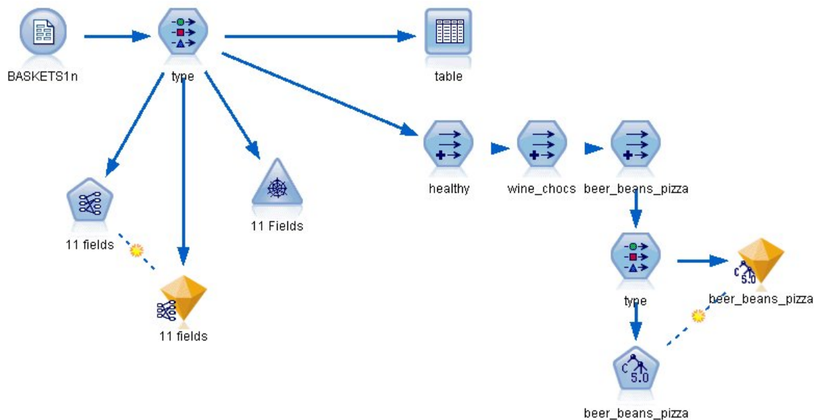
图 381. 购物规则流
