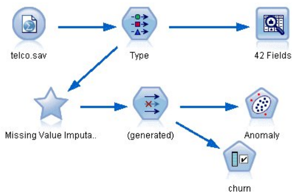
图 60. 构建流
