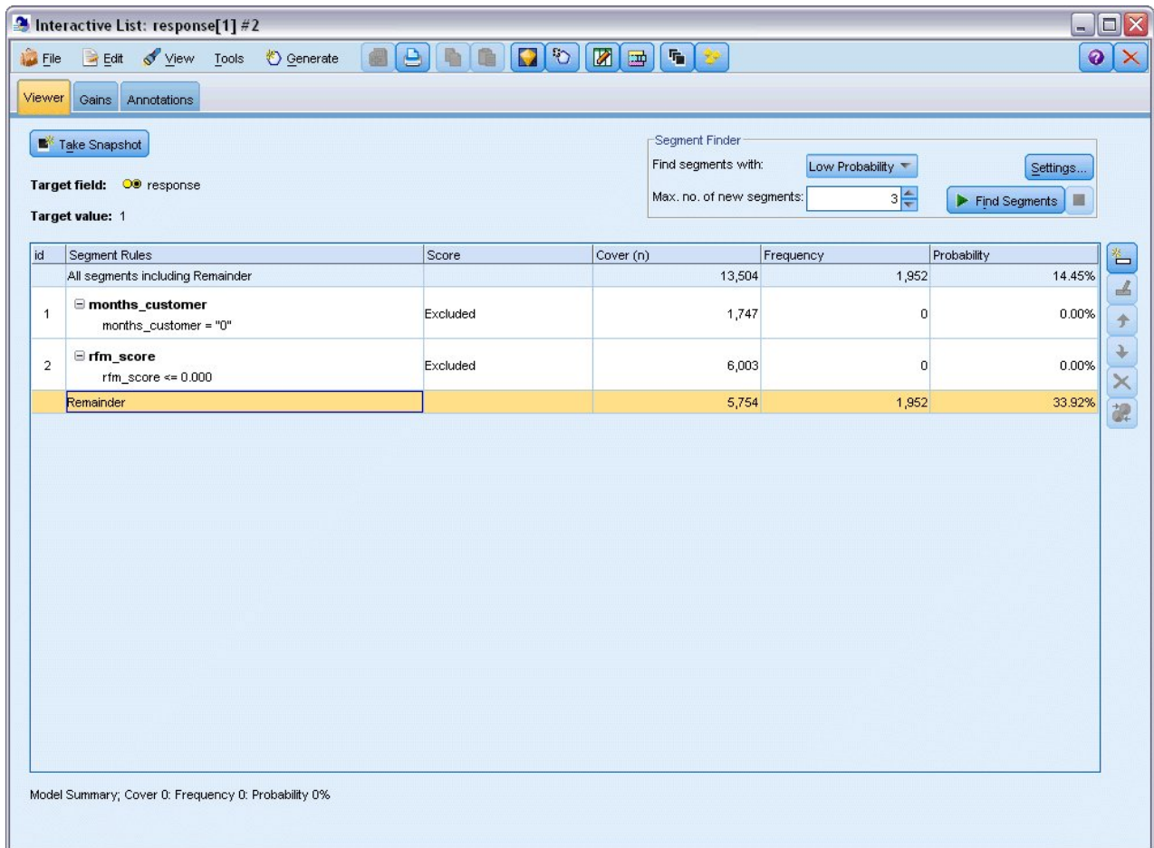
图 131. 选择段
