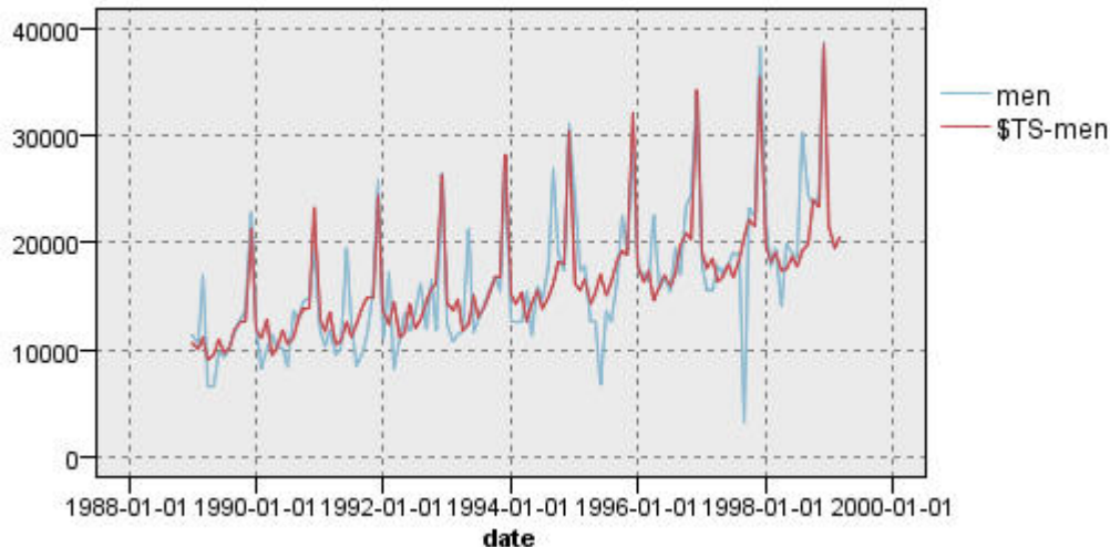
图 211. 温特斯乘法模型
