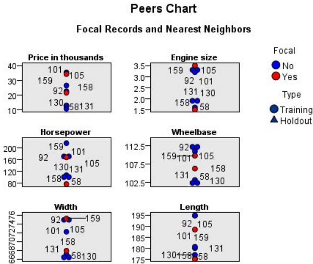
图 394. 对等图表
