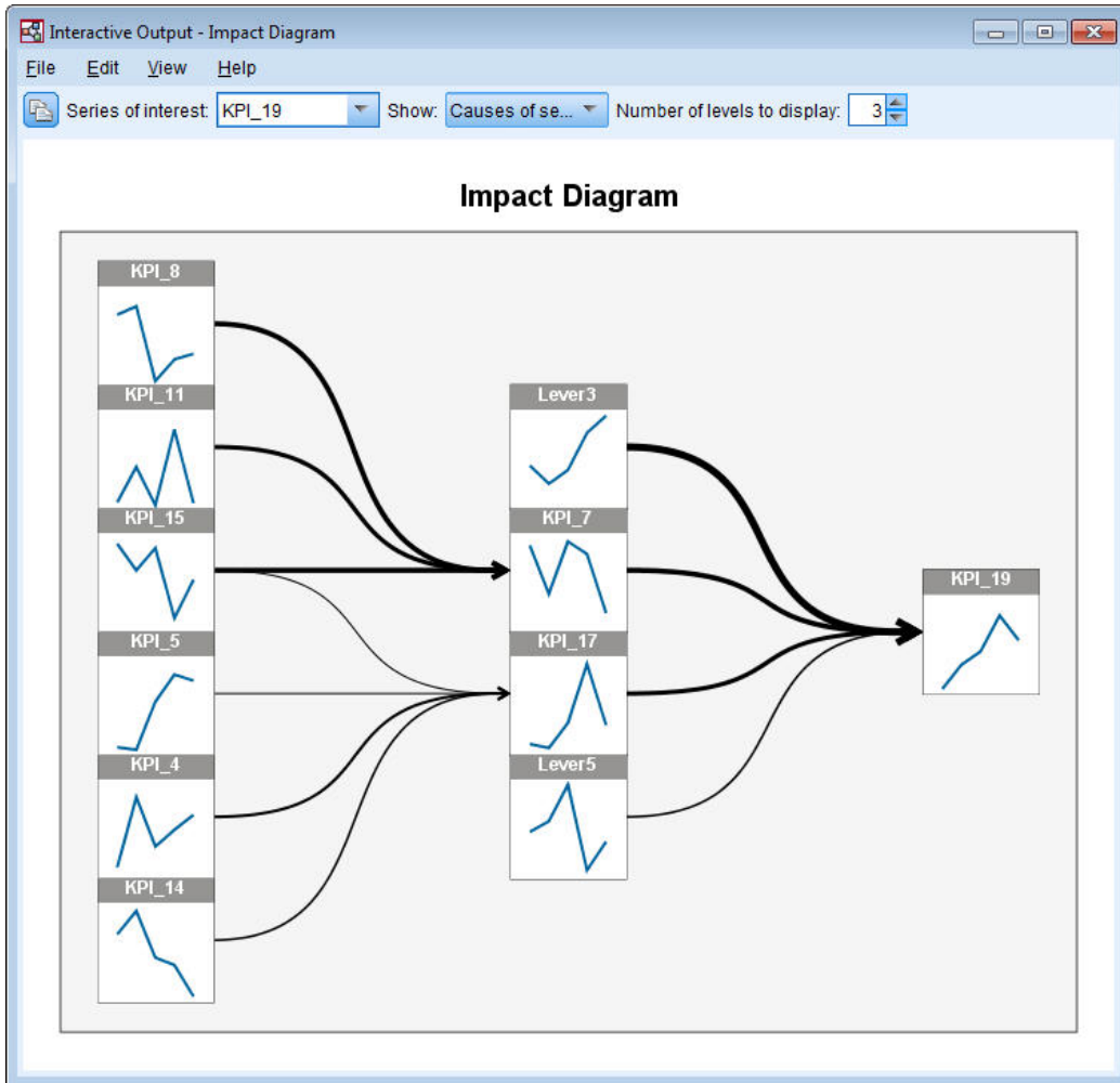
图 406. 原因影响图
