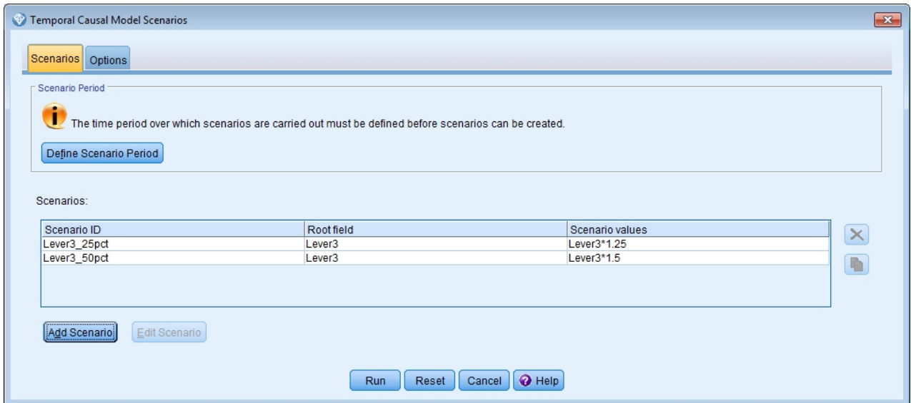
图 412. 方案
