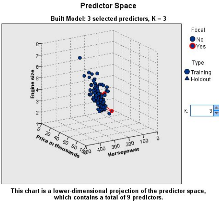
图 393. 预测变量空间图表
