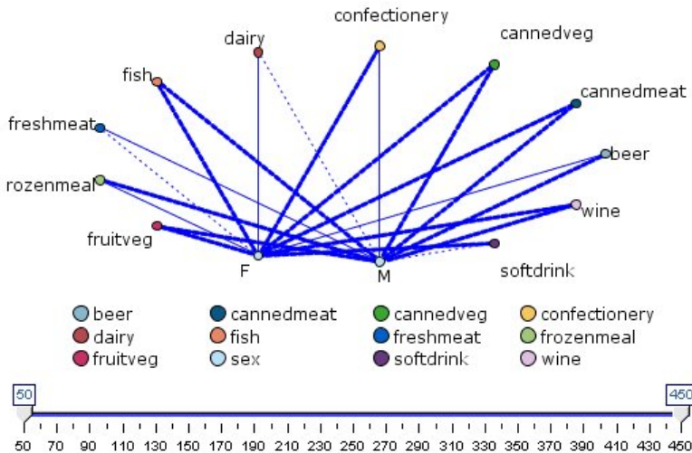
그림 36. 식료품 항목의 구매와 성별 간의 관계를 보여주는 방향성이 있는 웹 그래프
