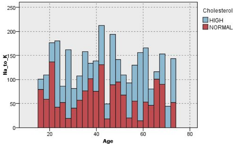
Rysunek 34. Wykres przedziałowy bez osi z nałożeniem koloru dla wartości Cholesterol
