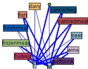
Rysunek 38. Wykres sieciowy przedstawiający etykiety jako węzły
