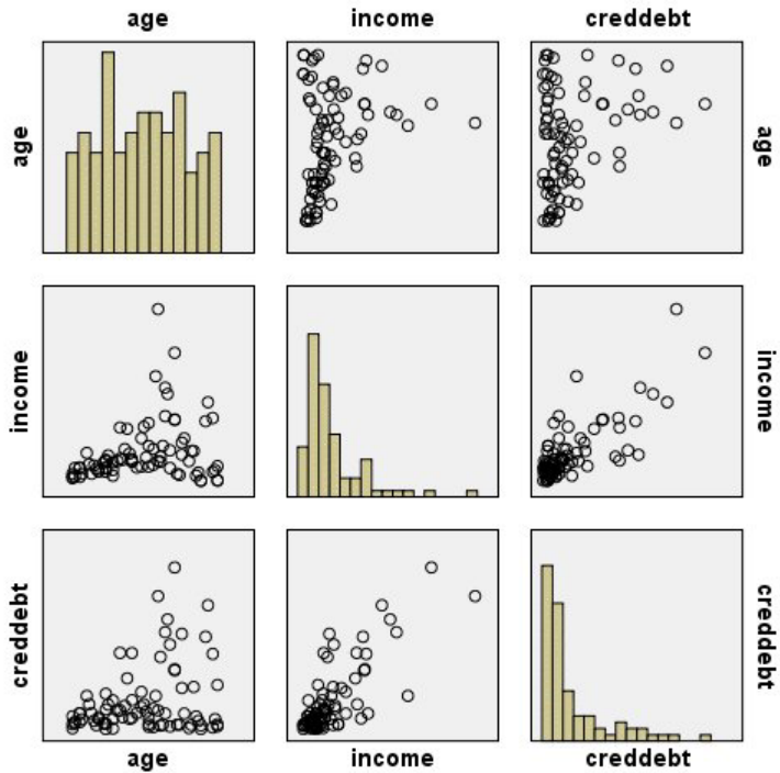
그림 17. 산점도 행렬(SPLOM)
