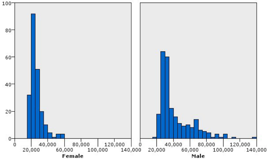
그림 12. 패널링된 히스토그램
