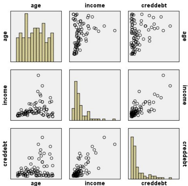
Abbildung 17. Streudiagrammmatrix (SPLOM)
