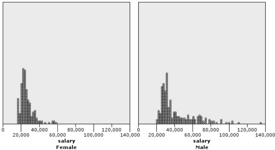
Abbildung 13. Unterteiltes Punktdiagramm
