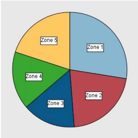
Abbildung 15. Kreisdiagramm
