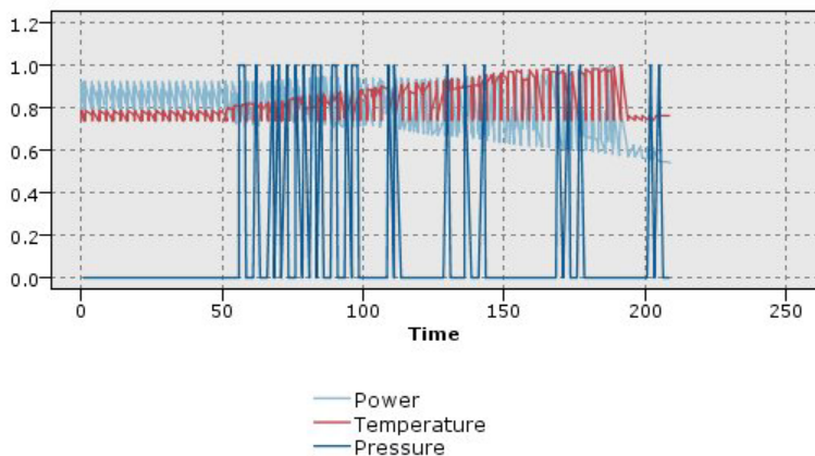
图 27. 显示压力散点图的标准化多重散点图
