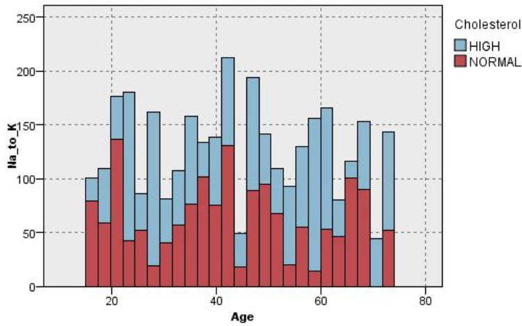
图 36. 显示没有 z 轴的集合图，并将胆固醇作为交叠以颜色标出
