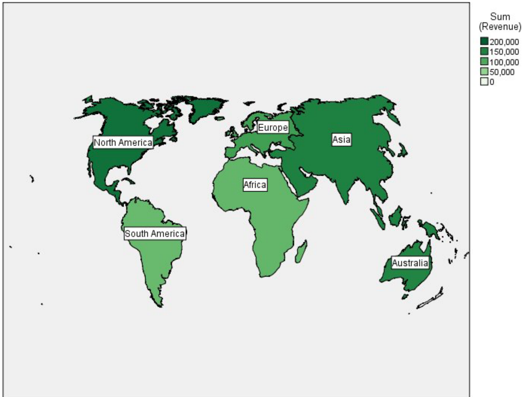
图 18. 总和的等值线图
