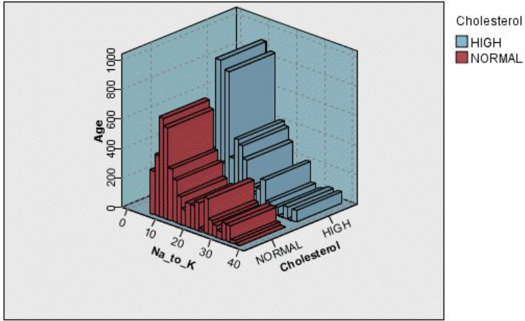
图 35. 三维集合图显示针对高、正常胆固醇水平，Na_to_K 相对于 Age 的合计
