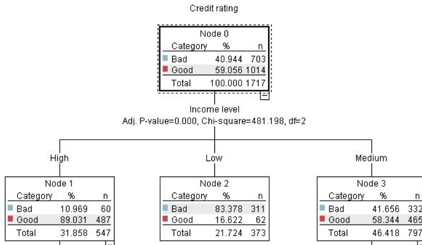
그림 1. 단순 의사결정 트리 모델
