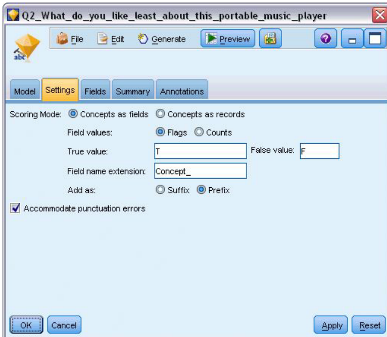
Figura 6. Finestra di dialogo del nugget del modello di concetto di estrazione testo: scheda Impostazioni
