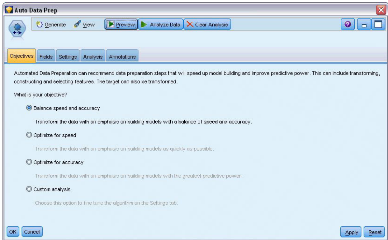
Abbildung 53. ADP-Standardziele
