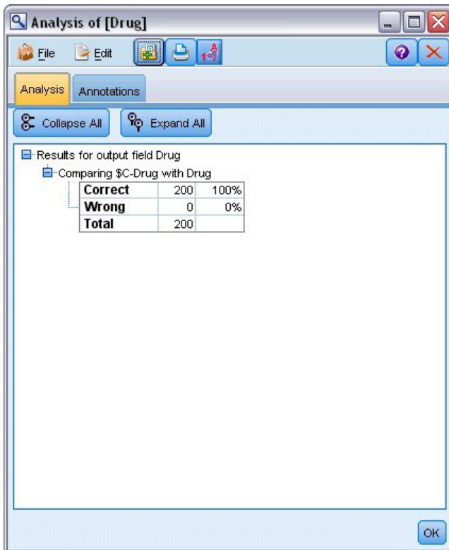
Abbildung 101. Analyseknott - Ausgabe
