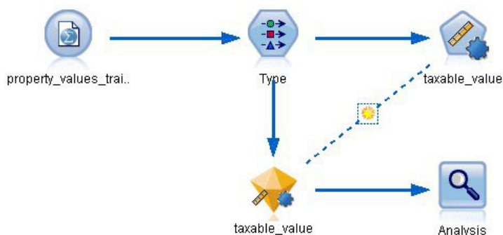
Abbildung 42. Auto-Numerisch - Beispielstream
