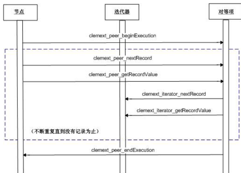
图 98. 典型执行块
