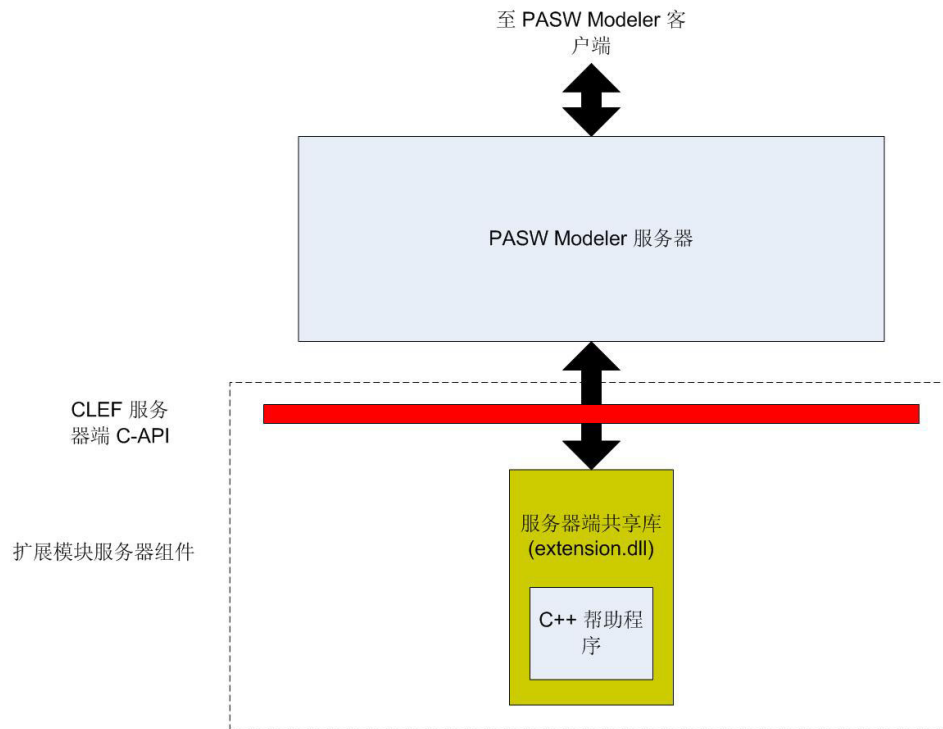
图 2. 服务器端组件
