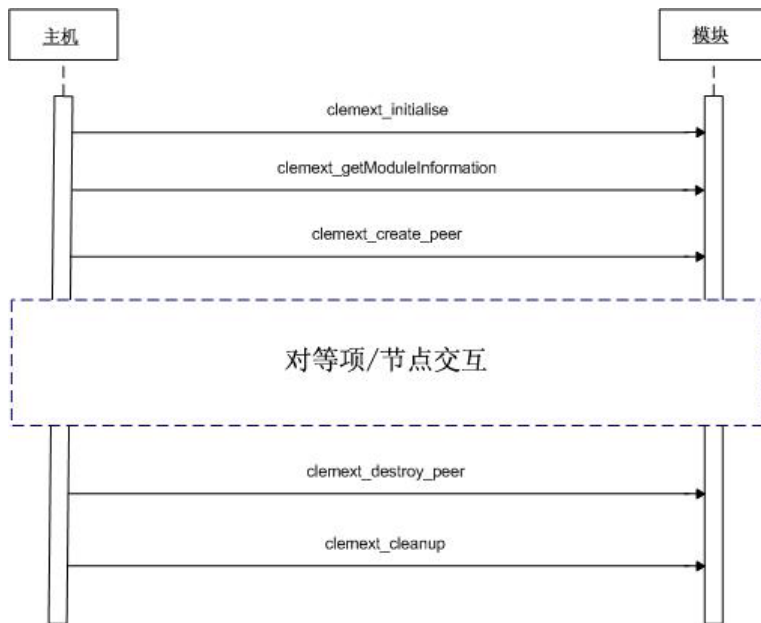
图 96. 典型过程流
