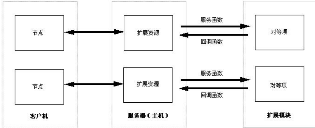
图 95. CLEF API 体系结构
