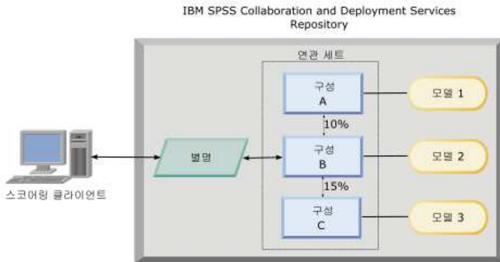
그림 10. A/B 검정 예제
