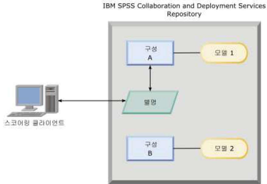
그림 7. 스코어링 구성의 예제 별명
