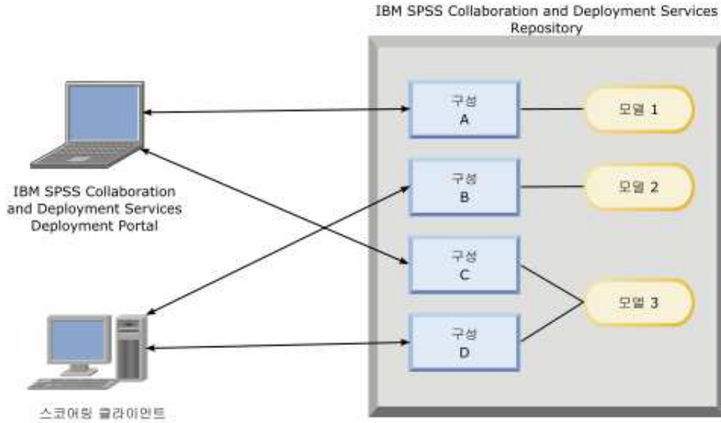
그림 6. 일반 스코어링 아키텍처
