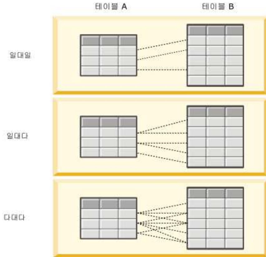
그림 4. 테이블 관계 유형
