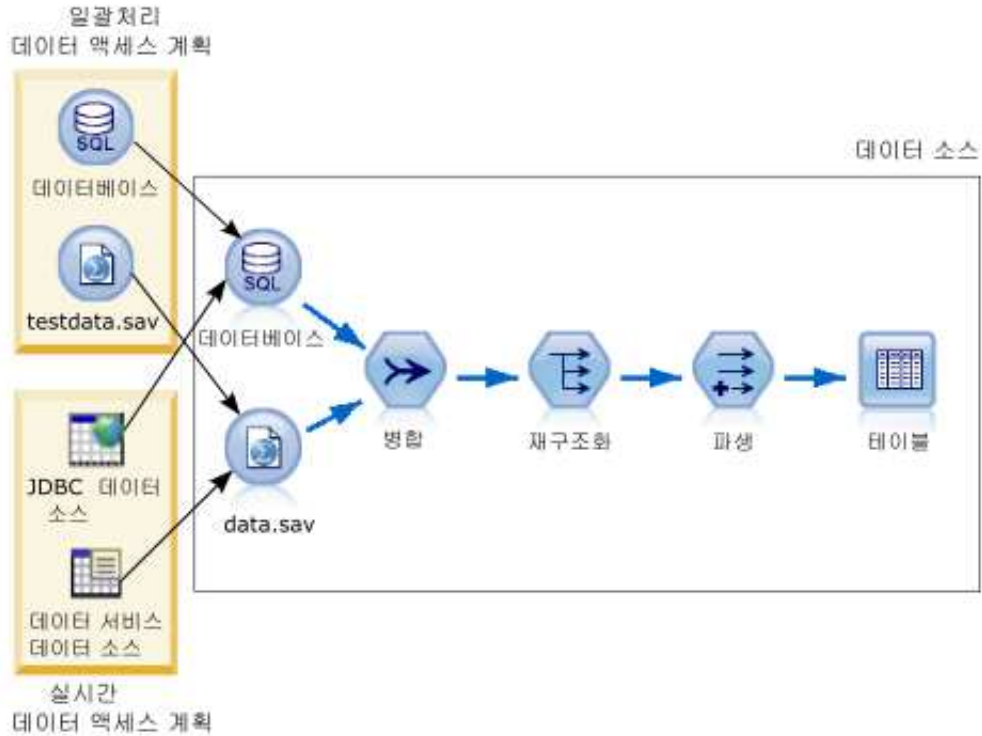
그림 3. 데이터 소스에 대한 데이터 액세스 계획
