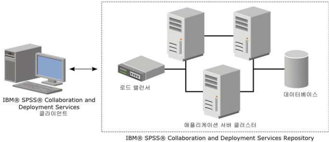
그림 5. 클러스터 아키텍처
