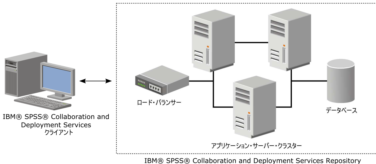
図 5. クラスター・アーキテクチャー
