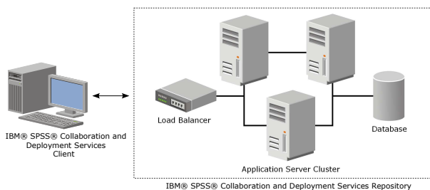
Figure 2. Architecture de déploiement groupée
