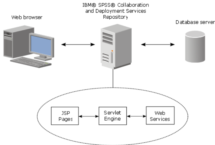
Abbildung 1. JSP-Architektur
