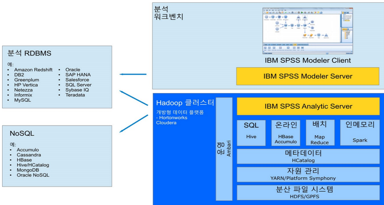
그림 1. 아키텍처
