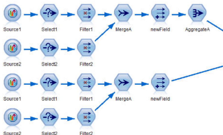
Figura 49. Ejemplo de secuencia
