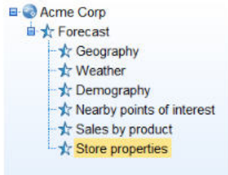
图 52. 子流示例
