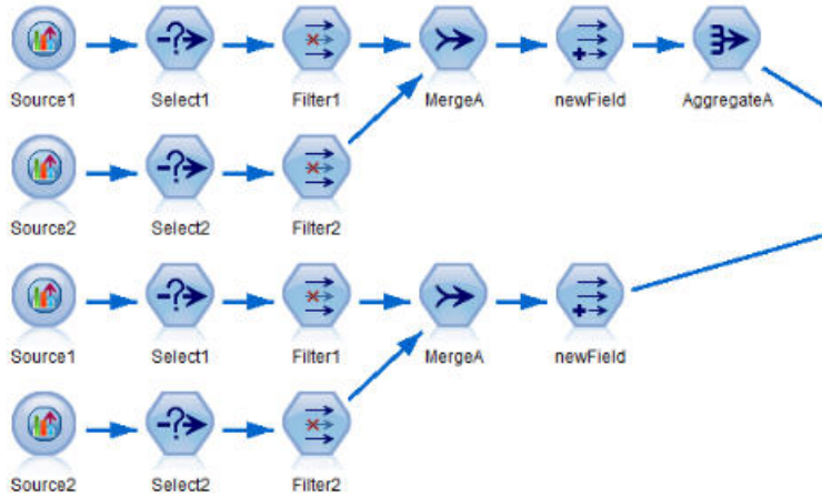
图 49. 示例流
