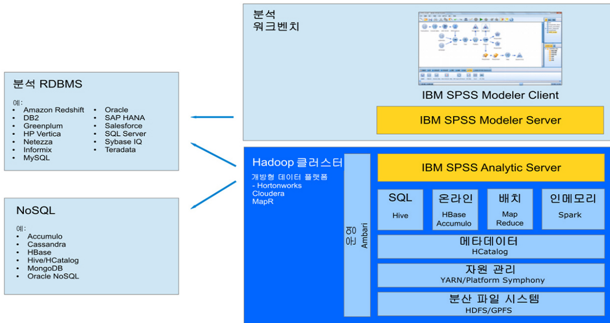
그림 1. 아키텍처
