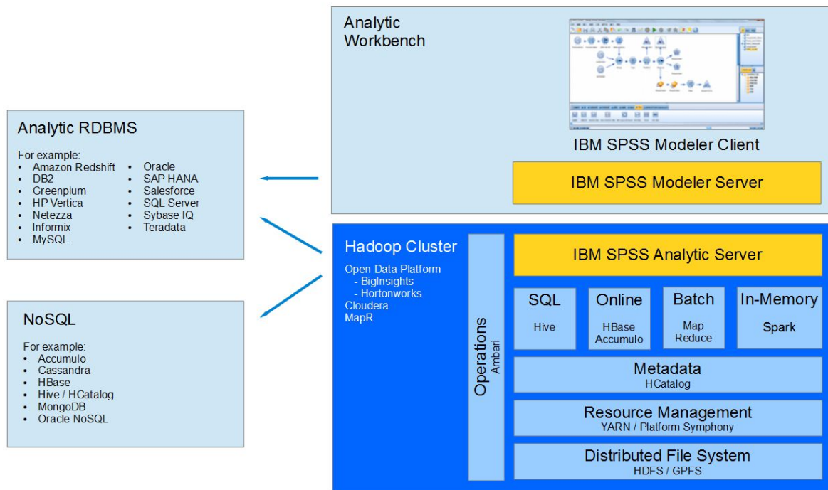
Figura 1. Arquitectura
