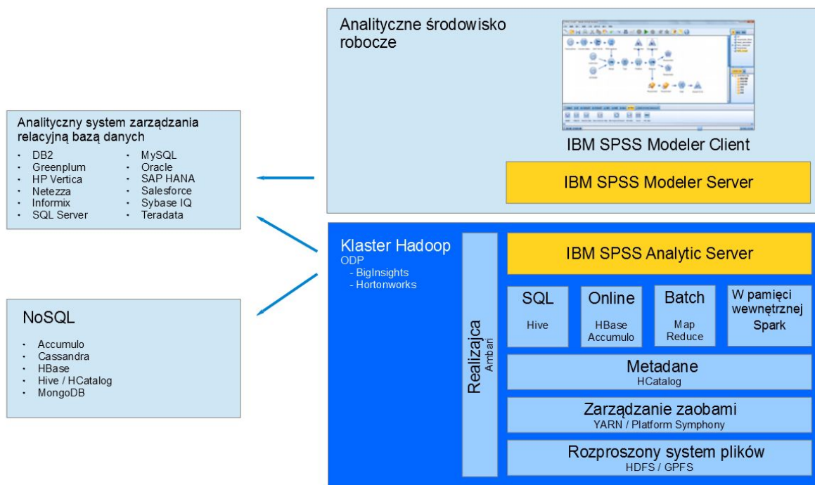
Rysunek 1. Architektura
