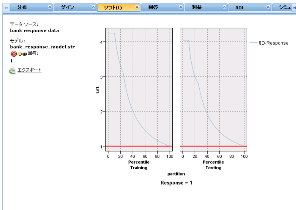
図 6-4 リフト グラフ
