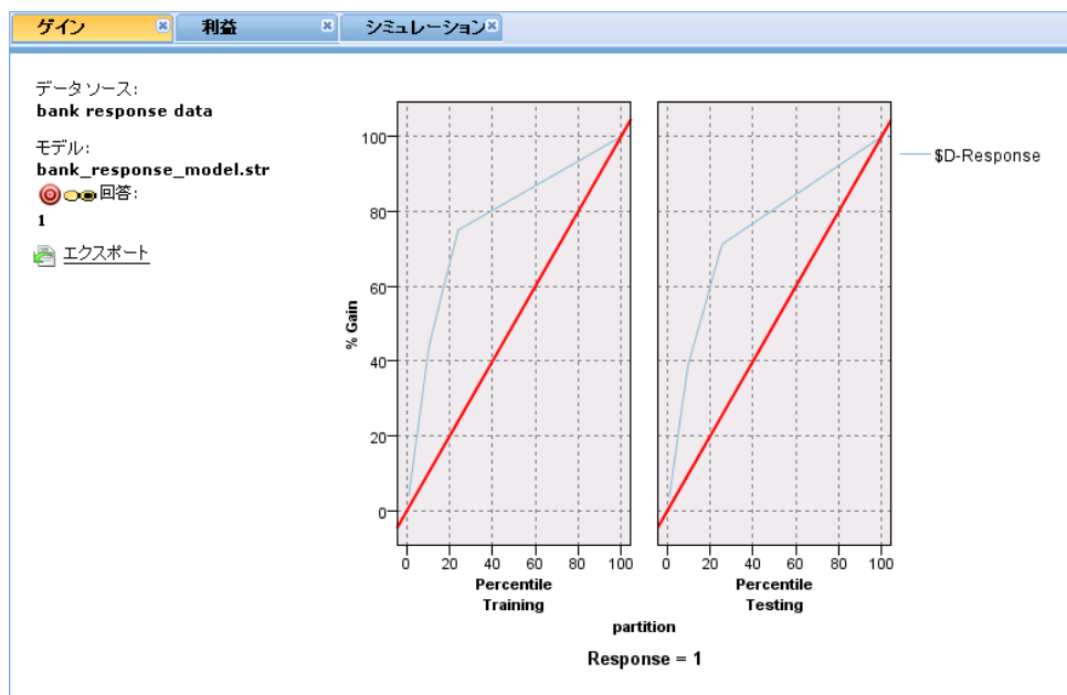
図 6-3 ゲイン グラフ
