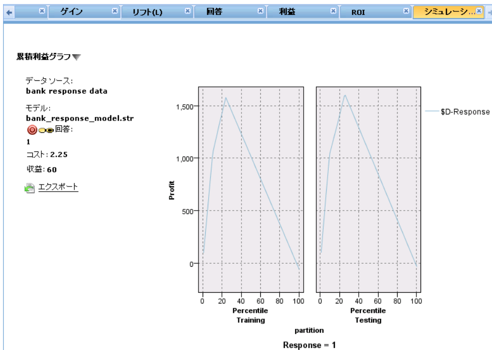
図 6-9 累積利益グラフ
