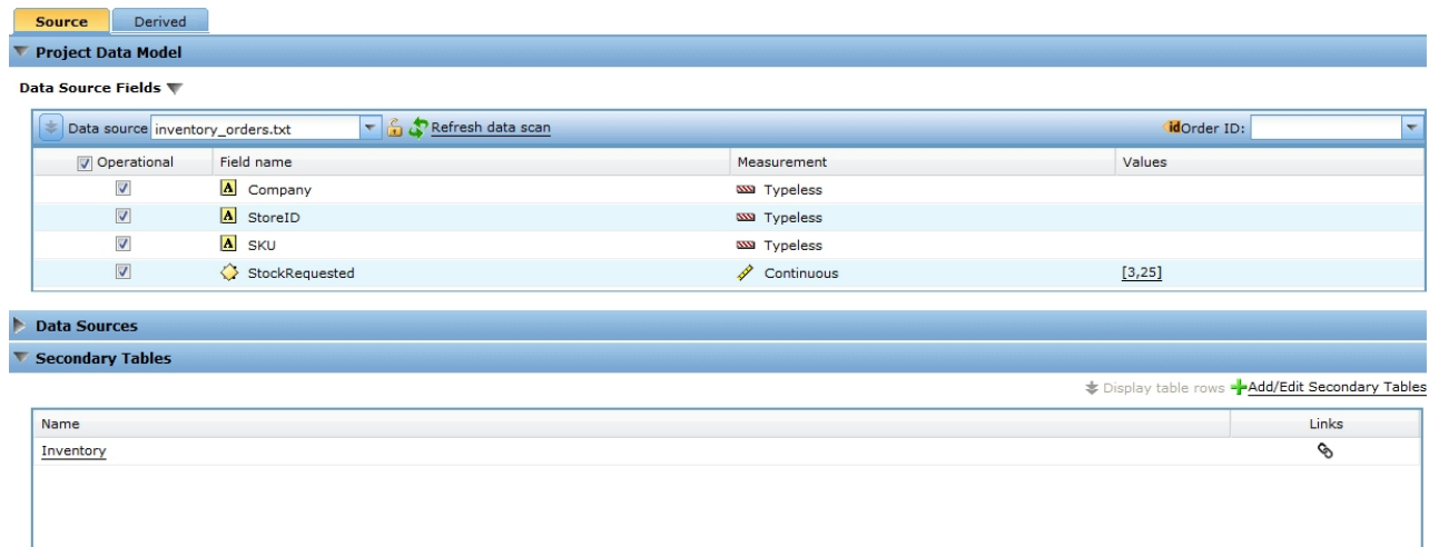
Figura 3. Data tab
