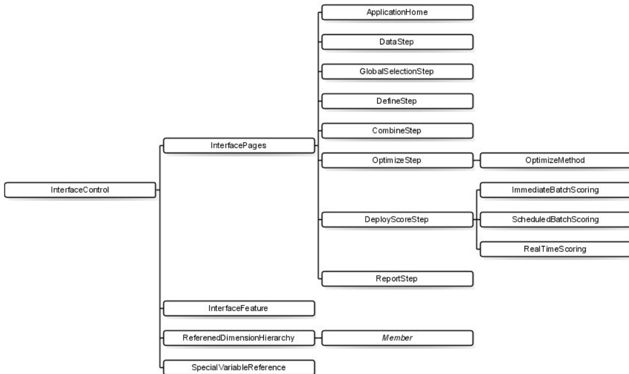
Figura 2. Elemento InterfaceControl
