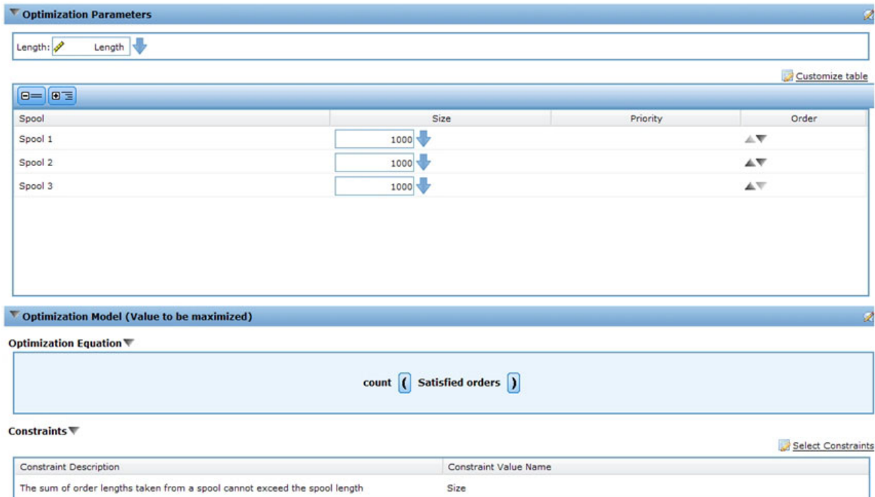
Figura 12. Guia Otimização
