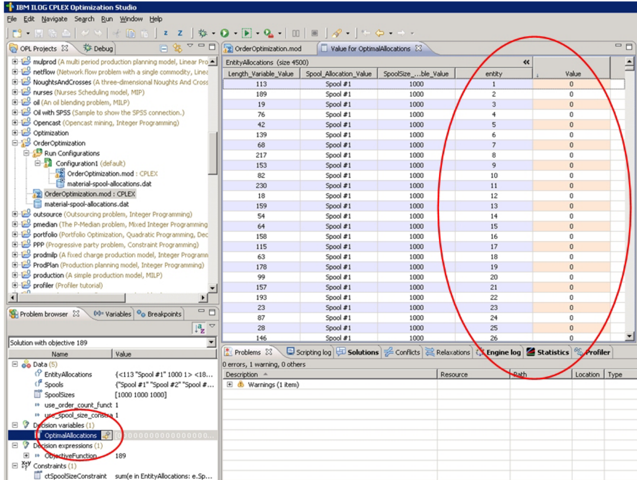
図 15. 「値」列
