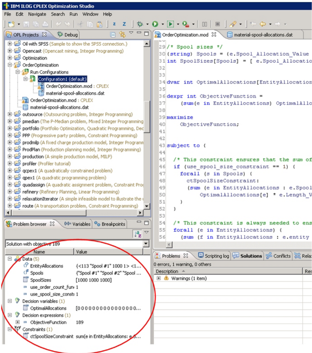
図 14. Configuration1 の実行
