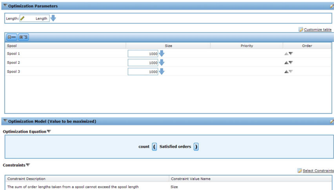
図 12. 「最適化」タブ
