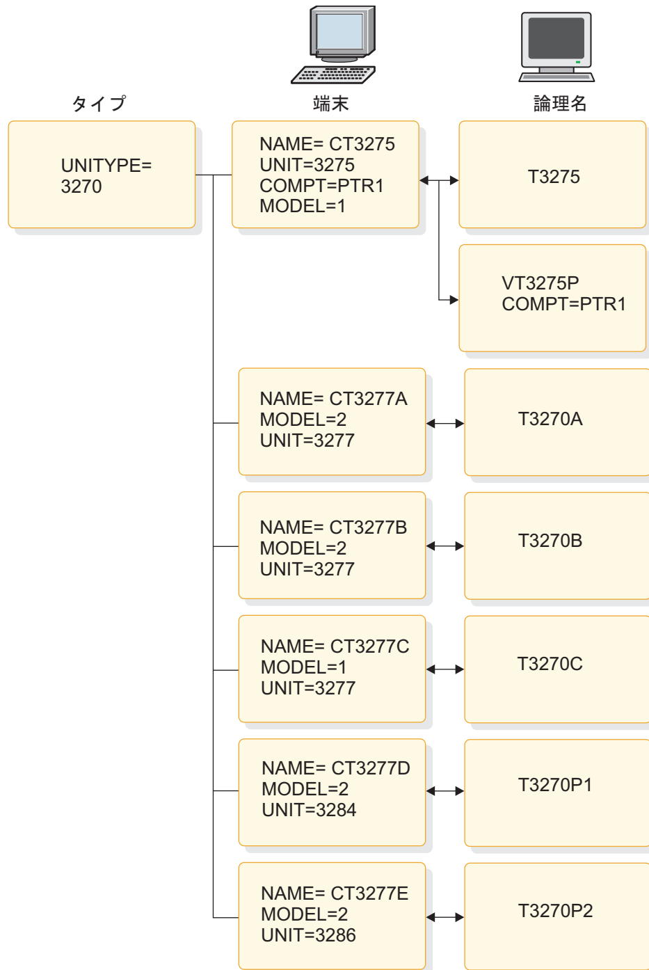
図 8. 3270 VTAM 端末の構成
