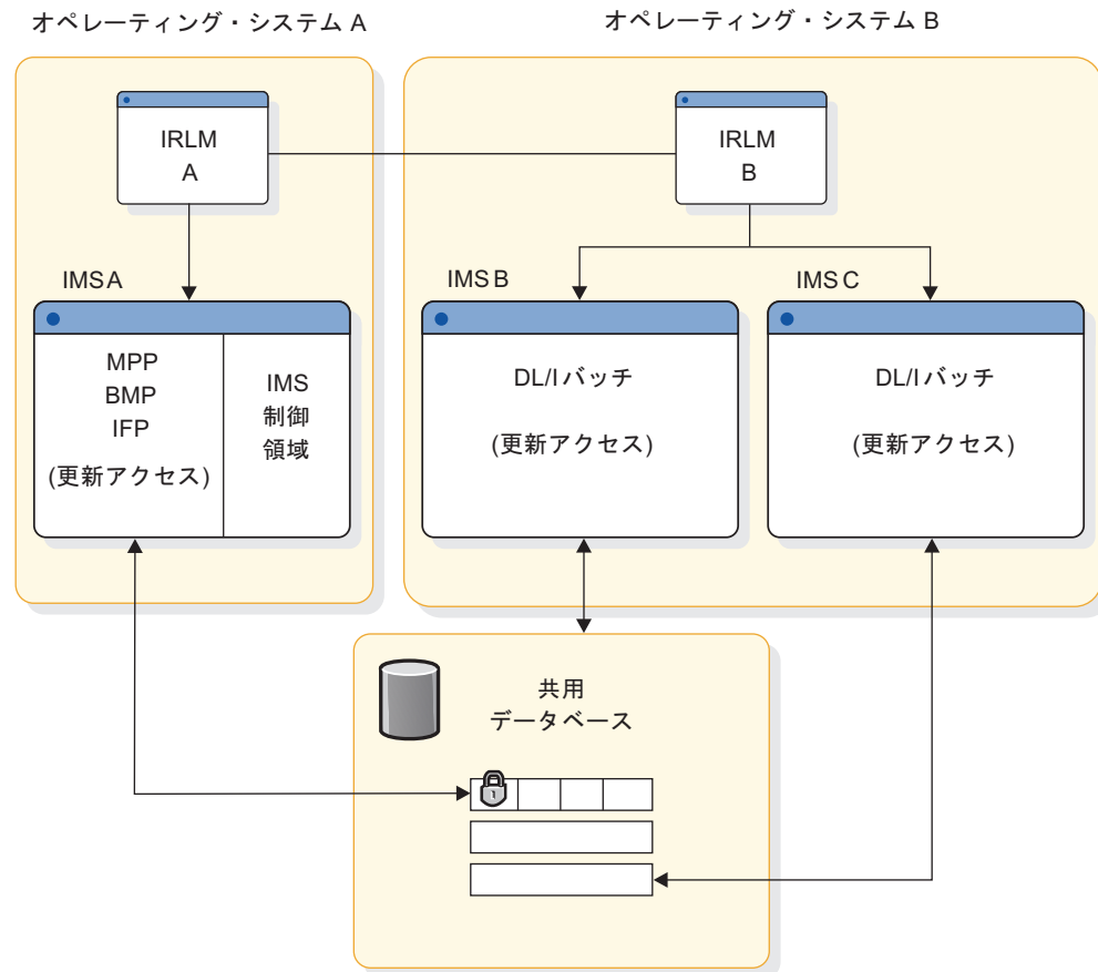
図 42. CPC 間ブロック・レベル・データ共有
