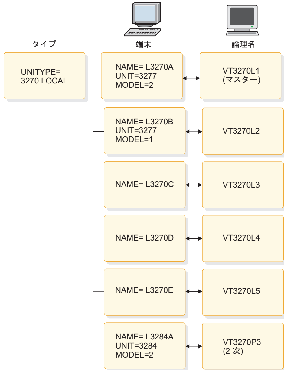
図 9. マスター端末の構成
