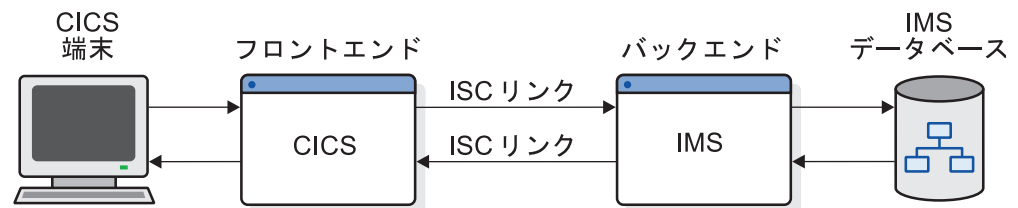
図 57. CICS からの呼び出される既存または新規のIMS トランザクション
