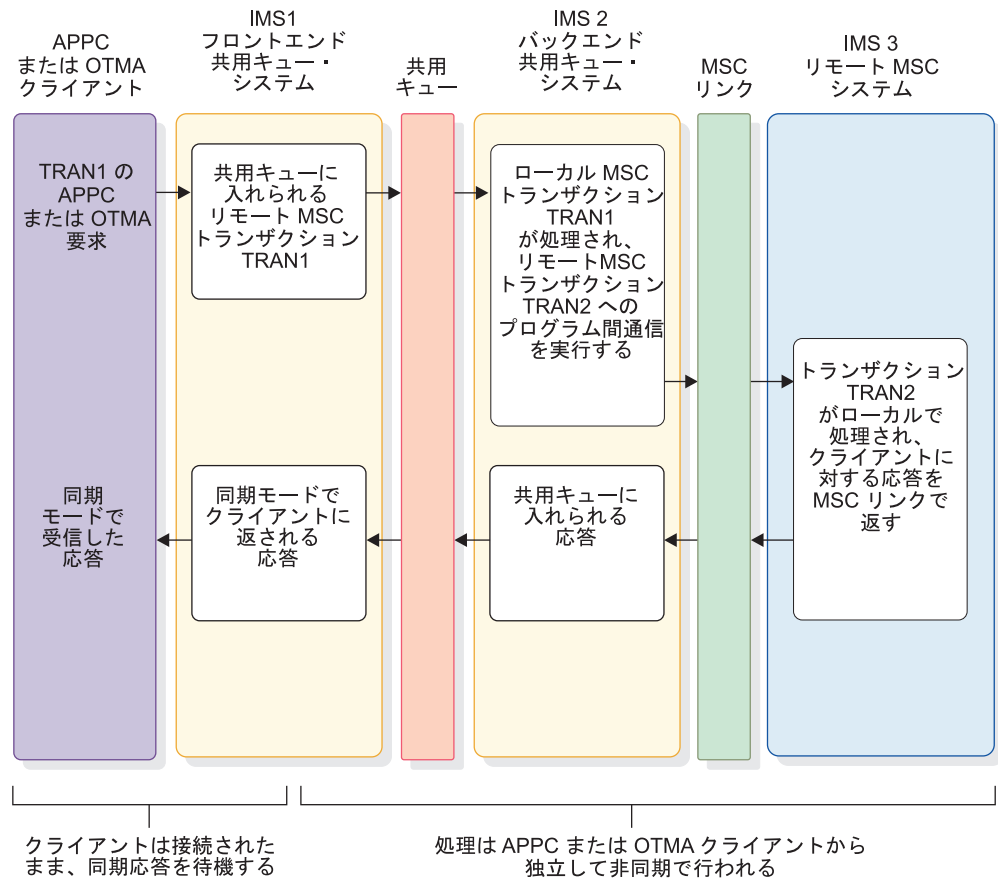
図 127. 1 つのプログラム間通信を伴う、MSC と共用キューを使用して経路指定される APPC または OTMA トランザクション
