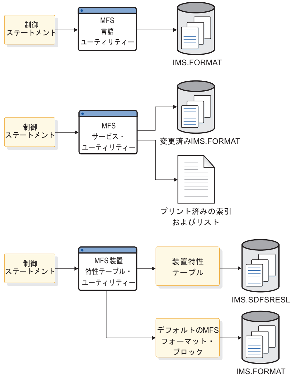
図 51. MFS ユーティリティとその出力
