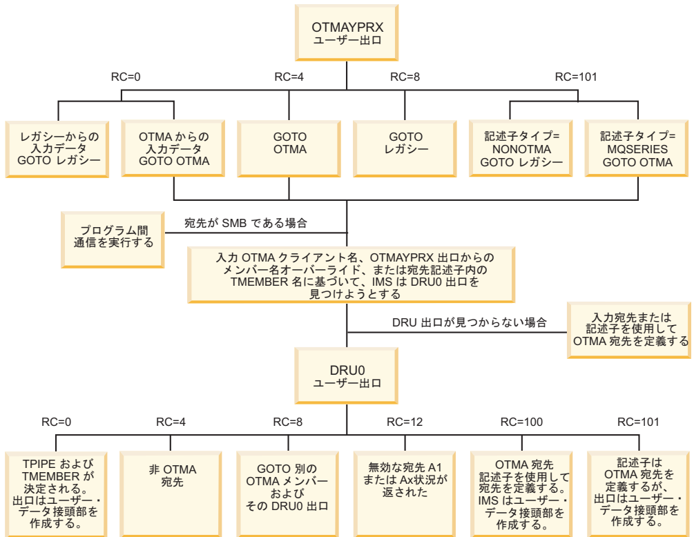
図 139. OTMAYPRX OTMA ユーザー出口および DFSYDRU0 OTMA ユーザー出口のメッセージ宛先の決定方法
