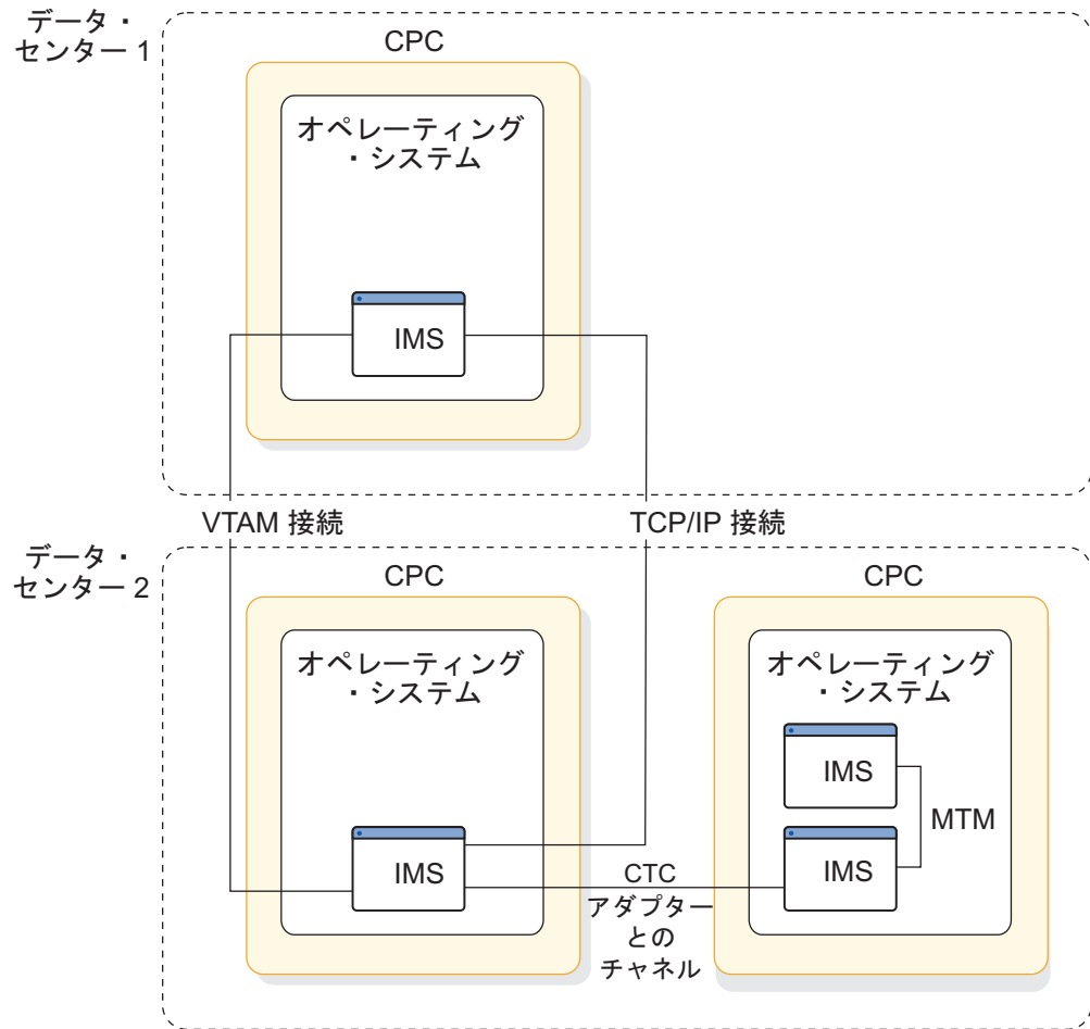
図 112. MSC 物理リンク・タイプ
