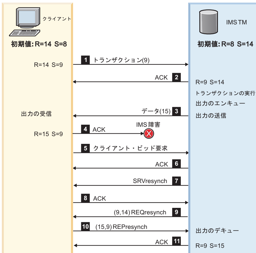
図 155. OTMA 再同期メッセージ・フローのサンプル
