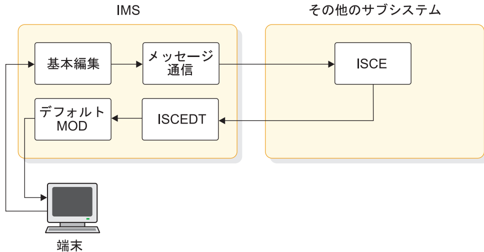
図 63. IMS とその他のサブシステム間のメッセージ通信経路指定の ISC 例
