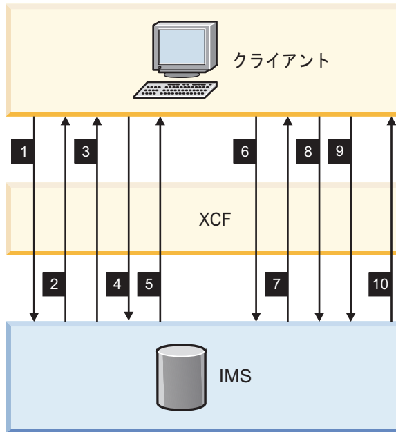
図 146. コミット後送信フローに対するメッセージ・フローのサンプル
