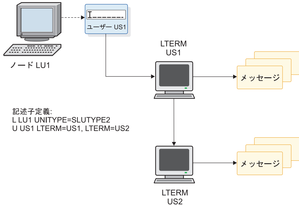
図 13. ETO 動的リソース
