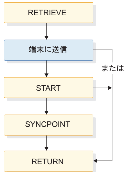
図 89. IMS から CICS への RETRIEVE を使用したアプリケーション・プログラムのフロー
