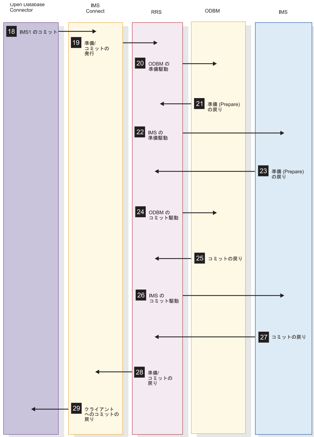
図 38. IMS Universal ドライバーに関する分散 1 フェーズ・コミット・グローバル・トランザクション・クライアントのフロー (2/2)
