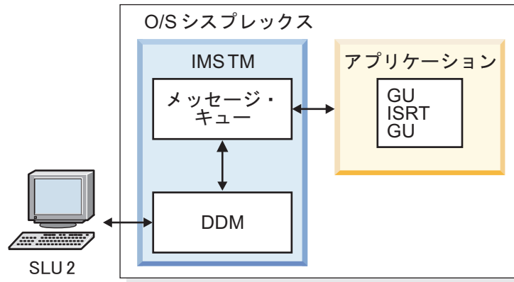
図 132. 標準 SLU 2 トランザクション・フロー
