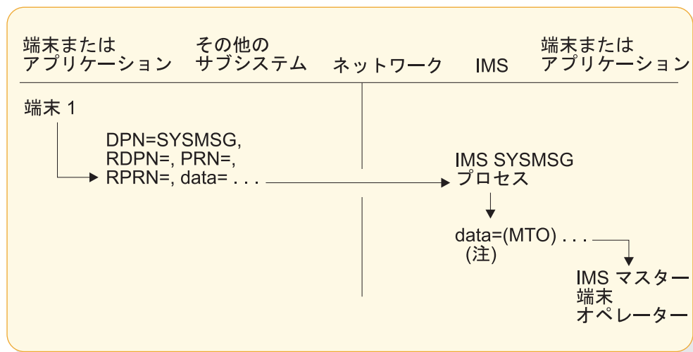
図 75. 他のサブシステム端末から IMS A への PRN のない SYSMMSG の例
