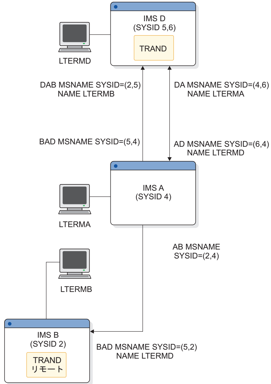
図 120. リモート LTERM
