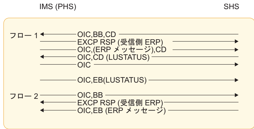
図 109. MULT1 として定義された IMS コンポーネントの受信側 ERP の例
