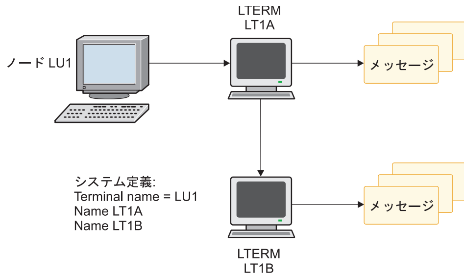
図 12. 静的リソース
