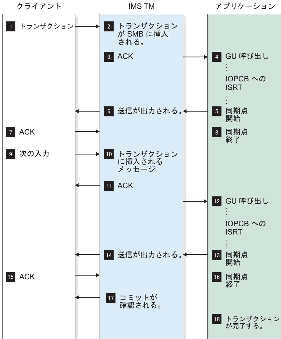
図 27. 送信後コミット、同期レベル = CONFIRM の場合の OTMA 会話型プロトコルのフロー
