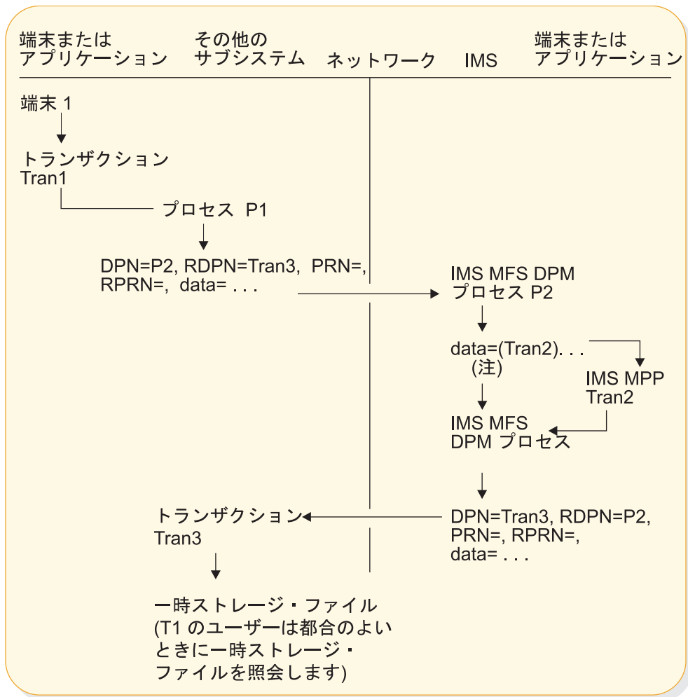
図 79. IMS MPP が他のサブシステム端末からアクセスされ、他のサブシステムの一時記憶域ファイルへの応答が返される例
