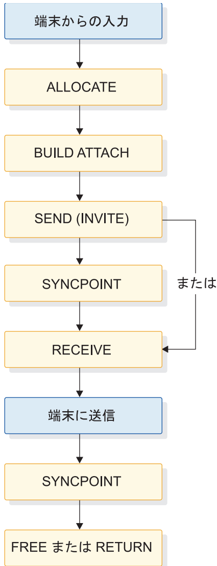
図 85. SEND/RECEIVE を使用した CICS から IMS へのアプリケーション・プログラムのフロー
