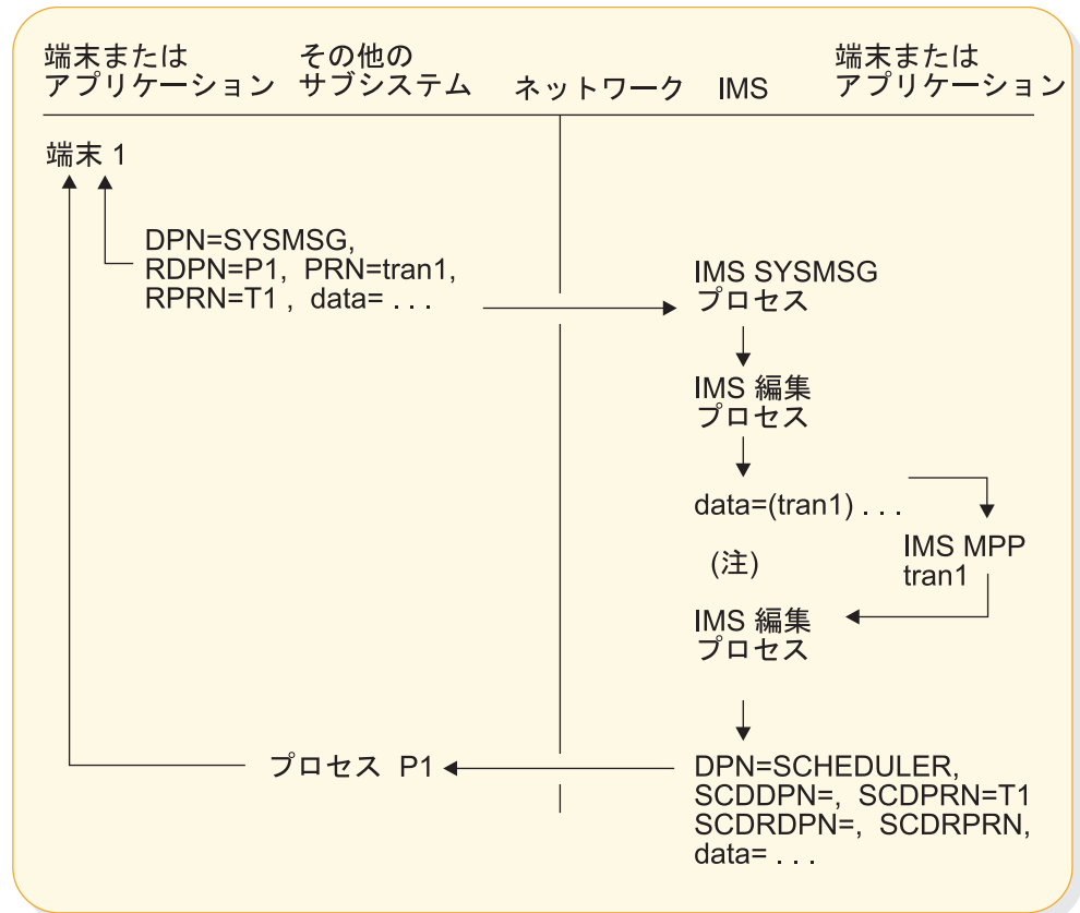
図 76. 別のサブシステム端末から IMS への PRN 付きの SYMSMSG の例
