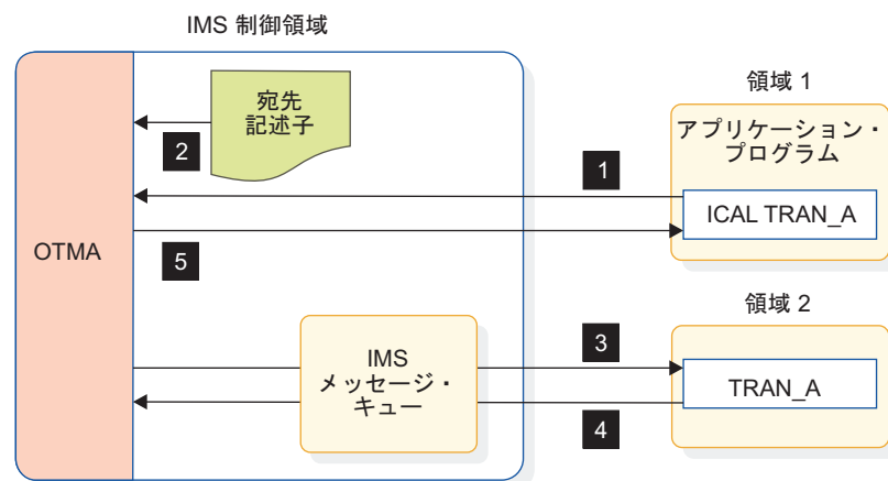
図 156. IMS 同期プログラム間通信処理
