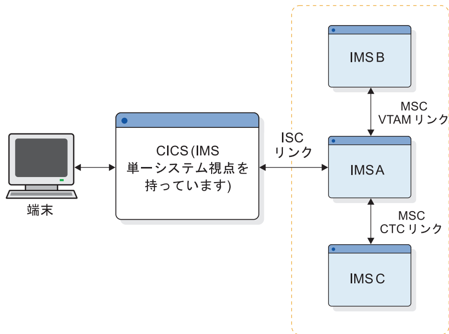
図 60. ISC を使用して CICS から IMS MSC へ
