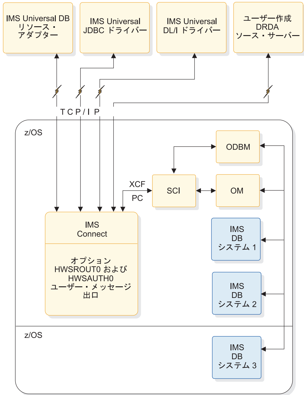
図 20. IMS DB システムのための IMS Connect サポートの概要
