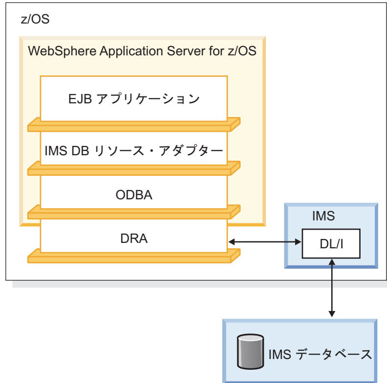
図 6. IMS DB リソース・アダプターを使用する WebSphere Application Server for z/OS EJB アプリケーション
