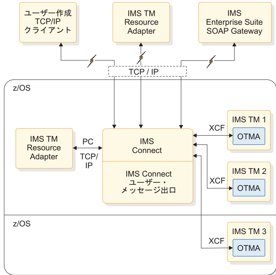
図 21. IMS TM システムのための IMS Connect サポートの概要
