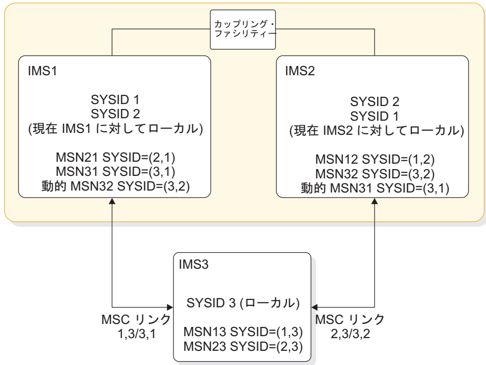
図 123. 共用キューを使用する IMSplex と共存する MSC ネットワーク
