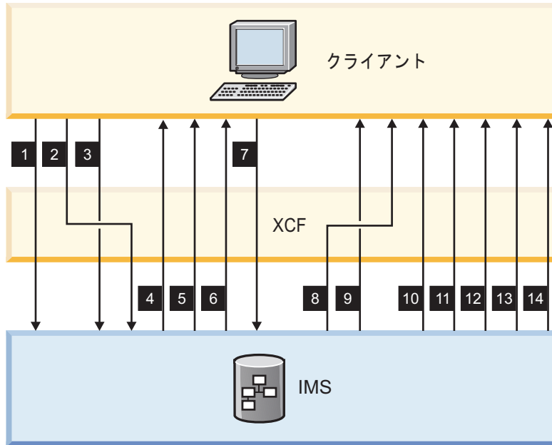
図 148. 送信後コミット・フローに対するサンプル・メッセージ・フロー
