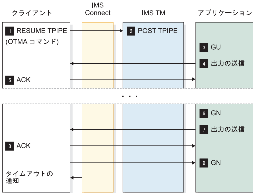
図 33. コミット後送信、非同期出力受信 (クライアントは出力を待機) のフロー
