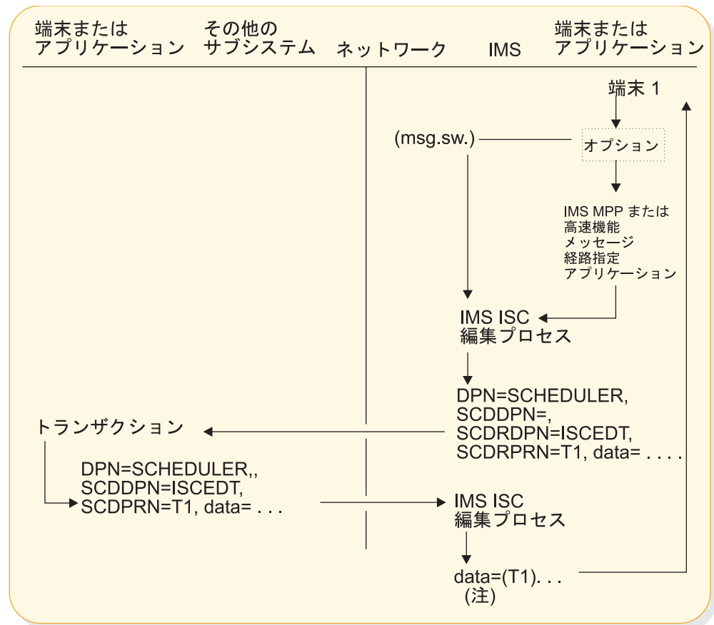
図 74. ISC 編集でのメッセージ経路指定の例
