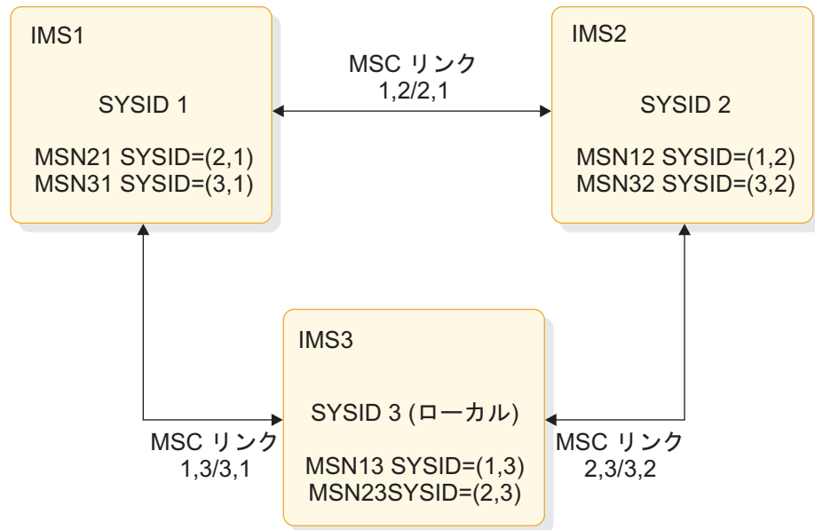
図 122. IMSplex を持たない MSC ネットワーク
