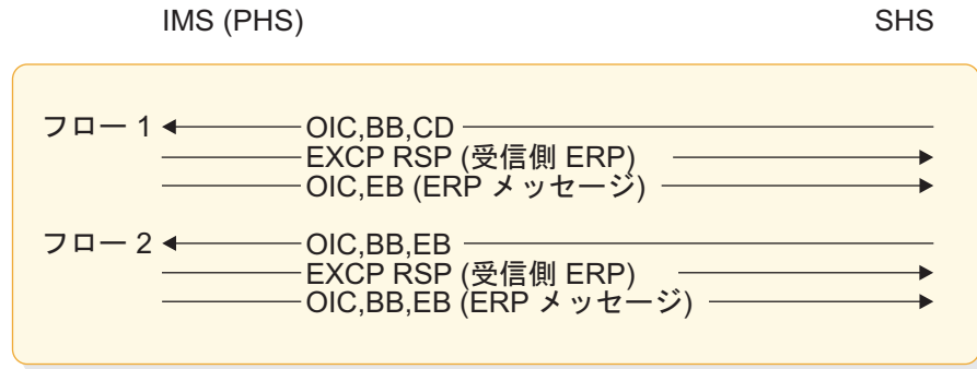
図 107. SINGLET1 として定義された IMS コンポーネントの受信側 ERP の例
