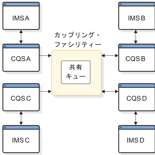
図 44. 基本的な共有キュー環境
