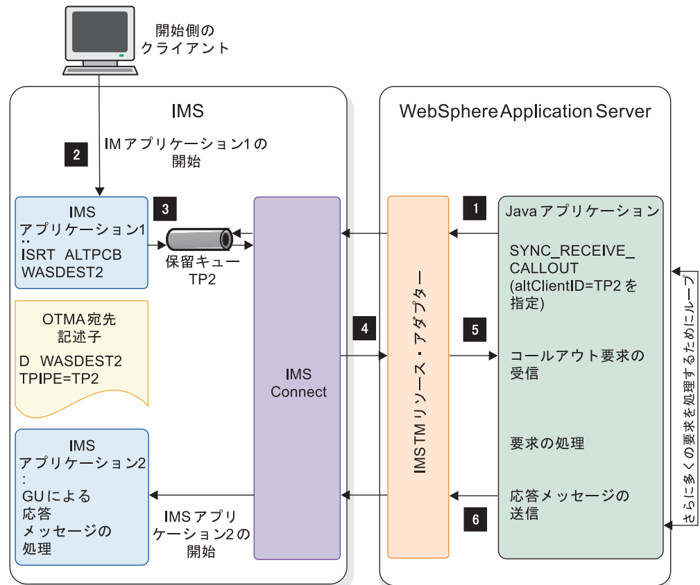
図 120. 非同期コールアウト・メッセージ・フロー
