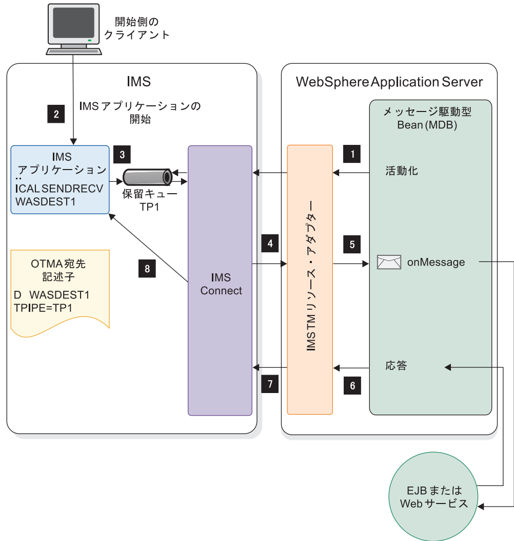
図 121. メッセージ駆動型 Bean を使用した IMS からの同期コールアウト・メッセージの処理
