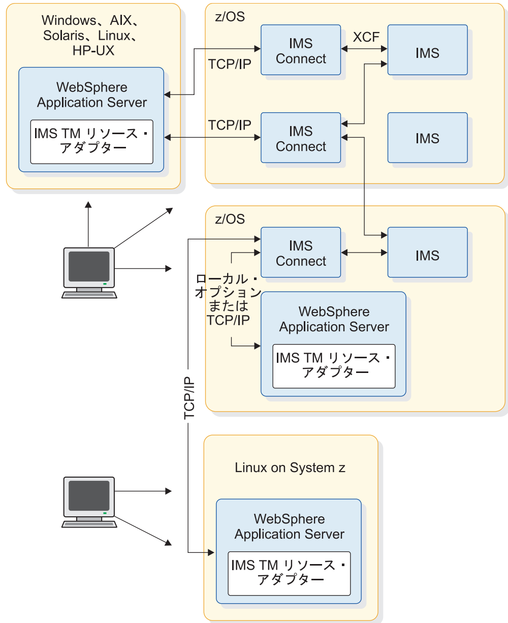
図 114. IMS TM リソース・アダプターの接続
