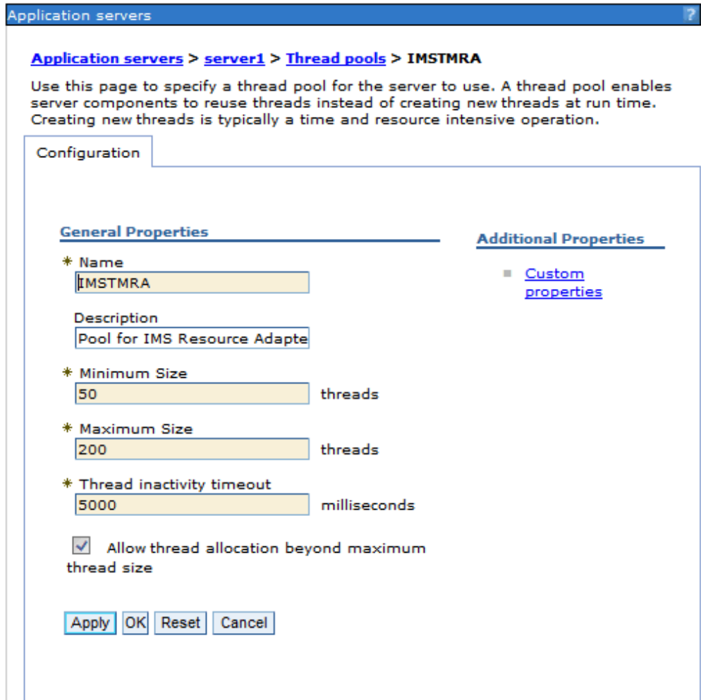
図 126. WebSphere Application Server でのスレッド・プール構成
