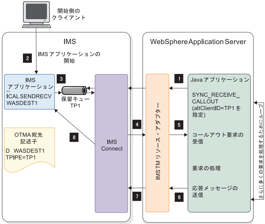
図 119. 同期コールアウト・メッセージ・フロー
