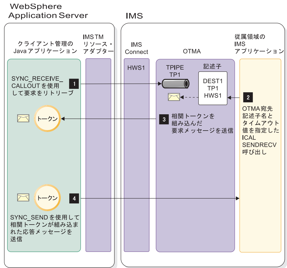
図 128. 非 MDB Java アプリケーションでの IMS からの同期コールアウト要求のリトリートとその要求に対する応答のプロセス・フロー
