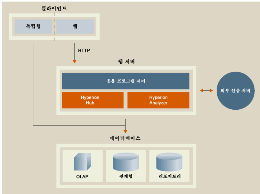
그림 1: HyperionAnalyzer 아키텍처
