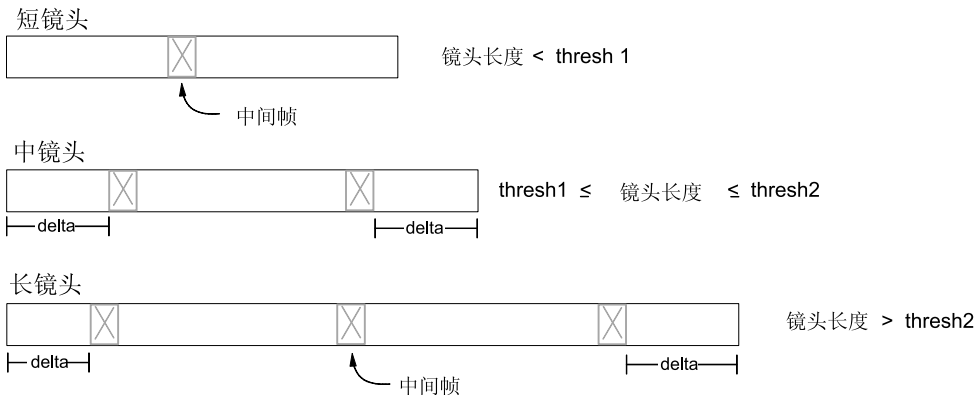
图 29. 如何使用 DBvStoryboardCtrl 结构中的值
