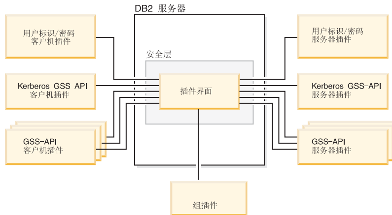
图 6. 在 DB2 服务器上部署安全插件
