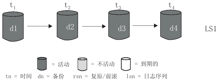
图 12. 活动数据库备份. num_db_backups 的值已设置为 4。
