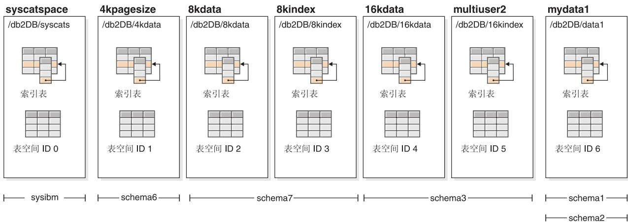
图 27. 传输后的 TARGETDB 数据库
