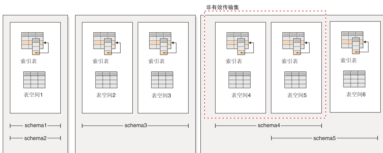
图 24. 表空间和模式集
