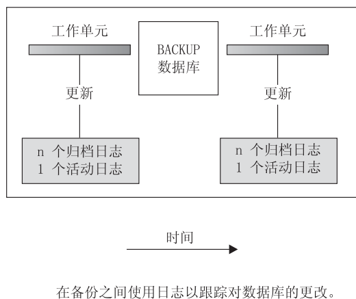
图 2. 前滚恢复中活动的和已归档的数据库日志。在运行时间较长的事务中，可以有多个活动日志。
