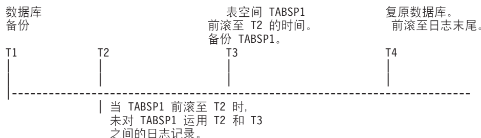
图 28. 表空间备份要求
