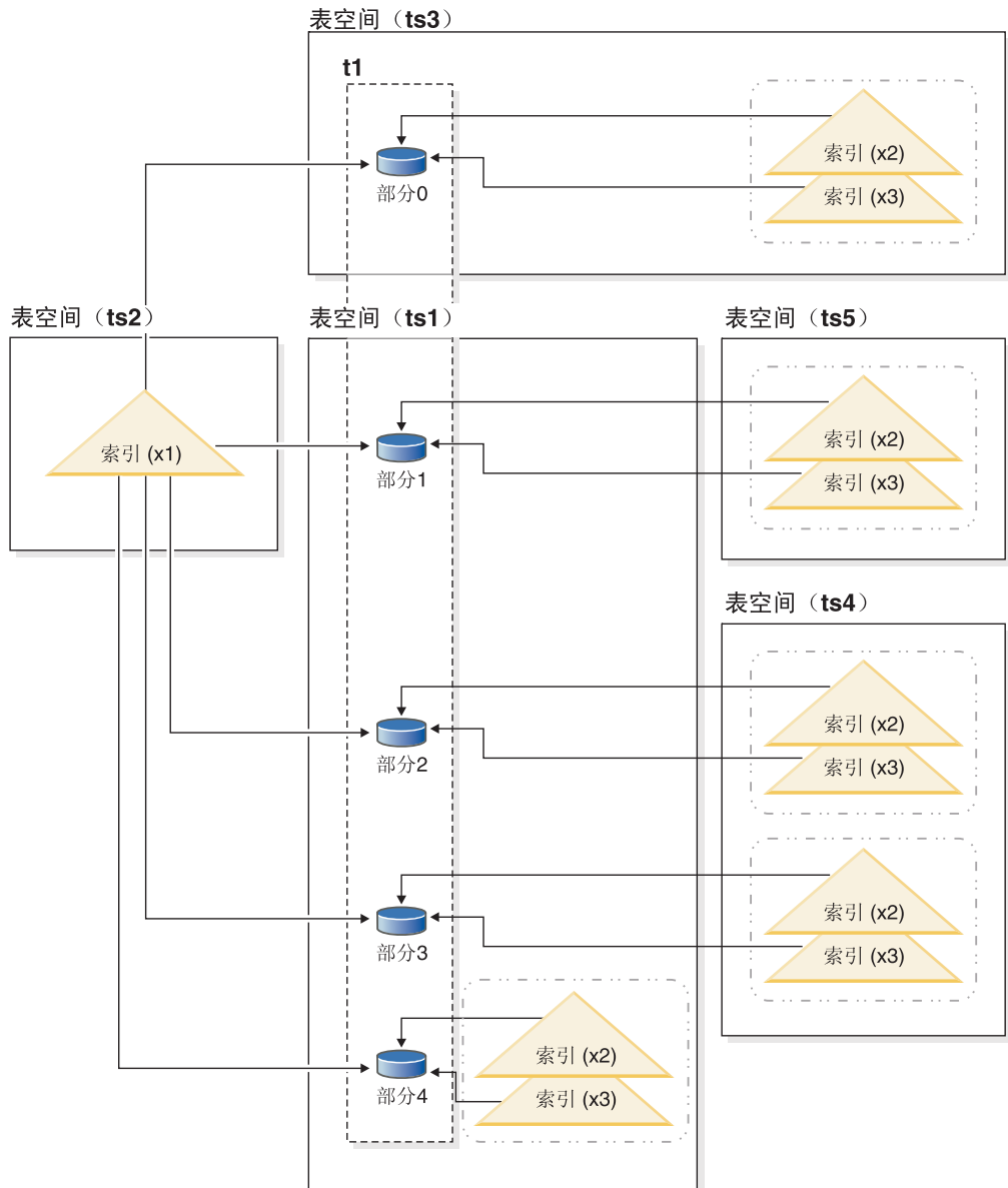
图 52. 分区表的分区索引和非分区索引
