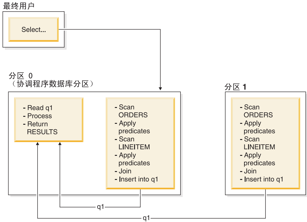
图 55. 并置连接示例
