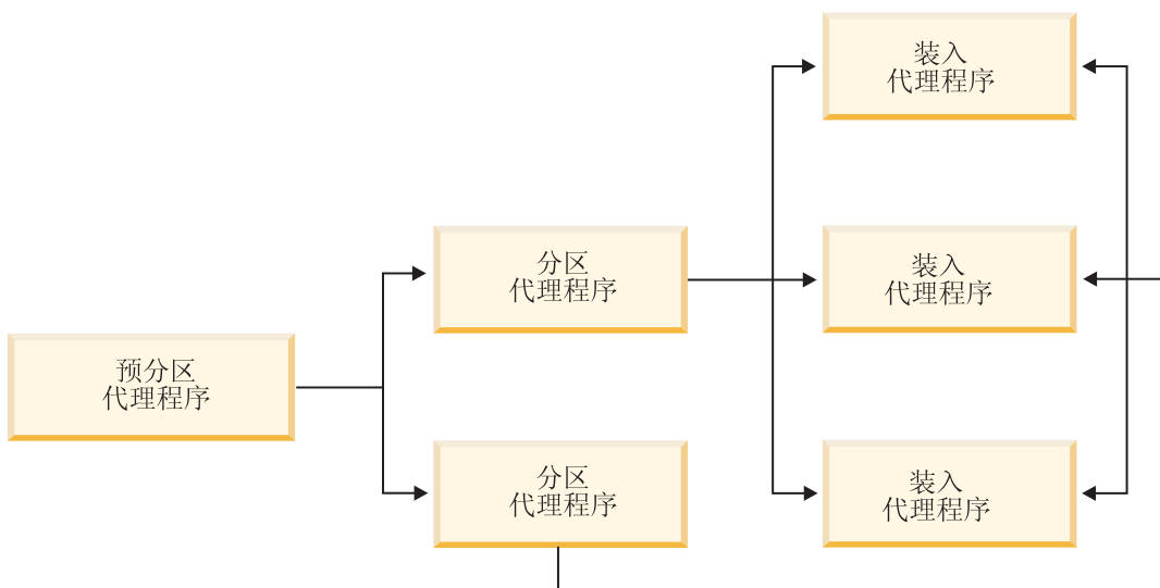
图 41. 分区数据库 load 概述。预分区代理程序读取源数据，然后向两个分区代理程序中的每个分区代理程序各发送接近一半的数据，这两个分区代理程序分布数据并将该数据发送给三个数据库分区中的一个数据库分区。每个数据库分区上的装入代理程序装入数据。
