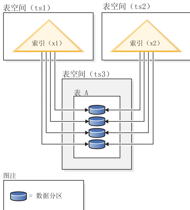
图 50. 分区表的非分区索引
