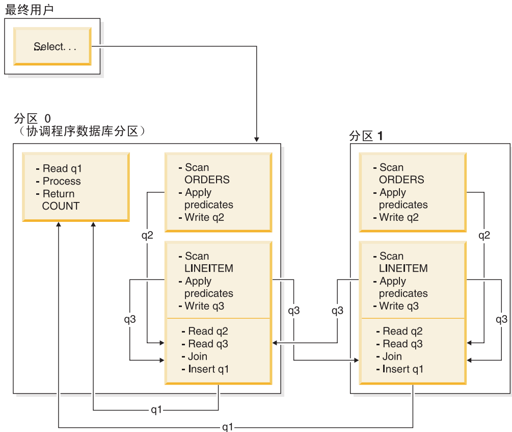
LINEITEM 表被发送到所有包含 ORDERS 表的数据库分区。表队列 q3 被广播至外表的所有数据库分区。 图 59. 广播内表连接示例
