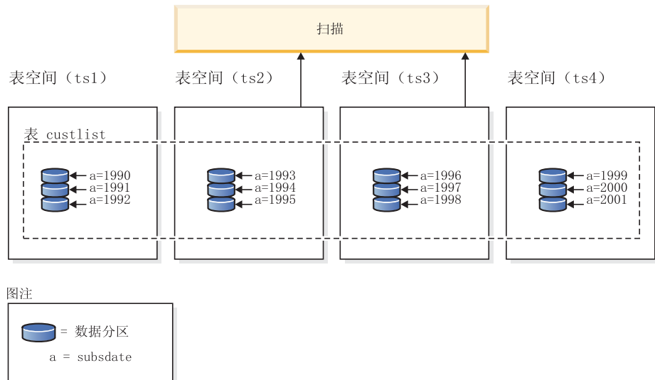
图 48. 数据分区消除功能在性能方面的好处
