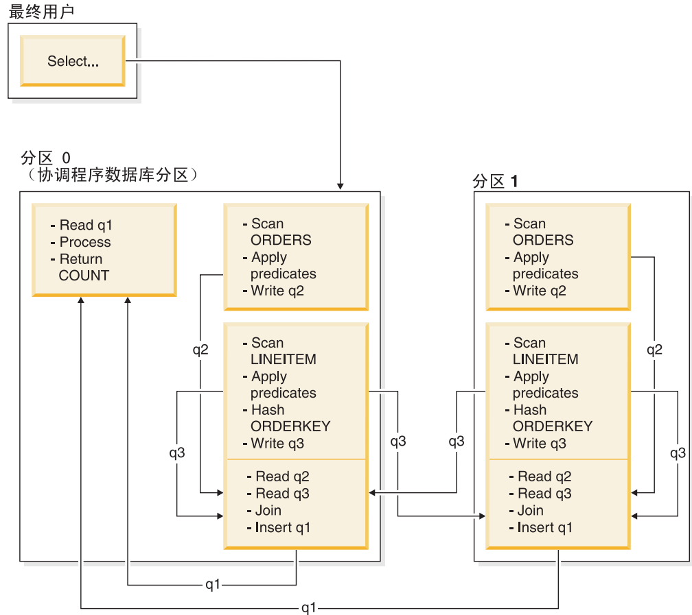
ORDERS 表根据 ORDERKEY 列进行分区。LINEITEM 表根据另一个列进行分区。LINEITEM 表将进行散列并被发送到 ORDERS 表的正确数据库分区。在此示例中，假定连接谓词为： orders.orderkey = lineitem.orderkey 。 图 60. 定向内表连接示例
