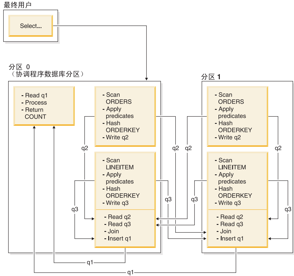
图 58. 定向内表和外表连接示例
