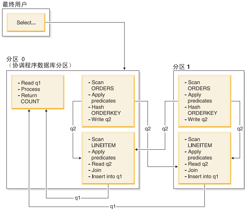
LINEITEM 表根据 ORDERKEY 列进行分区。ORDERS 表根据另一个列进行分区。ORDERS 表将进行散列并被发送到 LINEITEM 表的正确数据库分区。在此示例中，假定连接谓词为： orders.orderkey = lineitem.orderkey. 图 57. 定向外表连接示例
