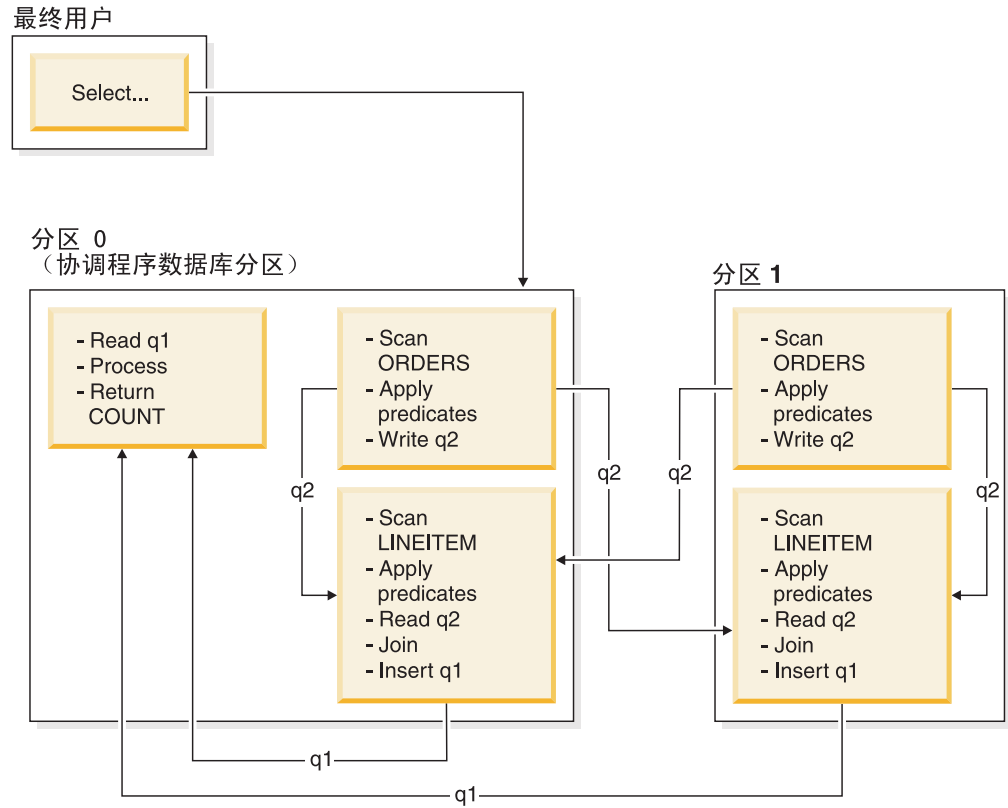
图 56. 广播外表连接示例
