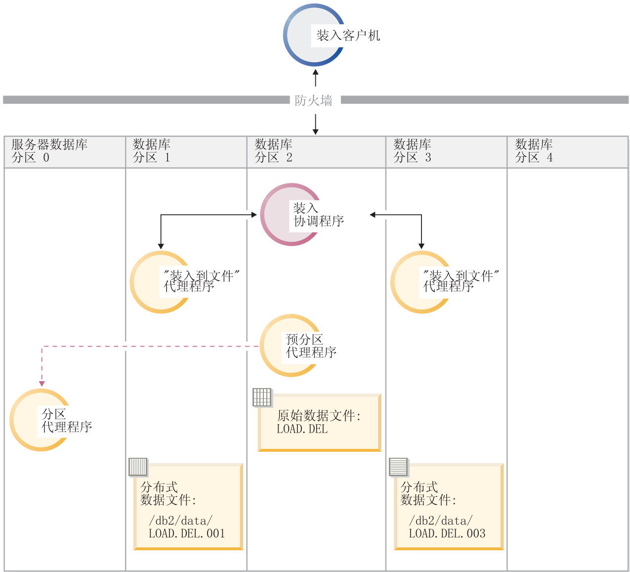
图 43. 使用一个分区代理程序将数据装入到数据库分区 1 和 3 中。此图说明发出以上命令后产生的行为。将使用数据库分区 0 上运行的 1 个分区代理程序将数据装入到数据库分区 1 和 3 中。
