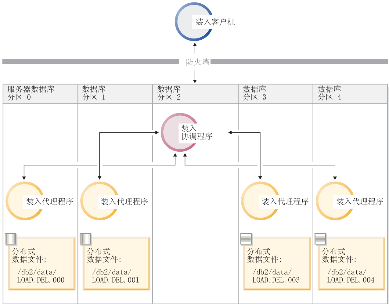
图 44. 将数据装入到其中定义了特定表的所有数据库分区中。此图说明发出以上命令后产生的行为。将分布式数据装入到所有用来定义 TABLE1 的数据库分区中。
