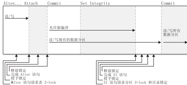
图 38. 此图演示 ATTACH 操作期间数据可用性的各个阶段。
