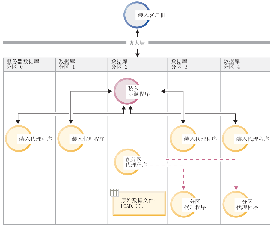
图 42. 将数据装入到数据库分区 3 和 4 中。此图说明发出以上命令后产生的行为。数据将装入到数据库分区 3 和 4 中。
