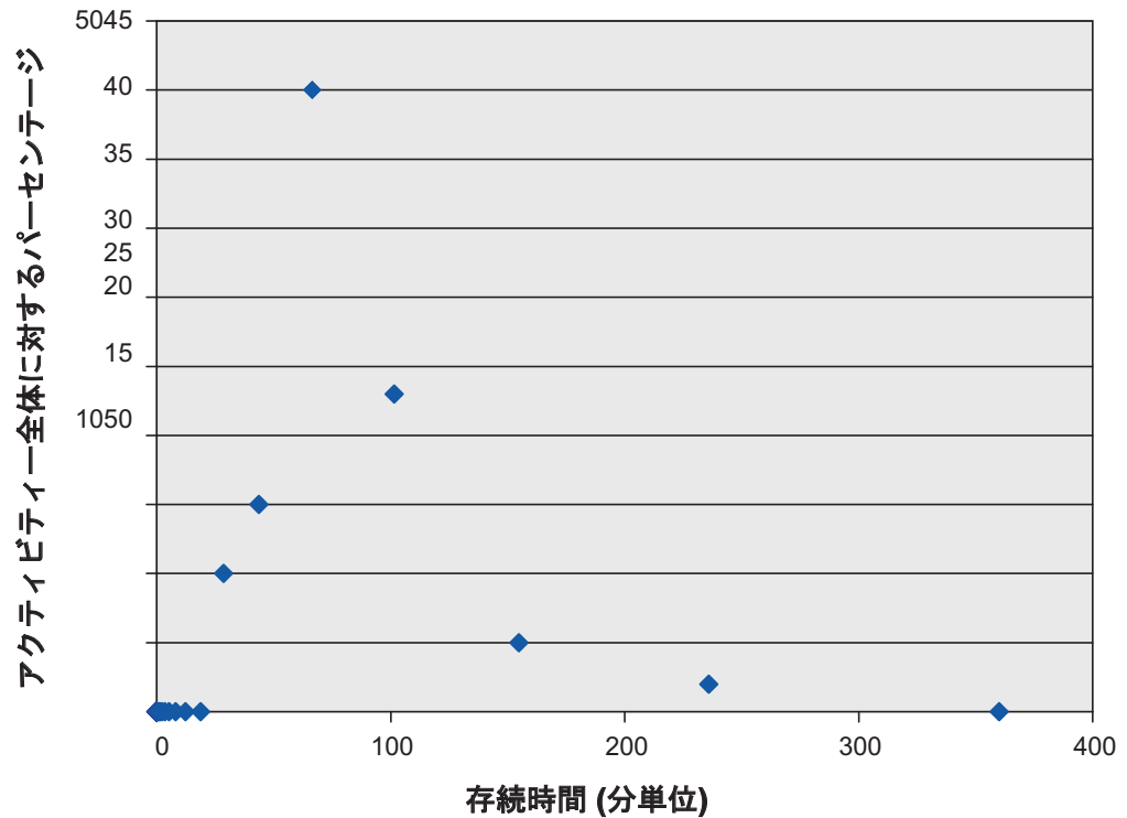
図 32. 未分類アクティビティのアクティビティ持続期間ヒストグラム
