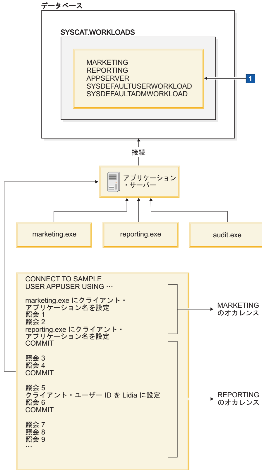
図 7. 3 層環境におけるワークロードの割り当ての例
