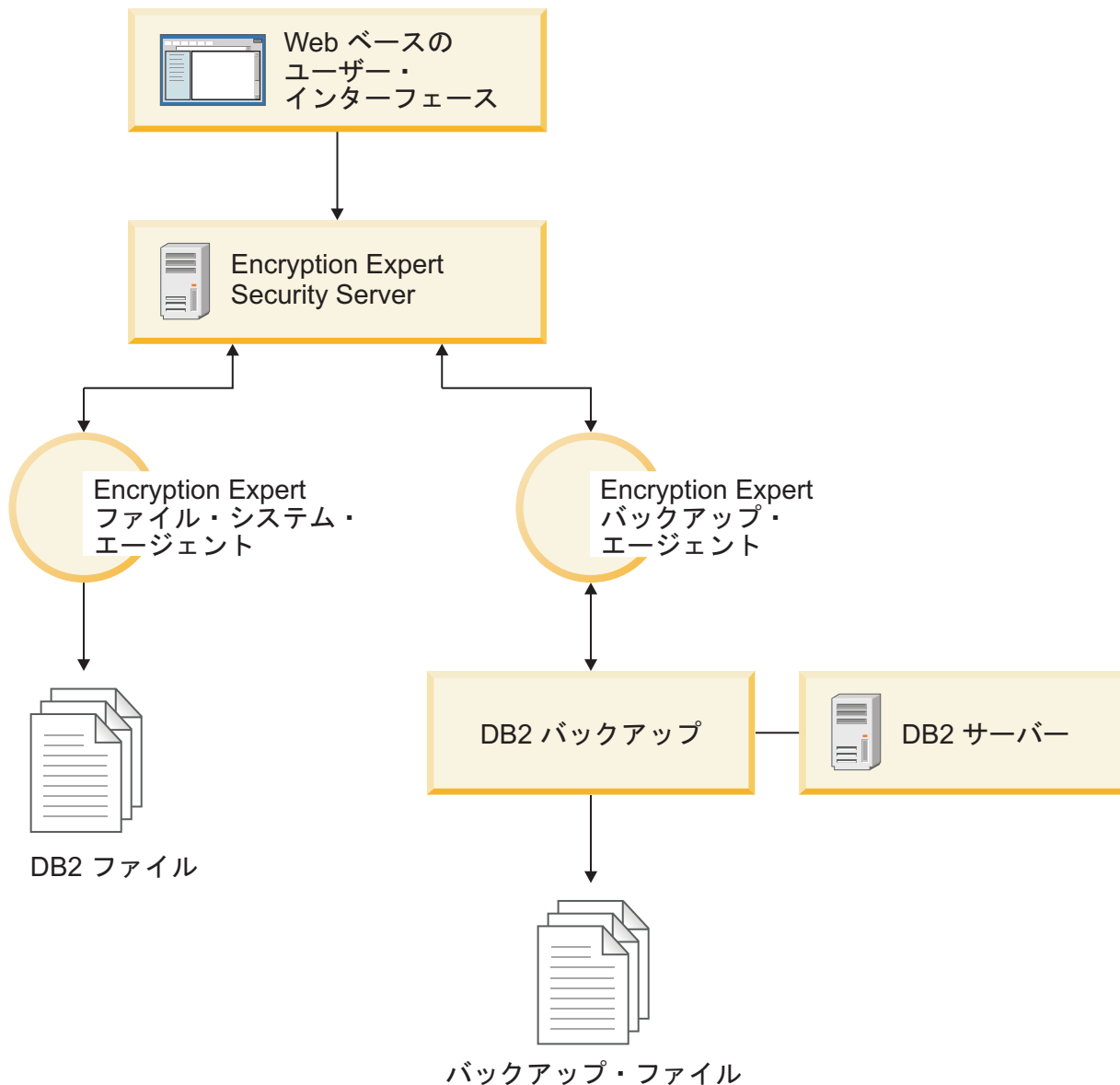
図4. Database Encryption Expert のアーキテクチャー
